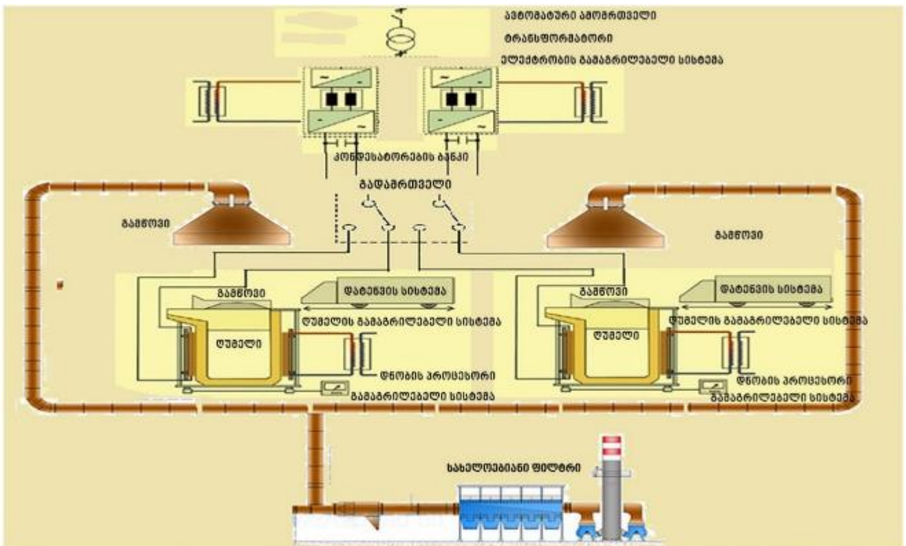
სურათი 4.2.2.2.1. ინდუქციური ღუმელის სქემა
