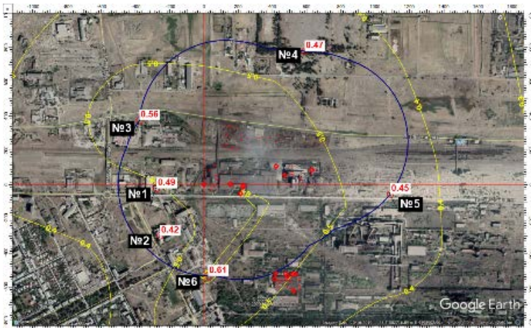
ნივთიერება: 6204 აზოტის დიოქსიდი, გოგირდის დიოქსიდი. მაქსიმალური კონცენტრაციები უახლოეს საცხოვრებელ სახლთან (წერტ. №1,2) და ნორმირებულ 500 მ. ზონის საზღვართან (წერტ.3,4,5,6).
