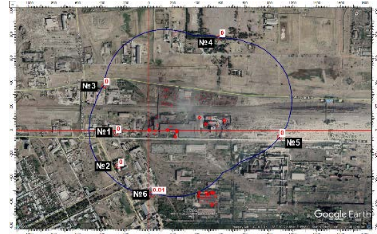
წივთიერება: 0328 ნახშირბადი (ქვარტლი).მაქსიმალური კონცენტრაციები უახლოეს საცხოვრებელ სახლთან (წერტ. N1,2) და ნორმირებულ 500 მ. ზონის საზღვართან (წერტ.3,4,5,6).
