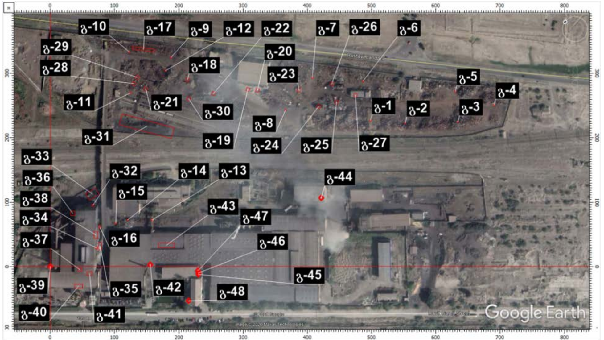
სურათი 6.3.2.1. საწარმოს სიტუაციური გეგმა მანვნი ნივთიერებათა გაფრქვევის წყაროების დატანით
