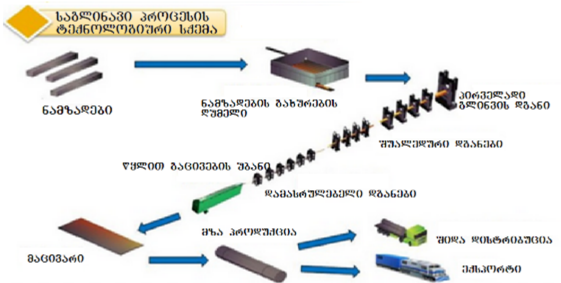
სქემა 4.2.2.4.1. გლინვის პროცესის ტექნოლოგიური სქემა
