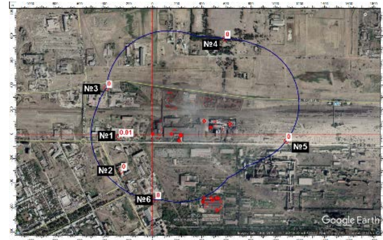
ნივთიერება: 6053 წყალბადის ფორიდი და ფორის სუსტად ხსნადი მარილები. მაქსიმალური კონცენტრაციები უახლოეს საცხოვრებელ სახლთან (წერტ. №1,2) და ნორმირებულ 500 მ. ზონის საზღვართან (წერტ.3,4,5,6).
