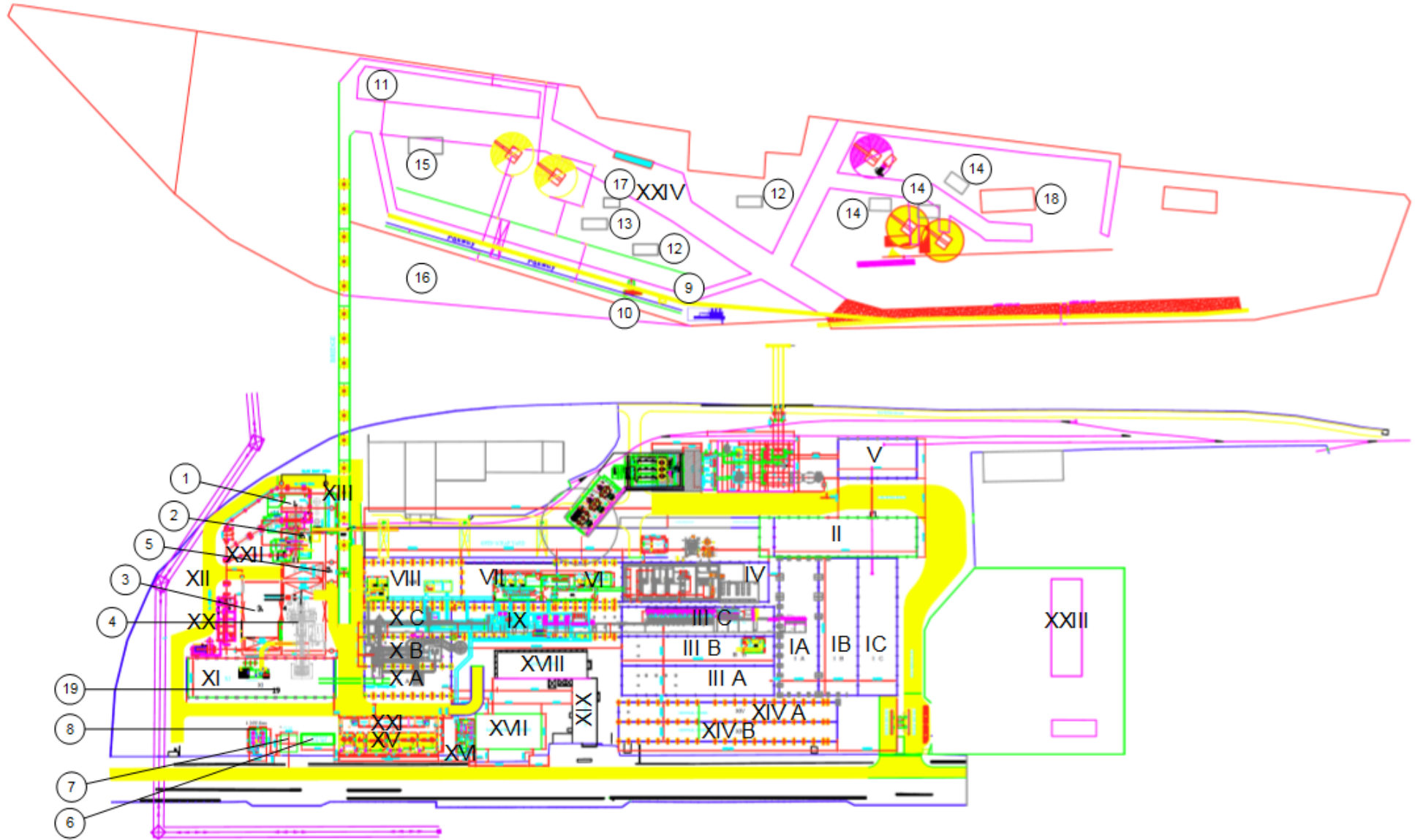
სქემა 4.2.1.1. საწარმოს გენ-გეგმა
