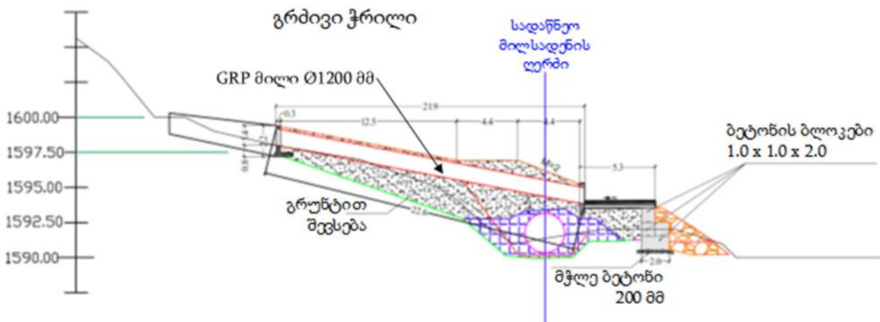
ნახაზი 3.2.4. პკ 17+13 მდებარე მშრალი ხევის წყალგამტარი ნაგებობის ჭრილი
