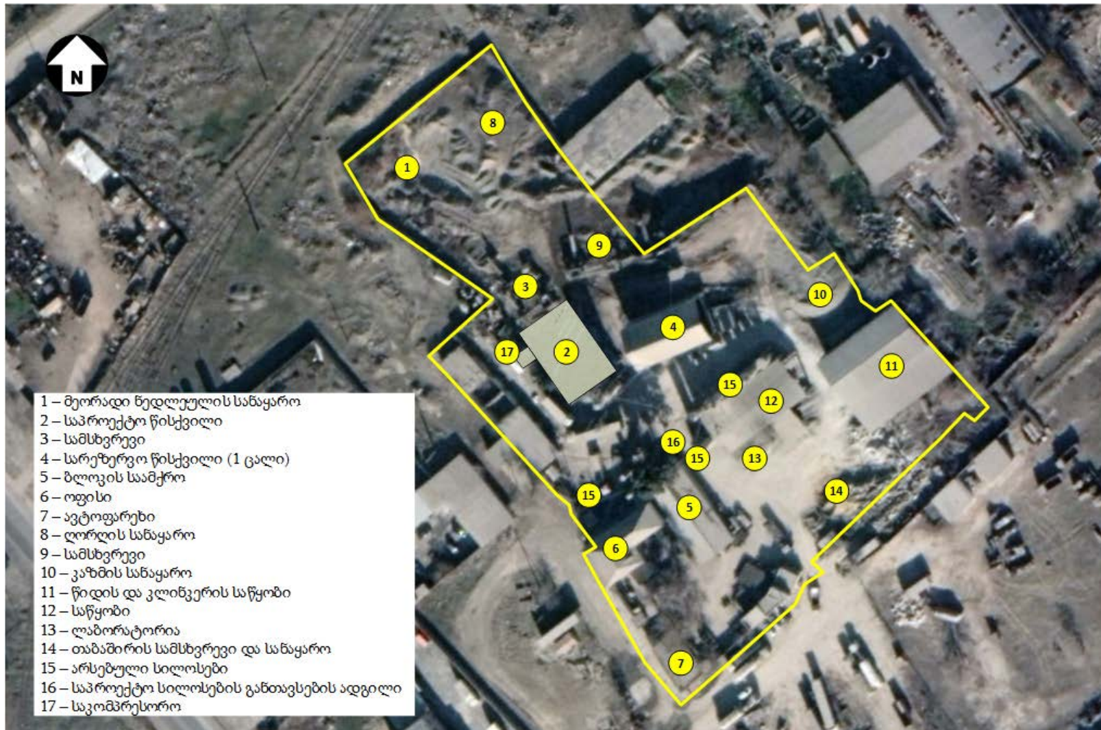
სურათი 4.3.1. საწარმოს გენ-გეგმა საპროექტო ინფრასტრუქტურის დატანით
