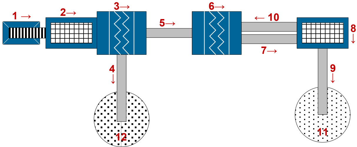
ნახაზი 3.1. სამსხვრევის ტექნოლოგიური სქემა
