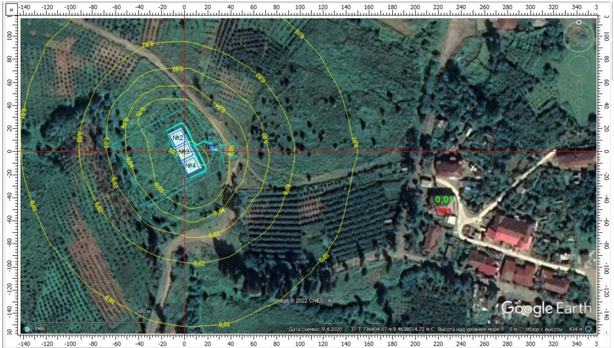
ჯამური ზემოქმედების 6003 ჯგუფის (კოდები 303+333) მაქსიმალური კონცენტრაციები საკონტროლო წერტილებში (№ 1÷2 უახლოს დასახლებებთან)
