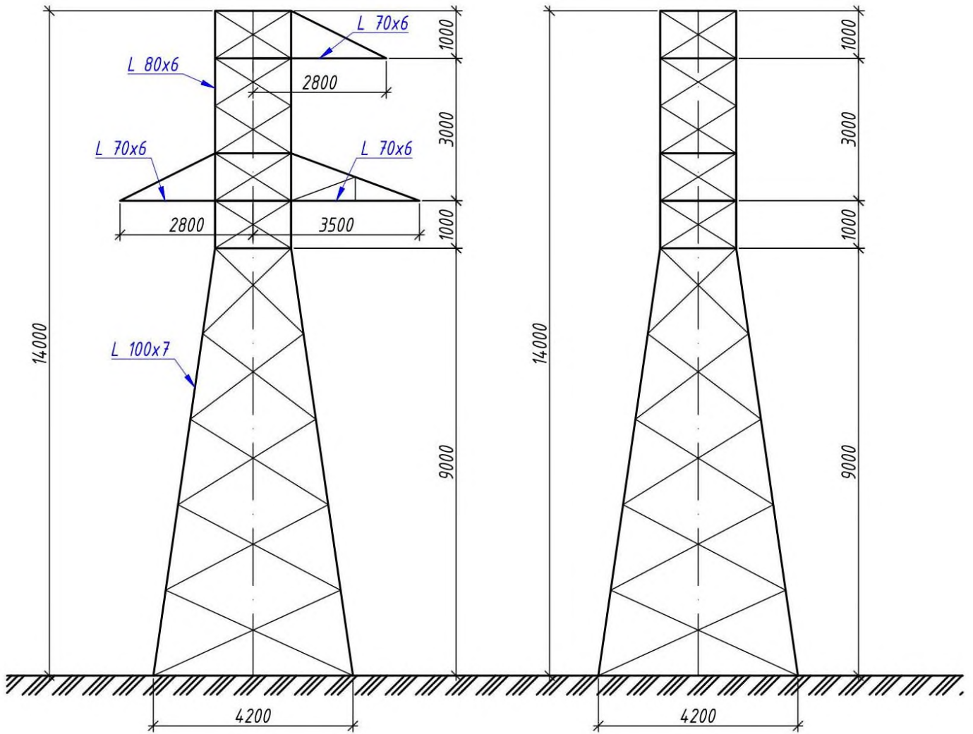
ნახაზი 2 ანძის ტიპური სქემა
