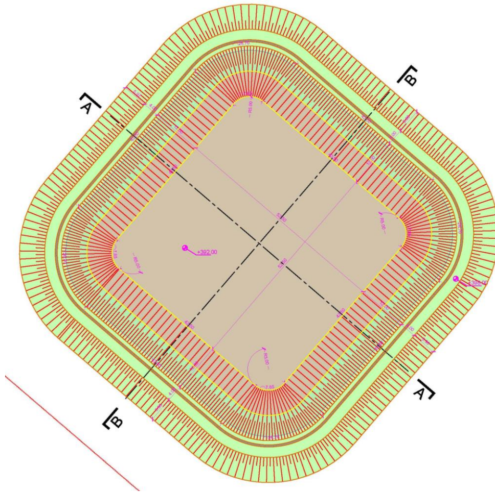
ნახაზი 4. წყალშემკრები რეზერვუარი
