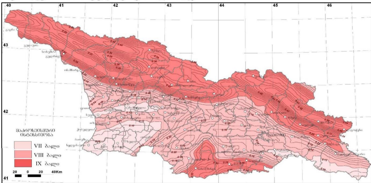
სეისმური საშიშროების რუკა მაქსიმალურ კორიზონტულ აჩქარებასა და ბალებში
