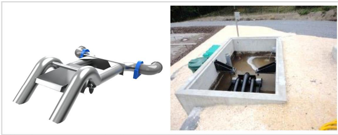
სურათი 3.2.5.1. ავტომატური რეგულირების სიფონი
