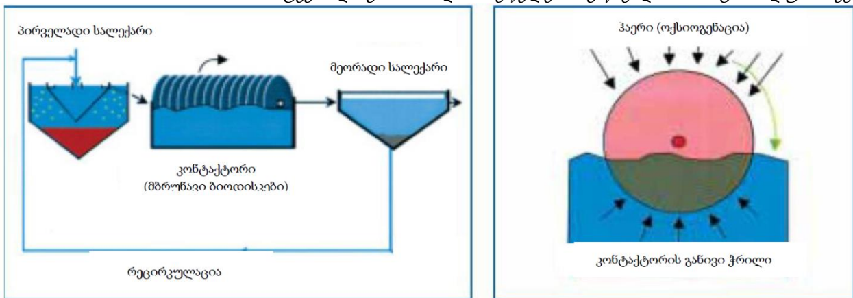
ნახაზი 3.1. RBC-ს ტექნოლოგიით ჩამდინარე წყლების გაწმენდის პრინციპიული სქემა
