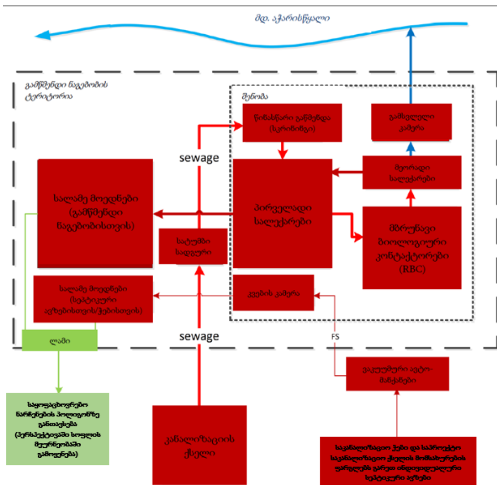
ნახაზი 3.4.1. ჩამდინარე წყლების გაწმენდის ტექნოლოგიური სქემა
