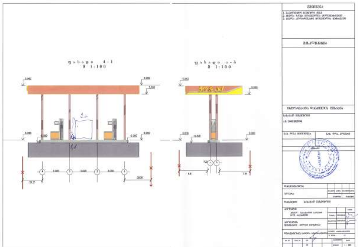
ნახაზი 2.2. ავტოგასამაღტი სადგური გადახურვის სქემით.
