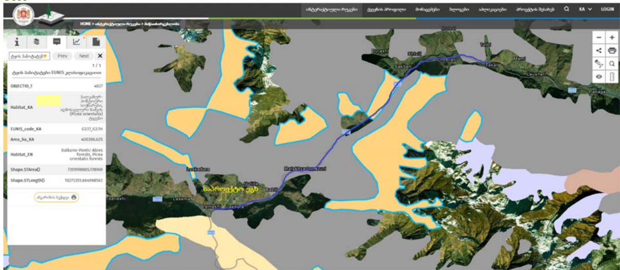
სურათი 6.3.3. ტყის ჰაბიტატები EUNIS კლასიფიკაციით_ბალკანურ-პონტოური სოჭნარები, ადმოსავლური ნაძვის ტყეები
