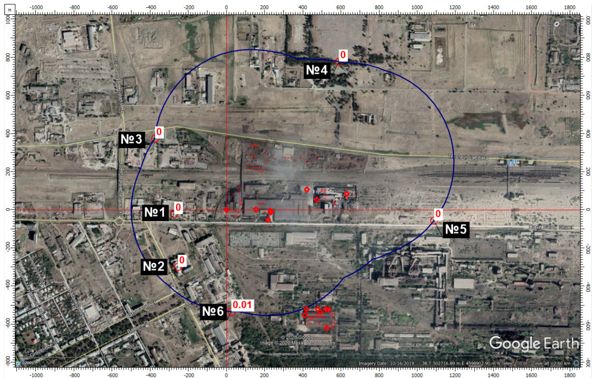
ნივთიერება: 0328 ნახშირბადი (კვარტლი). მაქსიმალური კონცენტრაციები უახლოეს საცხოვრებელ სახლთან (წერტ. N1,2) და ნორმირებულ 500 მ. ზონის საზღვართან (წერტ.3,4,5,6).
