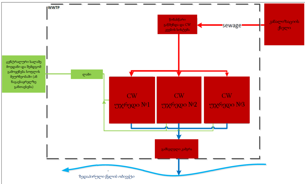
ნახაზი 3.1. ჩამდინარე წყლების გაწმენდის ტექნოლოგიური სქემა
