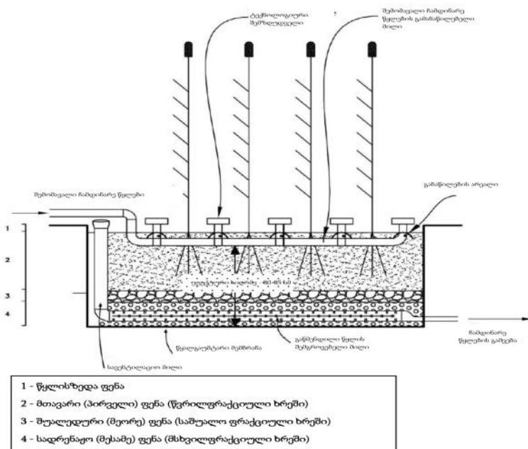
სურათი 2.3.1.1. ვერტიკალურ ნაკადიანი ჰიდრობოტანიკური მოედნის - . ე.წ. „აშენებული ჭაობების“ ტიპიური სქემა
