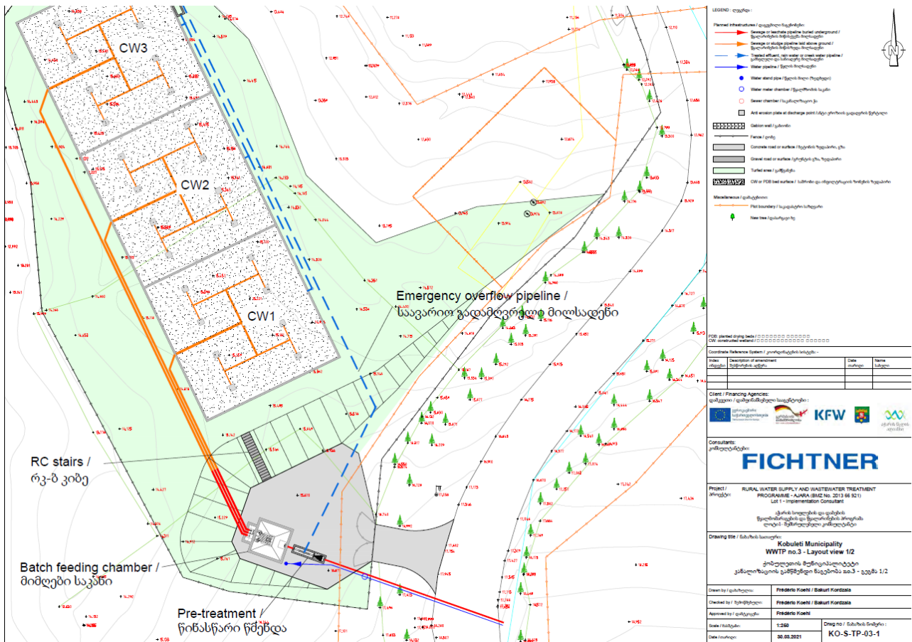
ნახაზი 2.3.5.1. გამწმენდი ნაგებობის გენ-გეგმა
