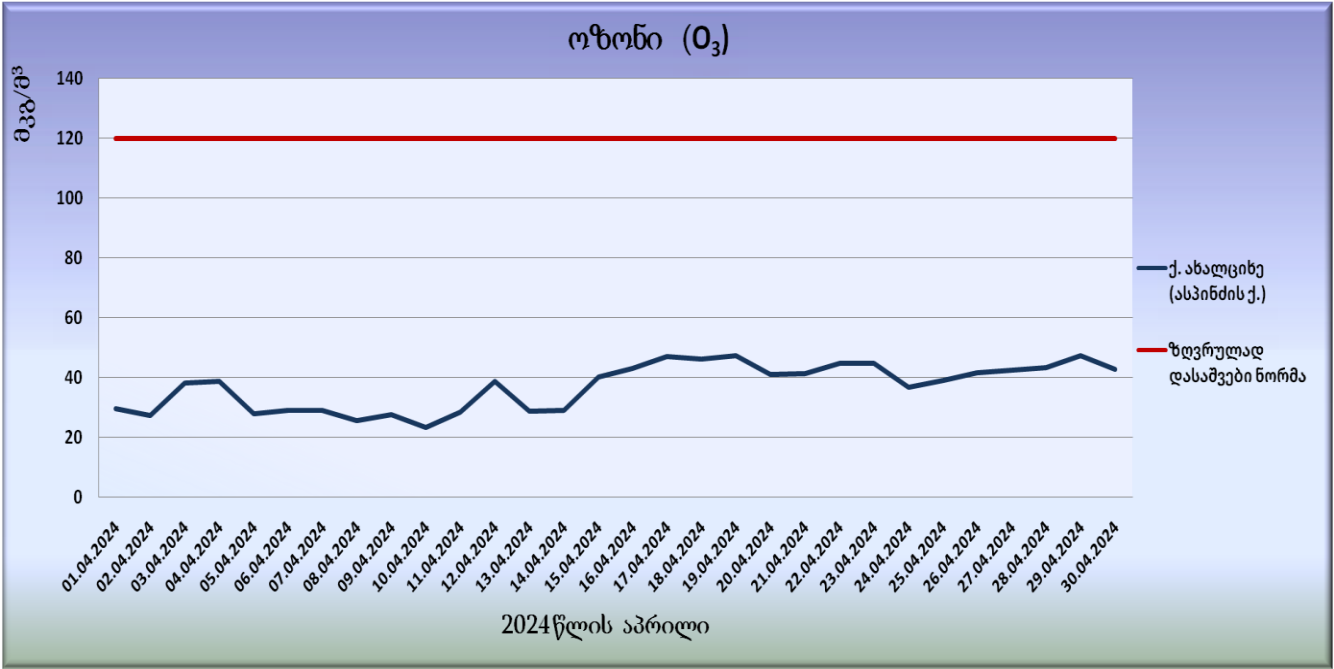
გრფიკი N20. ოზონის (O 3 ) რეასაათიანი საშუალო კონცენტრაციები
