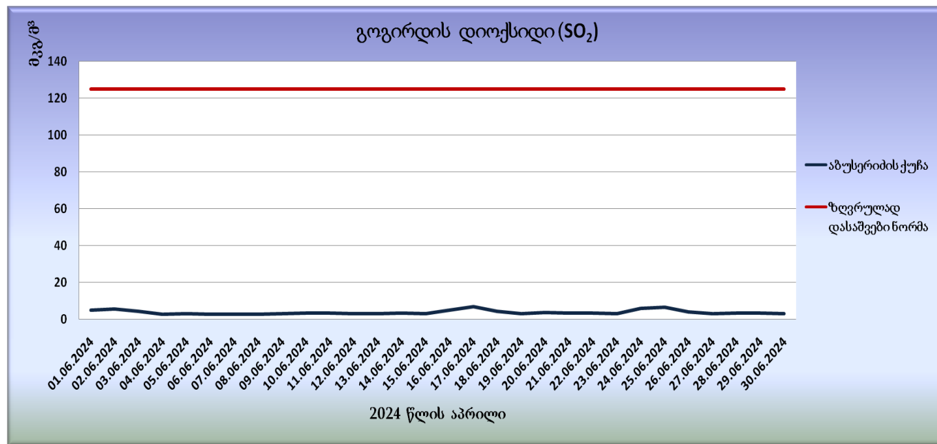
გრაფიკი N6. გოგირდის დიოქსიდის ( \text{SO}_2 ) საშუალოდღეობრივი კონცენტრაციები
