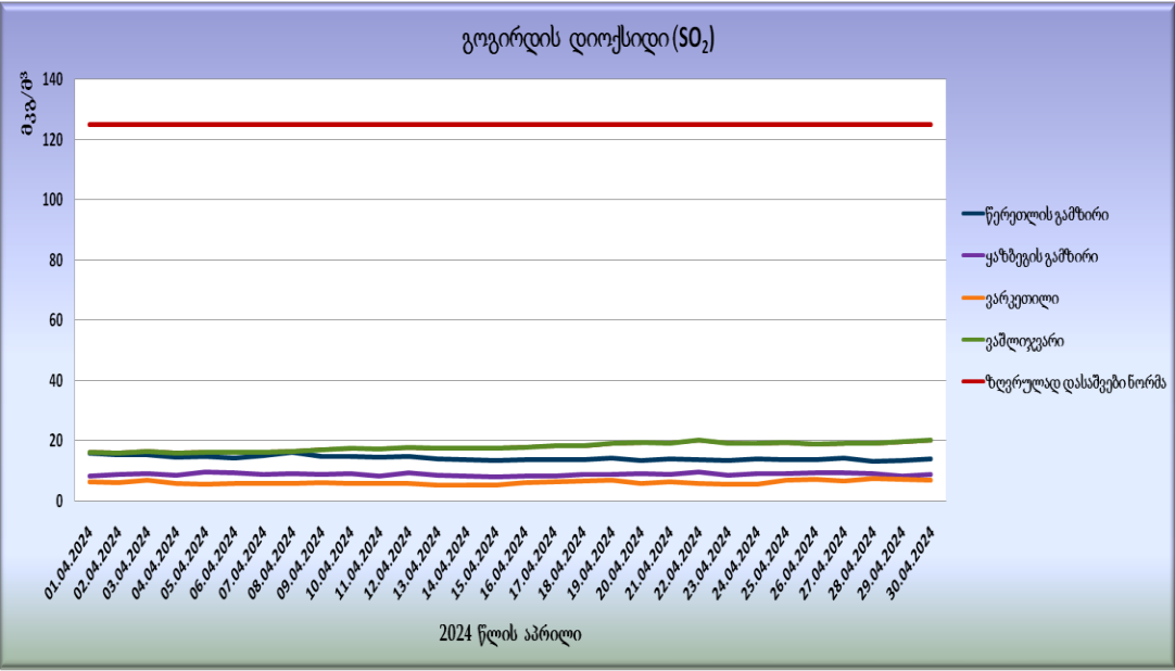
გრაფიკი N1. გოგირდის დიოქსიდის (SO 2 ) საშუალო სადღეღმისოკონცენტრაციები
