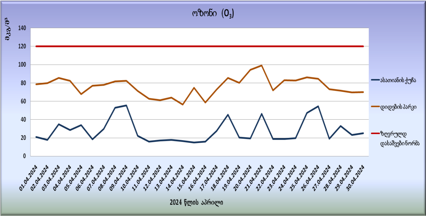
გრაფიკი N17. ოზონის (O 3 ) რეგისტრირებული საშუალო კონცენტრაციები
