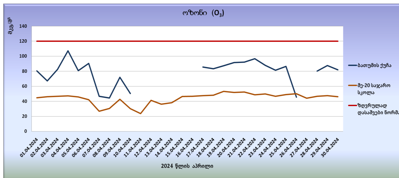
გრფიკი N14. ოზონის (O 3 ) მაქსიმალური ყოველდღიური რეგისტრირებული საშუალო კონცენტრაციები
