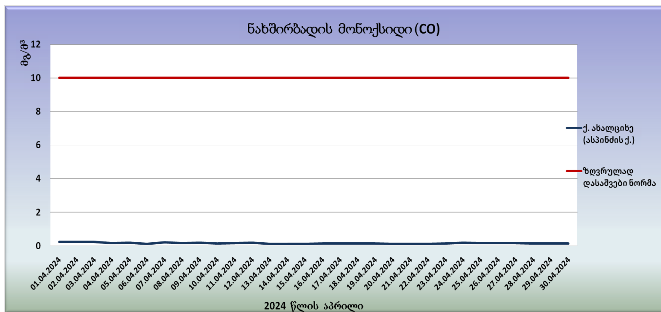
გრფუკი N22. ნახშირბადის მონოქსიდის (CO) მაქსიმალური ყოველდღიური რეგსაათიანი საშუალო კონცენტრაციები
