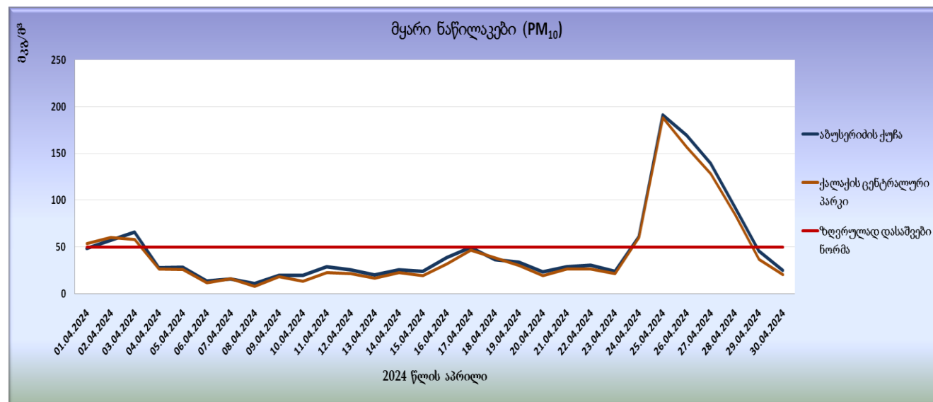
გრაფიკი N7. მყარი ნაწილაკების (PM 10 ) საშუალო დღეისო კონცენტრაციები
