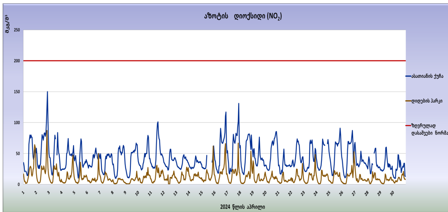
გრაფიკი N18. აზოტის დიოქსიდის ( \text{NO}_2 ) 1 სათიანო გასაშუალებით მიღებული კონცენტრაციები კონცენტრაციები
