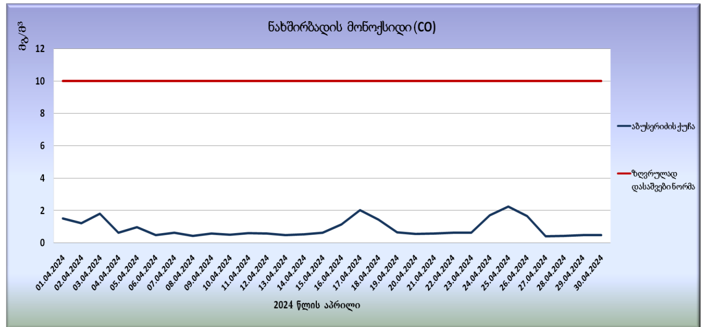
გრაფიკი N10. ნახშირბადის მონოქსიდის (CO) მაქსიმალური ყოველდღიური რეგსაათიანი საშუალო კონცენტრაციები
