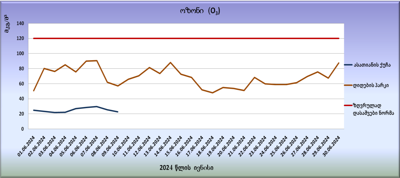
გრაფიკი N19. ოზონის (O 3 ) რეგისტრაციის საშუალო კონცენტრაციები
