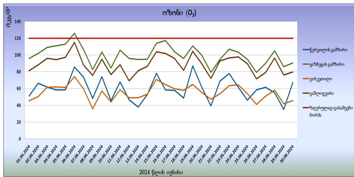
გრაფიკი N4. ოზონის (O 3 ) მაქსიმალური ყოველდღიური რეასაათანი საშუალოკონცენტრაციები
