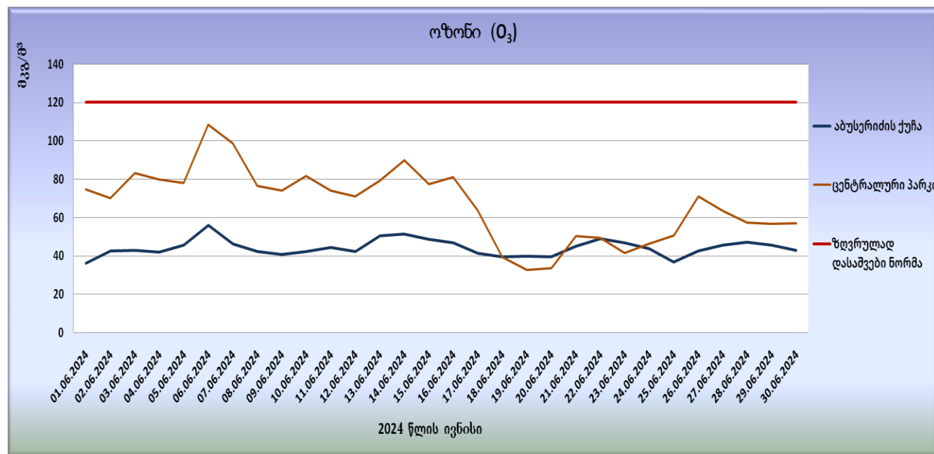
გრაფიკი N9. ოზონის (O 3 ) მაქსიმალური ყოველდღიური რეგისტრაციის საშუალო კონცენტრაციები
