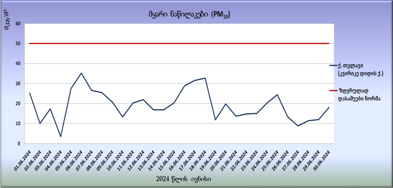
გრფიკი N31. მყარი ნაწილაკების (PM 10 ) საშუალო დღეისო კონცენტრაციები
