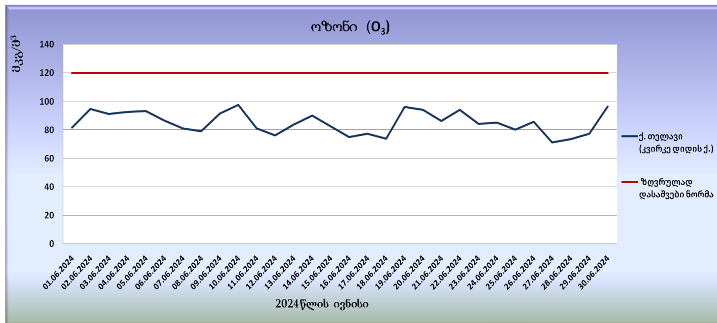
გრაფიკი N33. ოზონის (O 3 ) მაქსიმალური ყოველდღიური რეგსაათიანი საშუალო კონცენტრაციები
