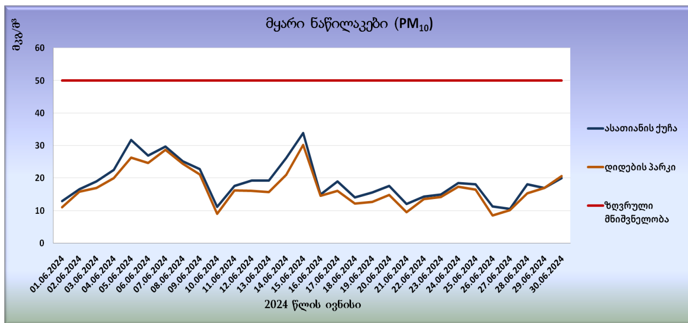
გრფიკი N17. მყარი ნაწილაკების (PM 10 ) საშუალო დღეის მისოკონცენტრაციები
