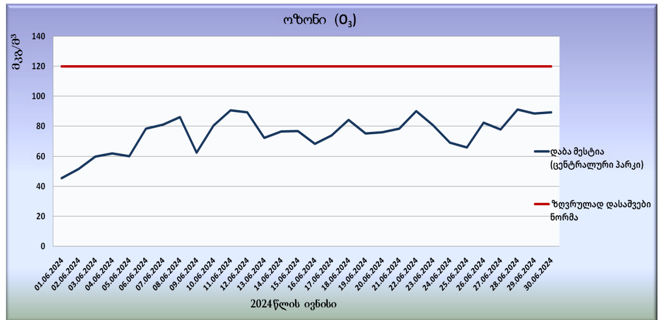
გრფიკი N34. ოზონის ( O_3 ) მაქსიმალური ყოველდღიური რეგისტრაციის საშუალო კონცენტრაციები
