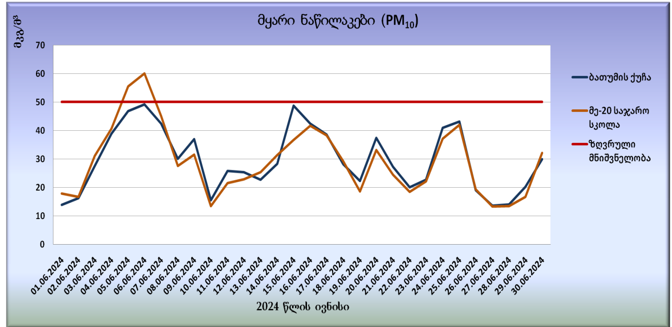
გრაფიკი N12. მყარი ნაწილაკების (PM 10 ) საშუალო დღეისო კონცენტრაციები
