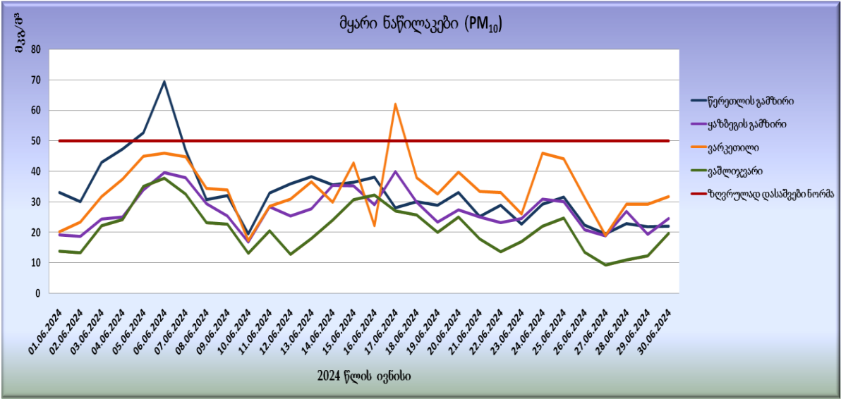
გრაფიკი N2. მყარი ნაწილაკების (PM 10 ) საშუალო სადღისო კონცენტრაციები
