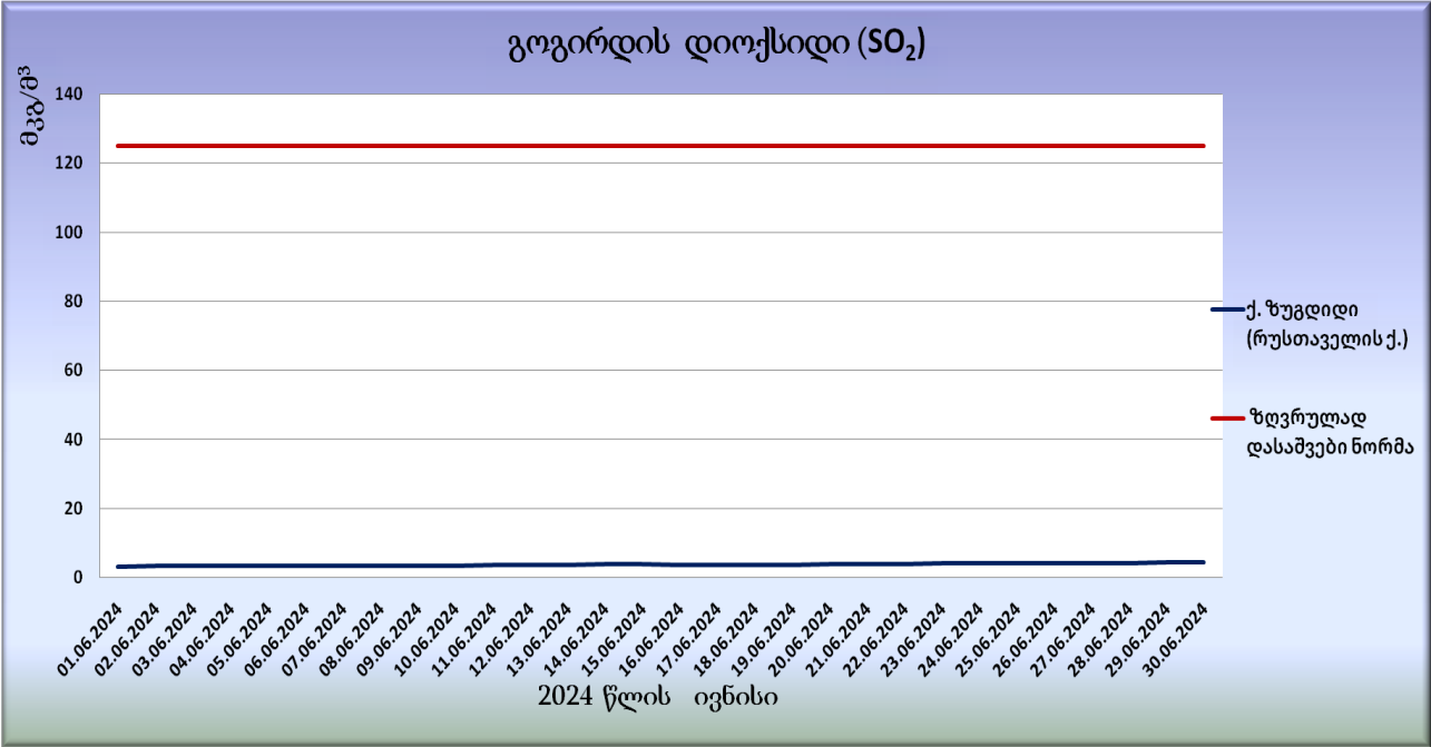
გრფიკი N26. გოგირდის დიოქსიდის (SO 2 ) საშუალო საღებო დონის კონცენტრაციები
