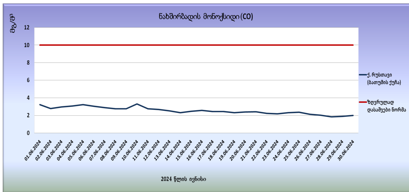
გრაფიკი N15. ნახშირბადის მონოქსიდის (CO) მაქსიმალური ყოველდღიური რეგსაათიანი საშუალო კონცენტრაციები
