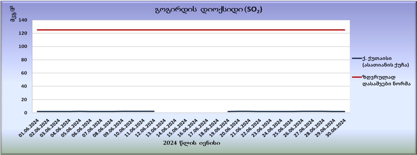
გრფუკი N16. გოგირდის დიოქსიდის (SO 2 ) საშუალო დღე-ღამის კონცენტრაციები
