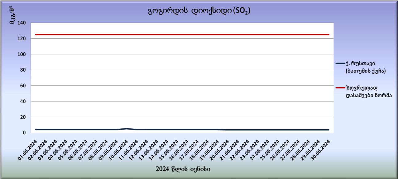
გრფიკი N11. გოგირდის დიოქსიდის (SO 2 ) საშუალო დღეობრივი კონცენტრაციები
