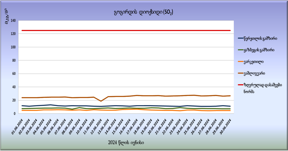
გრფუკი N1. გოგირდის დიოქსიდის (SO 2 ) საშუალოსაღებლისოკონცენტრაციები
