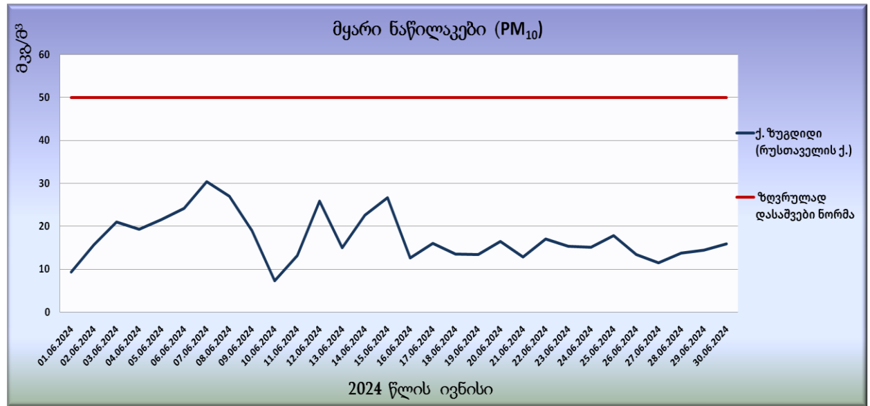
გრაფიკი N27. მყარი ნაწილაკების (PM 10 ) საშუალო დღეისო კონცენტრაციები
