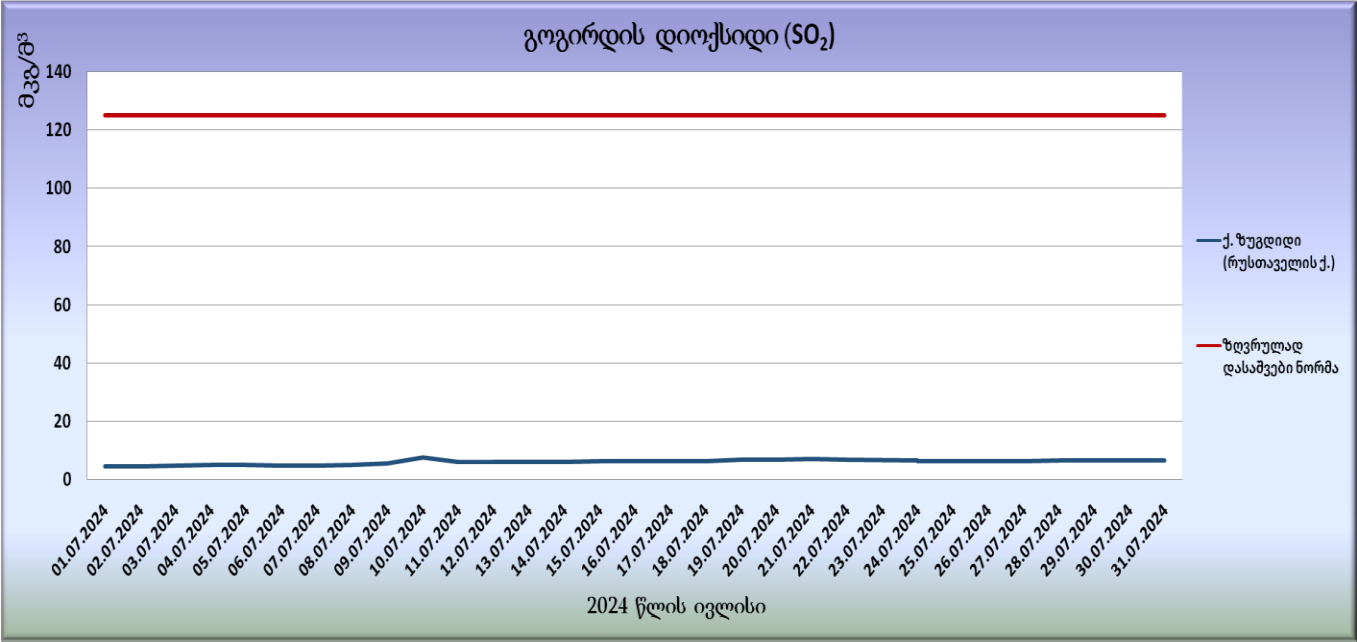
გრფიკი N26. გოგირდის დიოქსიდის (SO 2 ) საშუალო სადღეისო კონცენტრაციები
