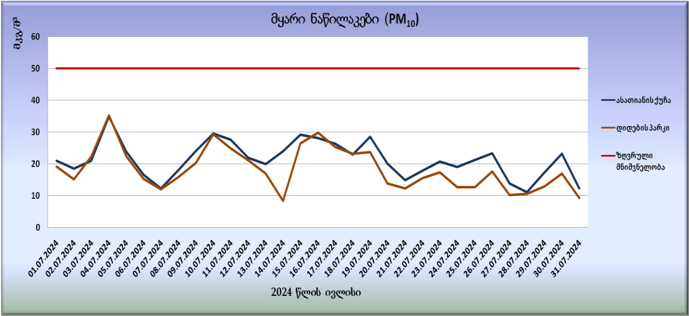
გრფიკი N17. მყარი ნაწილაკების (PM 10 ) საშუალო დღეისო კონცენტრაციები
