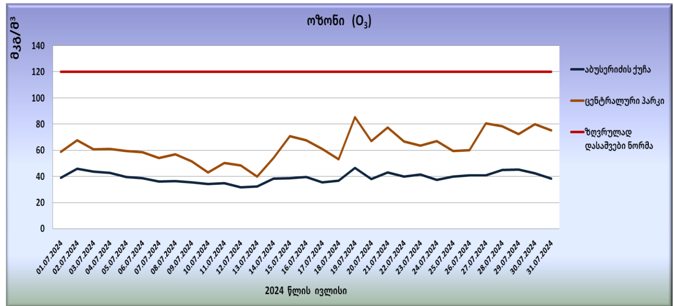
გრაფიკი N9. ოზონის (O 3 ) მაქსიმალური ყოველდღიური რეგისტრირებული საშუალო კონცენტრაციები
