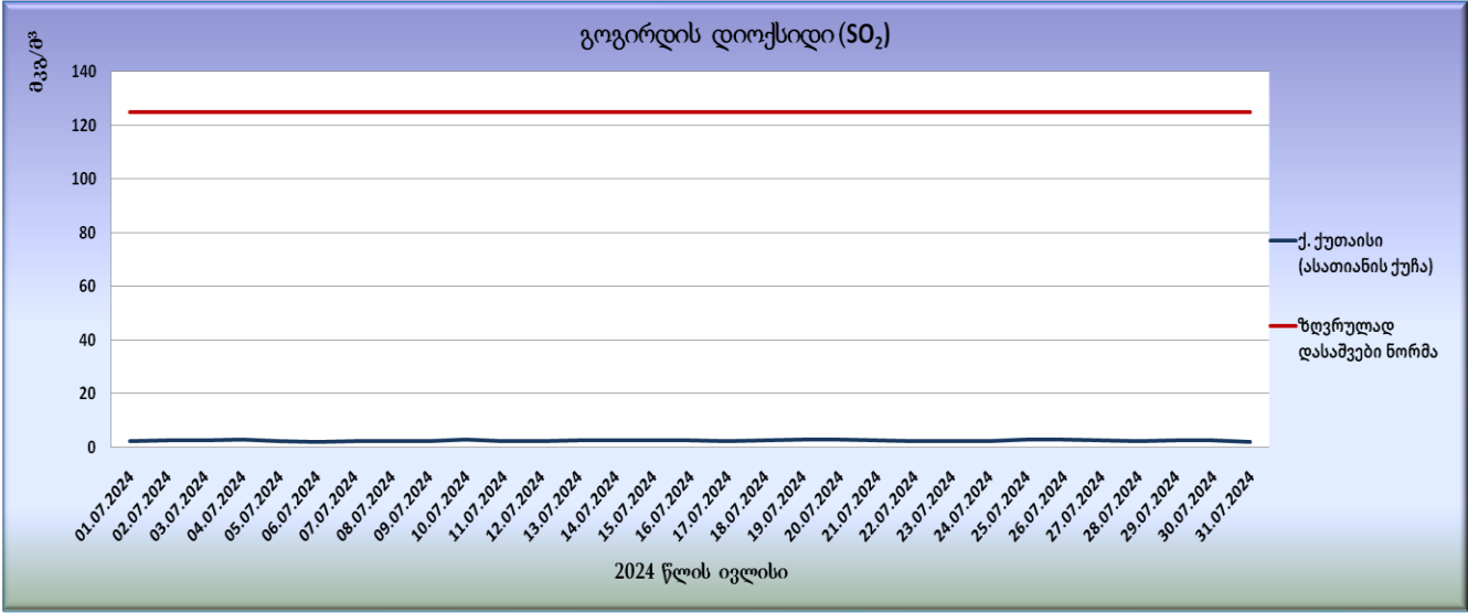
გრფიკი N16. გოგირდის დიოქსიდის (SO 2 ) საშუალო დღეისო კონცენტრაციები
