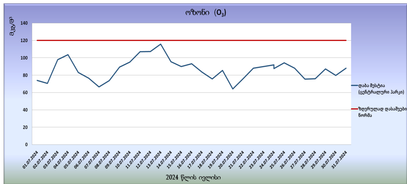
გრფიკი N34. ოზონის (O 3 ) მაქსიმალური ყოველდღიური რეასაათიანი საშუალო კონცენტრაციები
