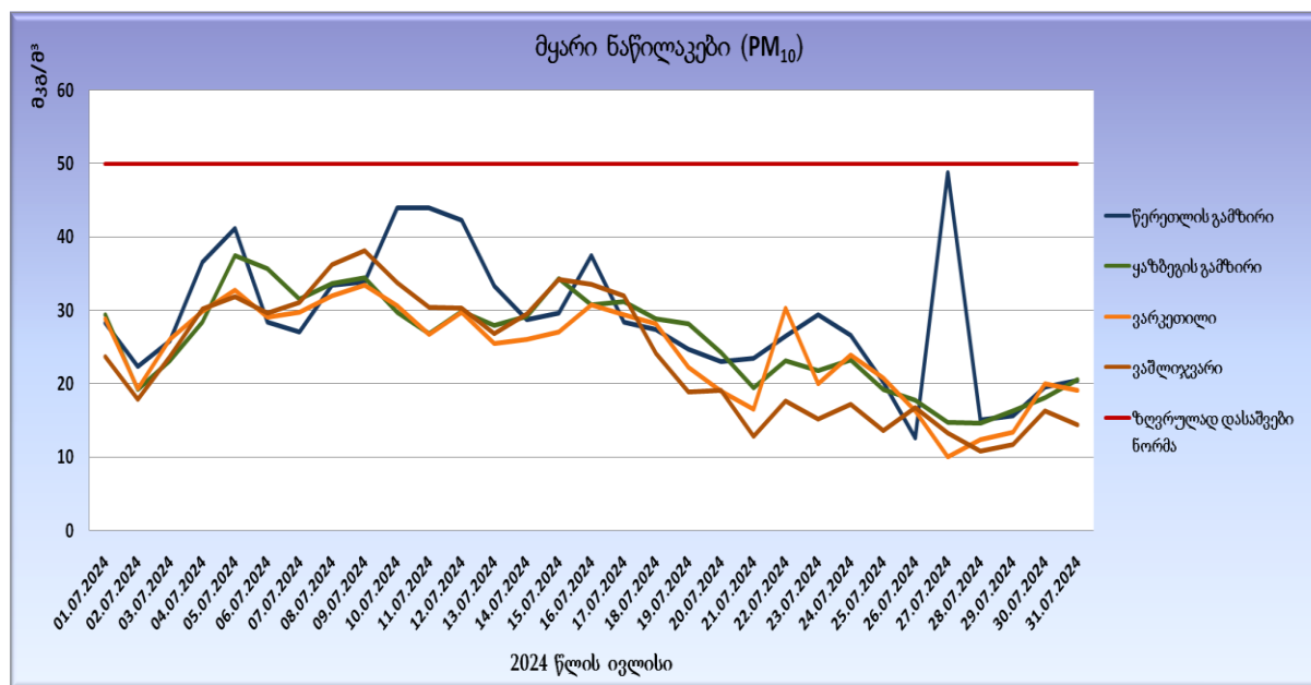
გრაფიკი N2. მყარი ნაწილაკების (PM 10 ) საშუალოდღმისოკონცენტრაციები
