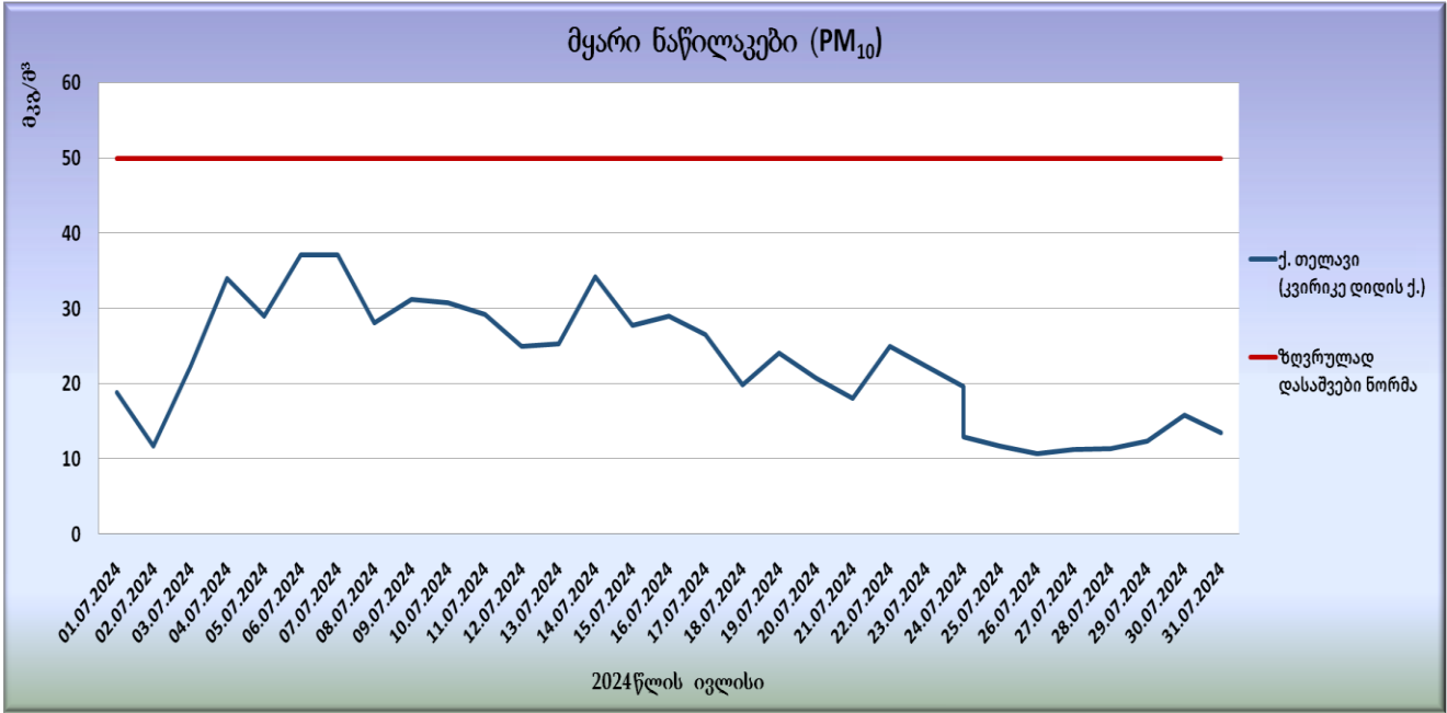
გრფიკი N31. მყარი ნაწილაკების (PM 10 ) საშუალო სადღეისო კონცენტრაციები
