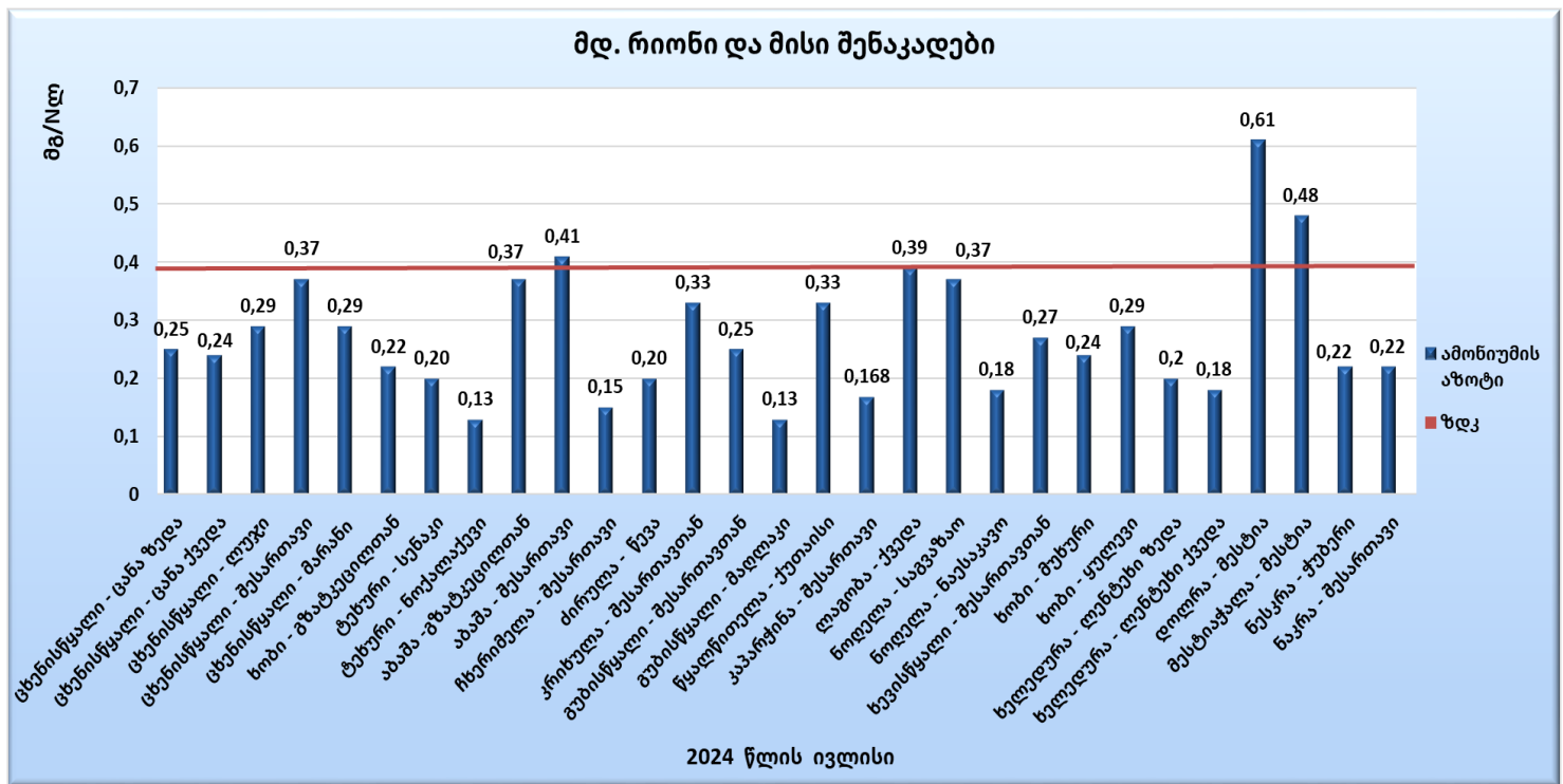
გრაფიკი 23. მდ.რიონი და მისი შენაკადები - ამონიუმის აზოტი, ივლისი, 2024
