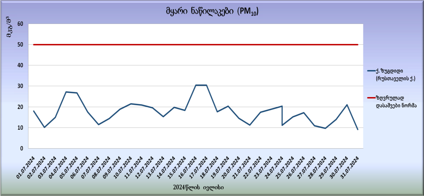
გრაფიკი N27. მყარი ნაწილაკების (PM 10 ) საშუალო სადღეისო კონცენტრაციები
