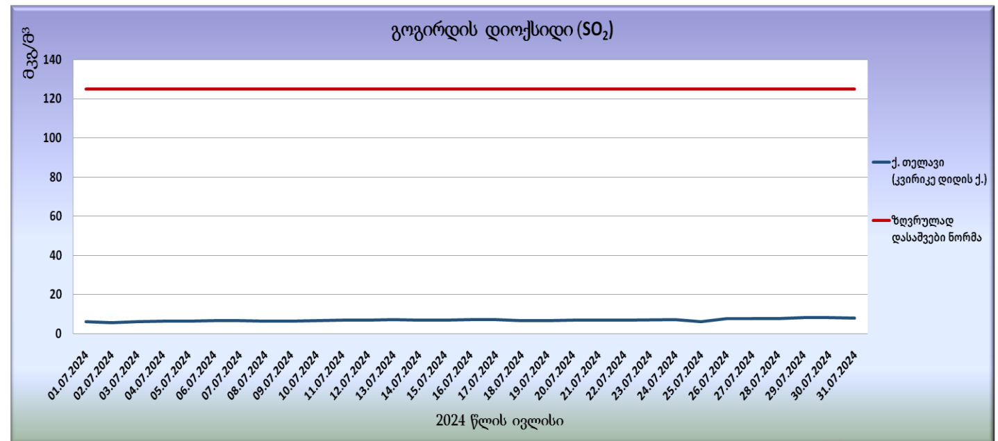
გრფიკი N30. გოგირდის დიოქსიდის (SO 2 ) საშუალო სადღეღამისო კონცენტრაციები
