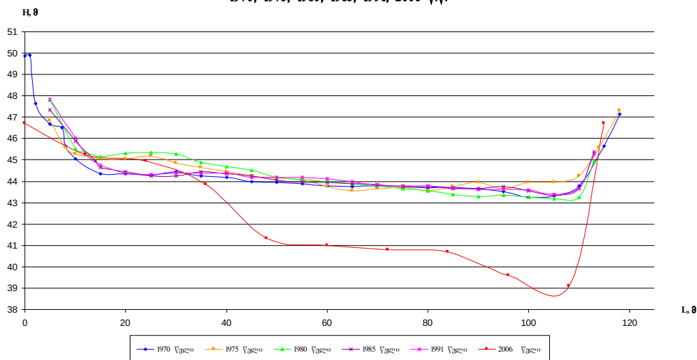
მდ.ჭოროხის განივი ჭრილები მირვეთთან 1970, 1975, 1980, 1985, 1991, 2006 წ.წ.
