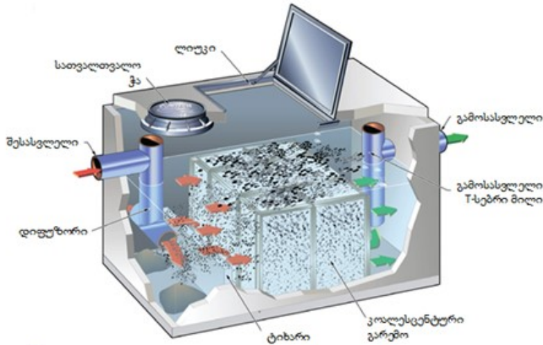
სურათი 8.2.2.3.1. კომპანია conteches-ის წარმოების წყლის კოალესცენტური სეპარატორი
