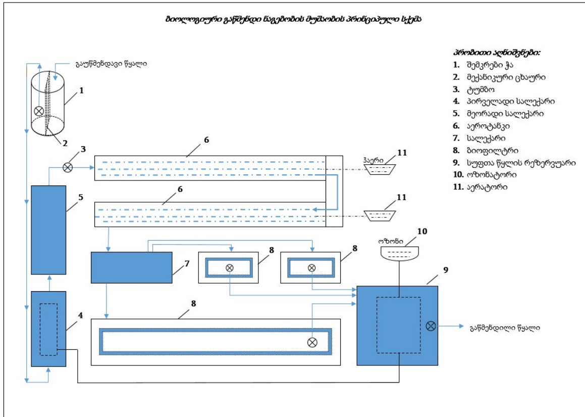
ნახაზი 8.2.1.4.1. ბიოლოგიური გამწმენდი ნაგებობის ტექნოლოგიური სქემა
