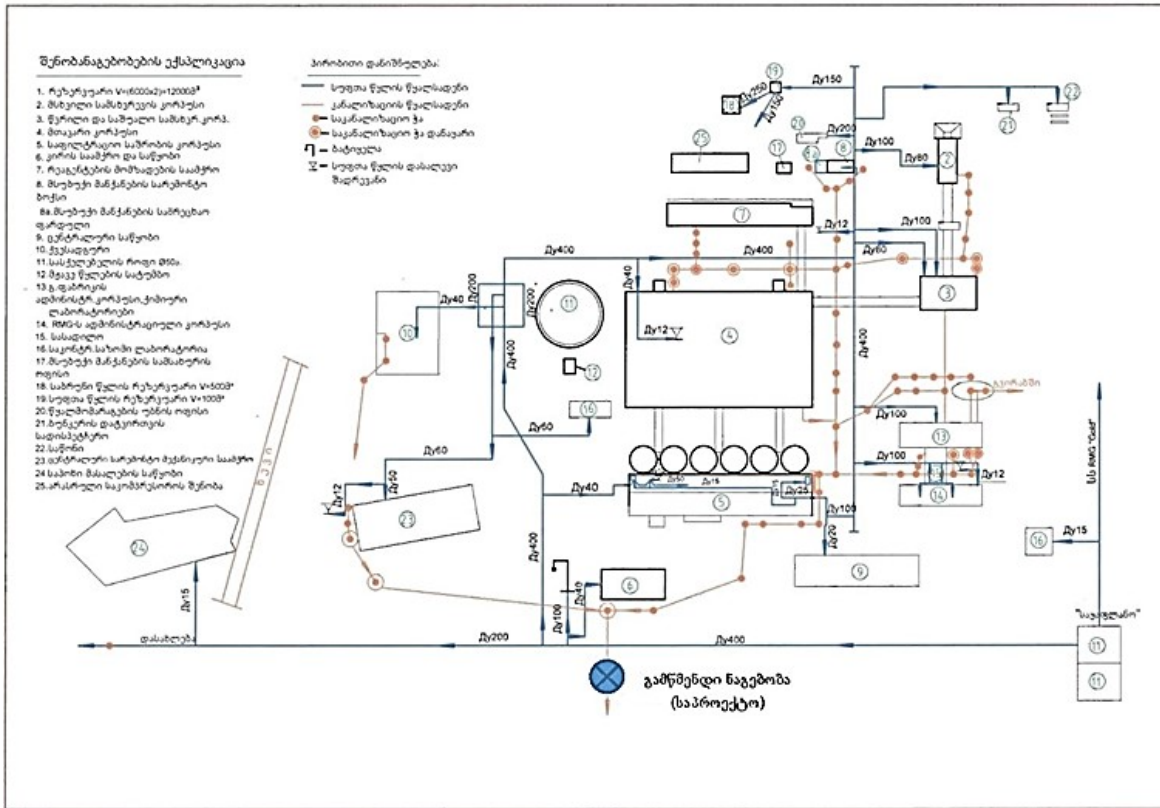
ნახაზი 8.1.1. წყალმომარაგების სქემა
