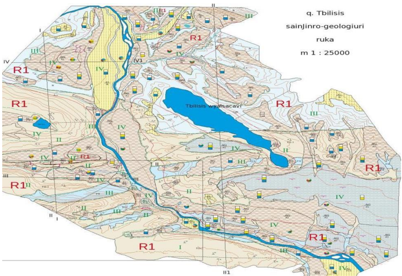
ფიგურა 5.4 კ. თბილისის საინჟინრო-გეოლოგიური რუკა
