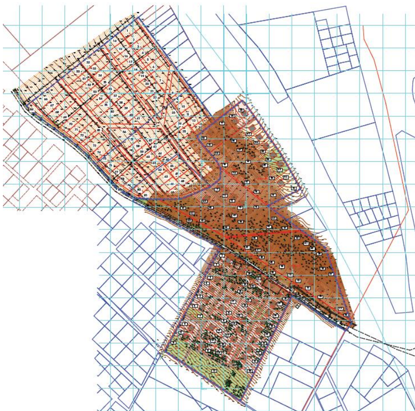
ფიგურა 3.1 საპროექტო გენგეგმა დასავლეთით შეთანხმებული განაშენიანების რეგულირების გეგმასთან ერთად
