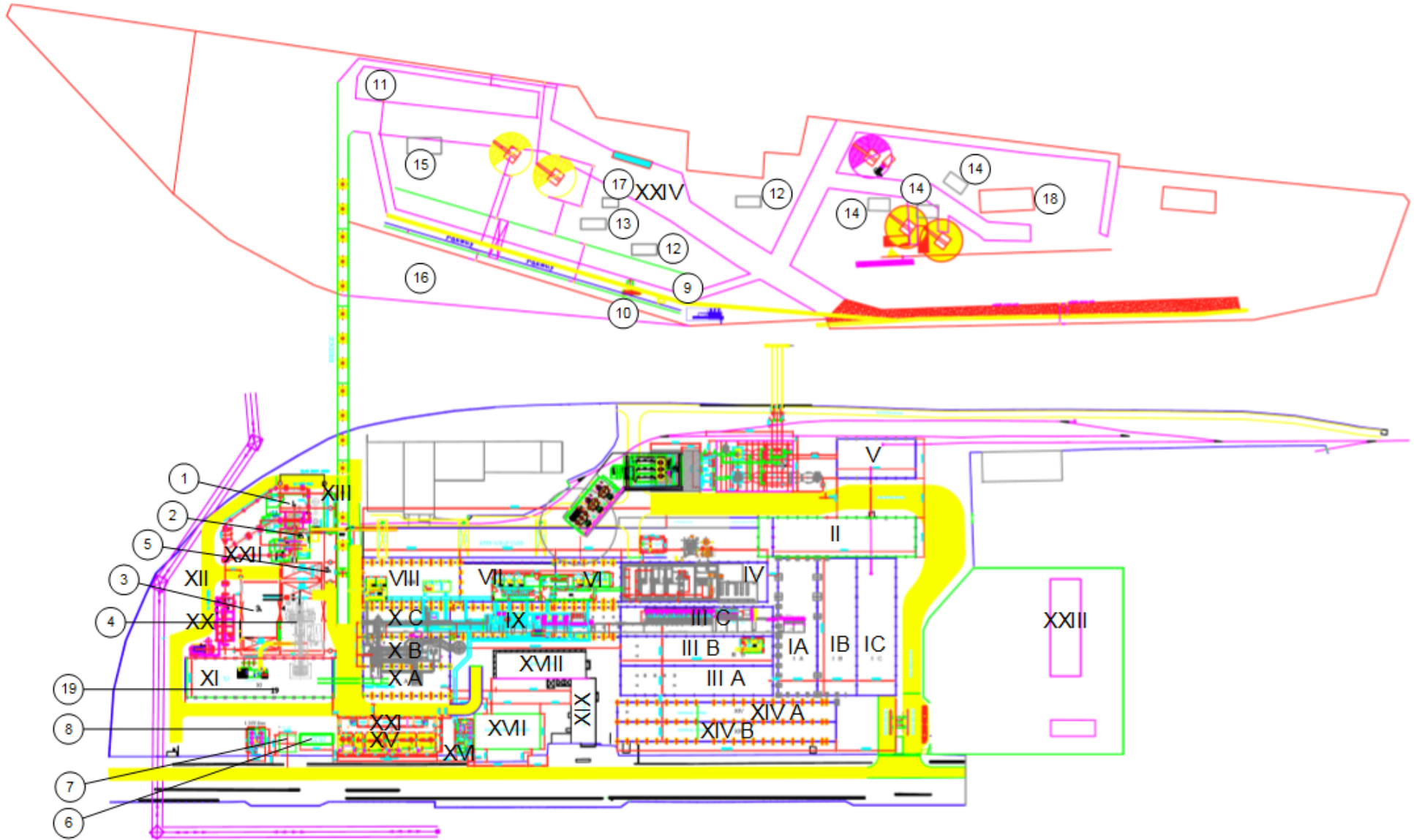
სქემა 3.2.1.1. საწარმოს გენ-გეგმა
