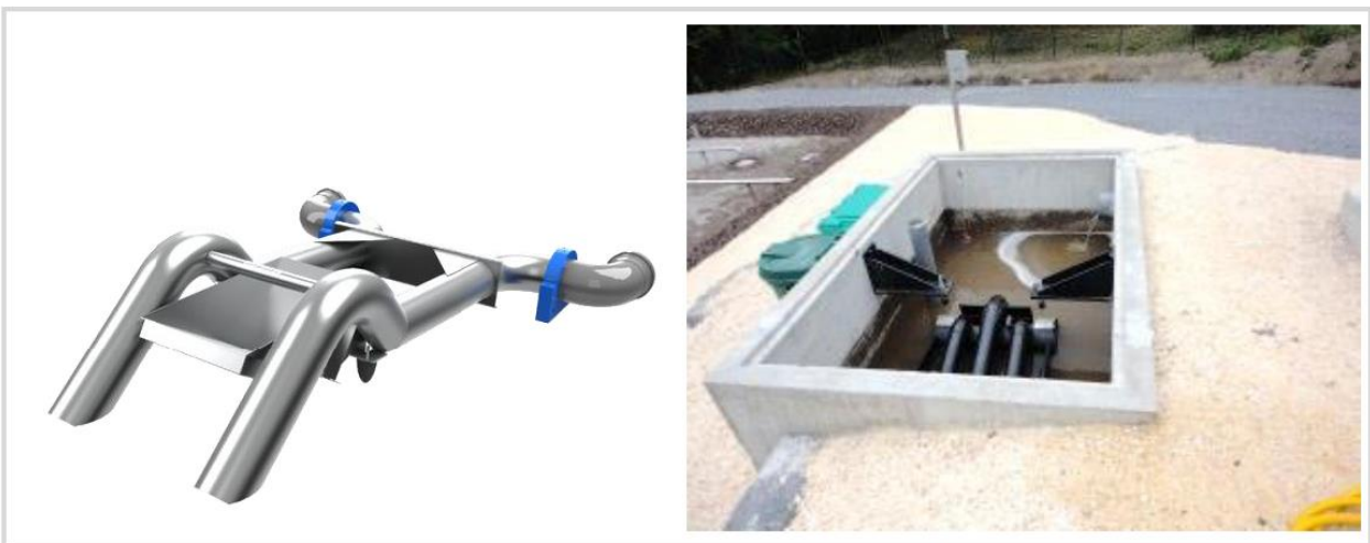
სურათი 2.4.1. ავტომატური რეგულირების სიფონი
