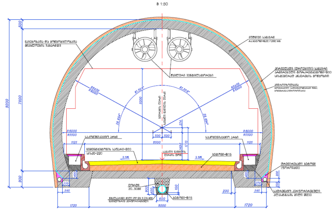
ნახაზი 2.3.1.3. საპროექტო გვირაბის ტიპური განივი პროფილი
