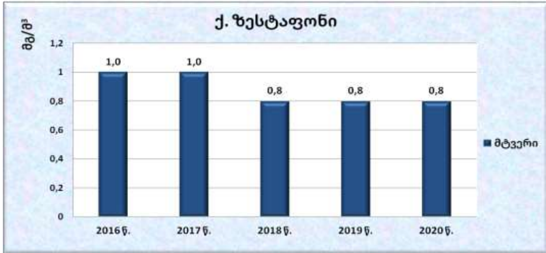
გრაფიკი 3. მტვერის ერთჯერადი მაქსიმალური კონცენტრაციები, მგ/მ³
