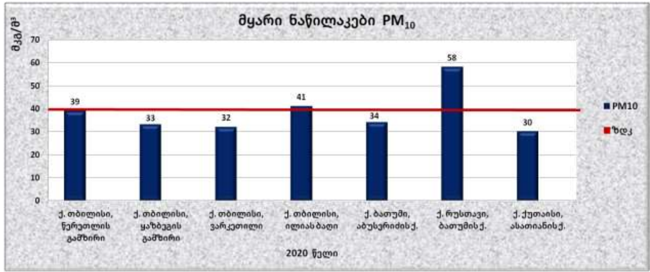
გრაფიკი 14. მყარი ნაწილაკების (PM 10 ) საშუალო წლიური კონცენტრაციები
