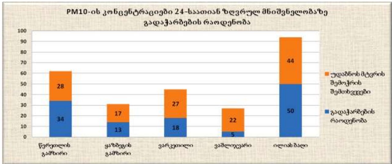
გრაფიკი N9. მყარი ნაწილაკების (PM 10 ) საშუალო სადღეღამისო კონცენტრაციების გადაჭარბებების დღეების რაოდენობა
