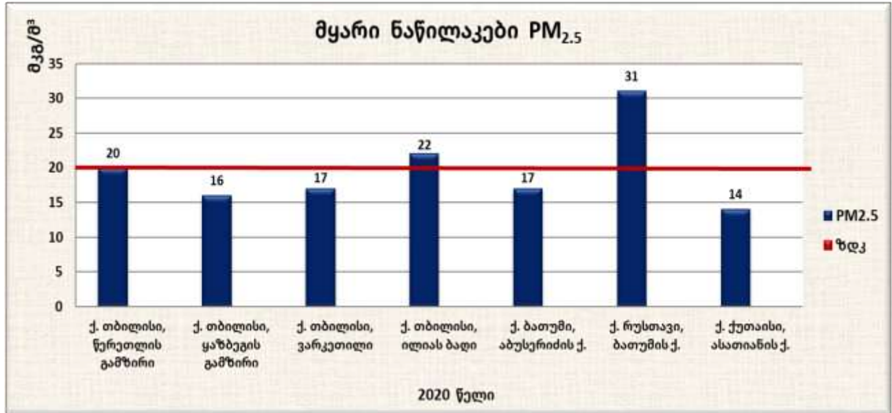
გრაფიკი 15 . მყარი ნაწილაკების (PM 2.5 ) საშუალო წლიური კონცენტრაციები
