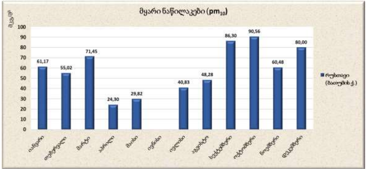
გრაფიკი 10. მყარი ნაწილაკების (PM 10 ) საშუალო სადღეღამისო კონცენტრაციების საშუალო თვიური მნიშვნელობები
