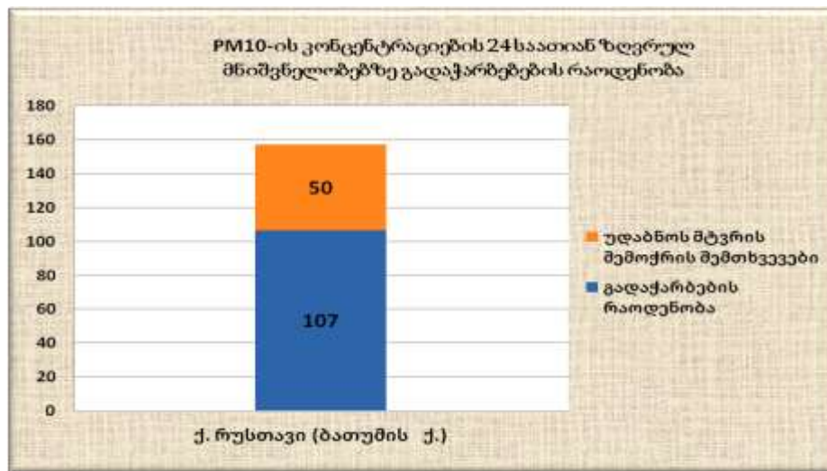
გრაფიკი 11. მყარი ნაწილაკების (PM 10 ) საშუალო სადღეღამისო კონცენტრაციების გადაჭარბებების რაოდენობა
