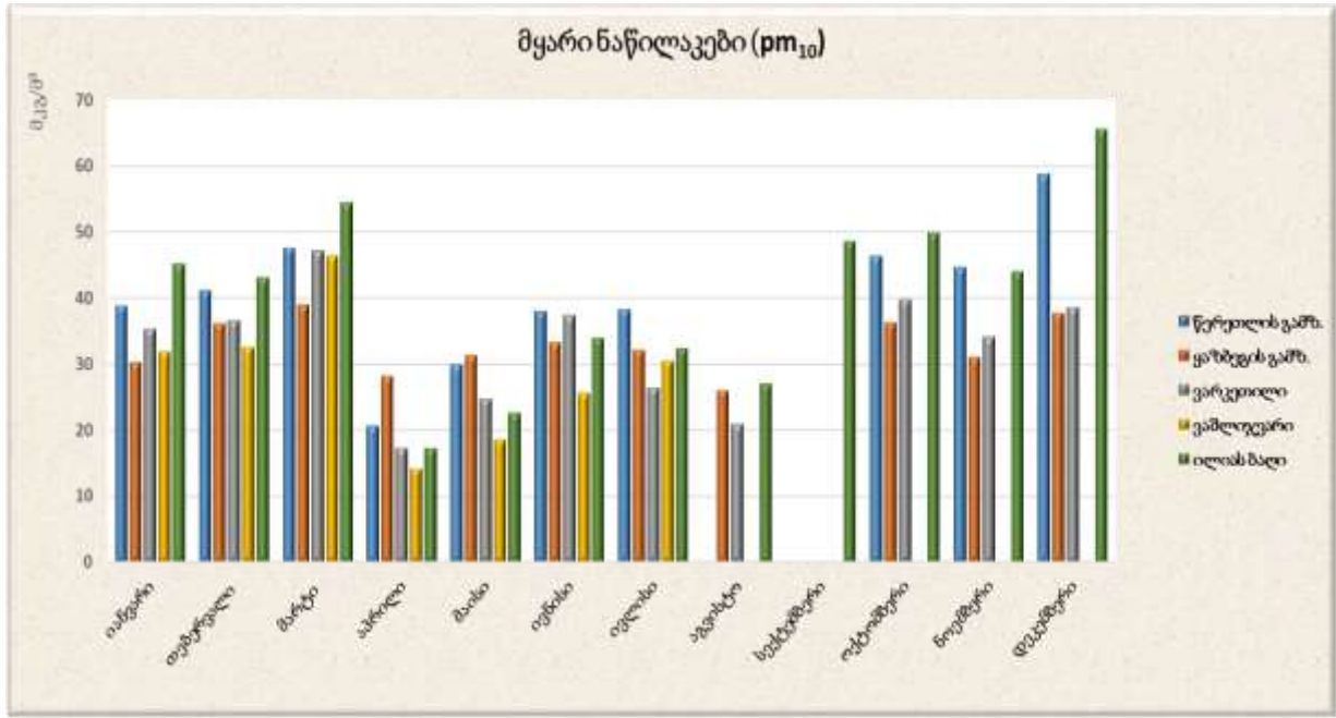
გრაფიკი 8. მყარი ნაწილაკების (PM 10 ) საშუალო სადღეღამისო კონცენტრაციების საშუალო თვიური მნიშვნელობები
