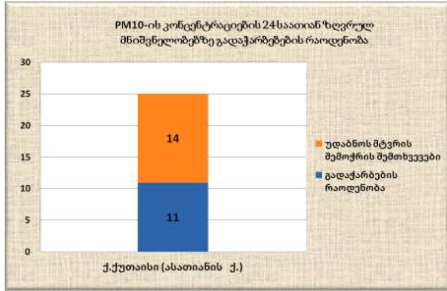
გრაფიკი N13. მყარი ნაწილაკების (PM 10 ) საშუალო სადღეღამისო კონცენტრაციების გადაჭარბებების რაოდენობა
