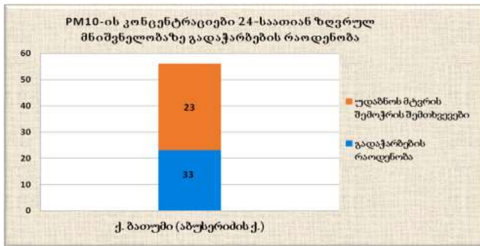
გრაფიკი 2. მყარი ნაწილაკების (PM 10 ) საშუალო სადღეღამისო კონცენტრაციების გადაჭარბებების დღეების რაოდენობა
