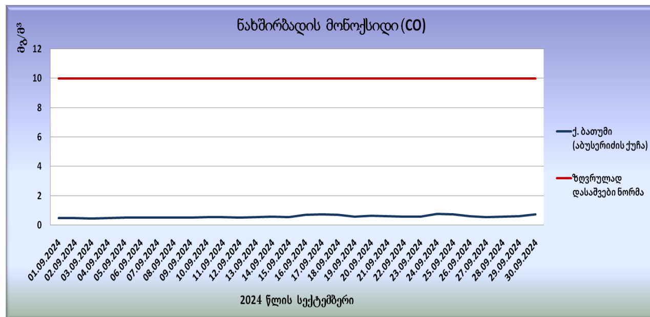
გრაფიკი N10. ნახშირბადის მონოქსიდის (CO) მაქსიმალური ყოველდღიური რეკორდები საშუალო კონცენტრაციები
