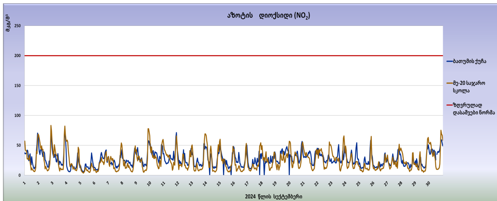
გრაფიკი N13 . აზოტის დიოქსიდის ( \text{NO}_2 ) 1 სთ-იანი გასაშუალოებით მიღებული კონცენტრაციები
