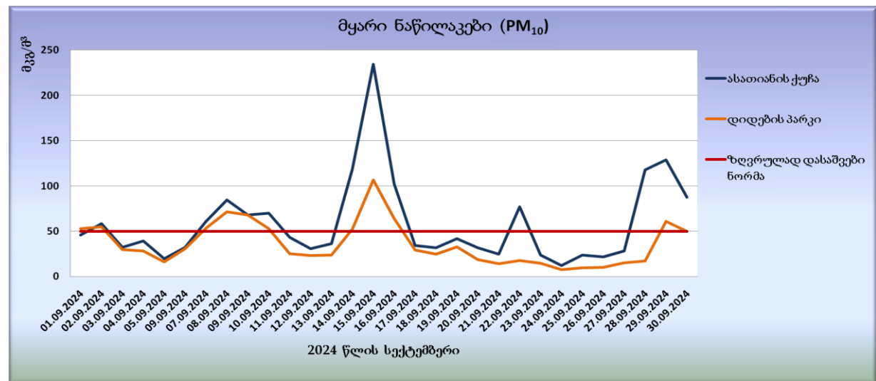
გრაფიკი N16. მყარი ნაწილაკების (PM 10 ) საშუალო სადღეღამისო კონცენტრაციები
