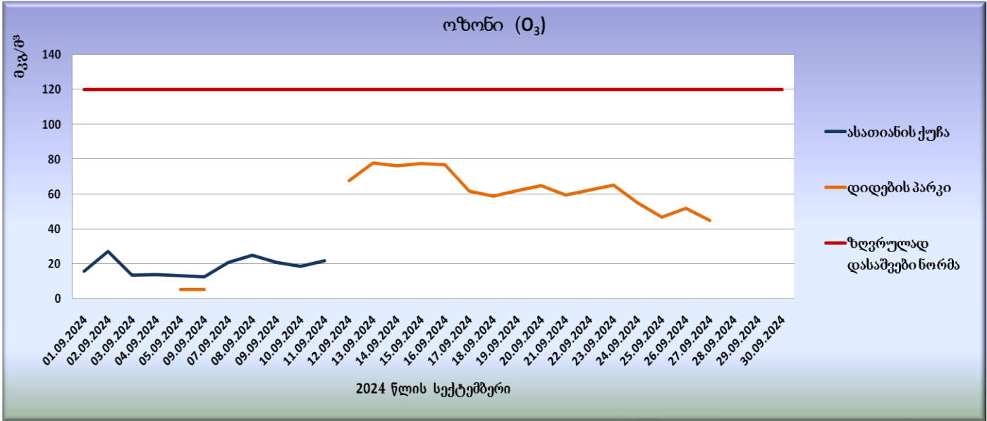
გრაფიკი N17. ოზონის (O 3 ) რეკორდული საშუალო კონცენტრაციები
