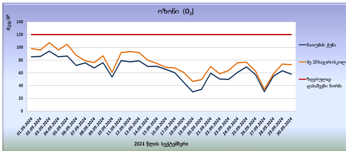
გრაფიკი N14. ოზონის (O 3 ) მაქსიმალური ყოველდღიური რეკონსტრუირებული კონცენტრაციები
