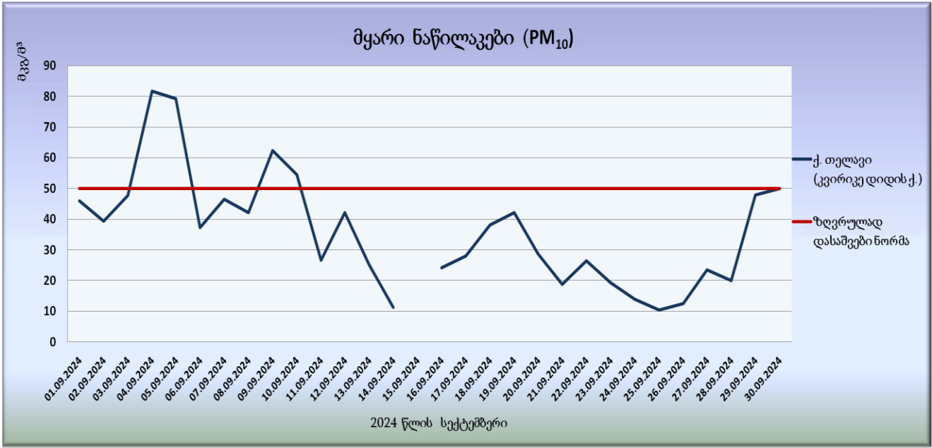
გრაფიკი N29. მყარი ნაწილაკების (PM 10 ) საშუალო სადღეღამისო კონცენტრაციები
