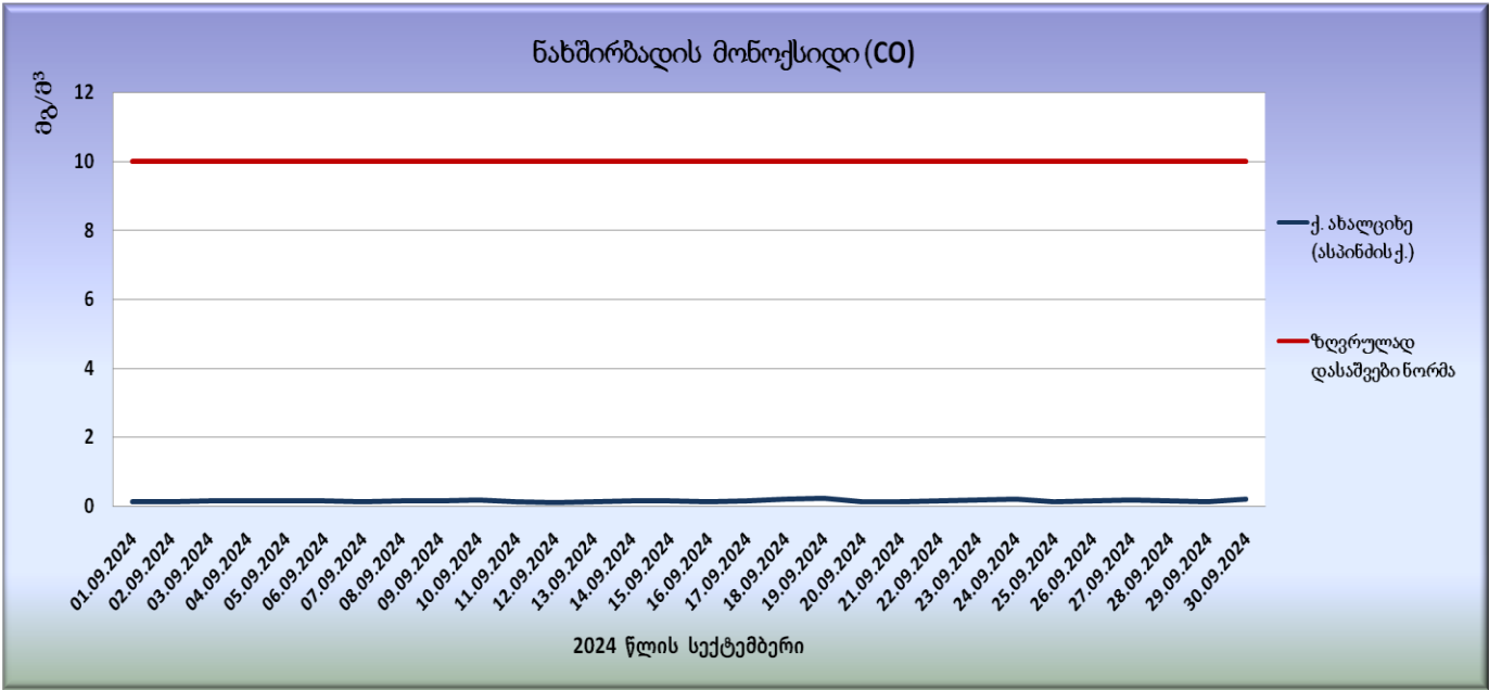
გრაფიკი N24. ნახშირბადის მონოქსიდის (CO) მაქსიმალური ყოველდღიური რეკორდული საშუალო კონცენტრაციები
