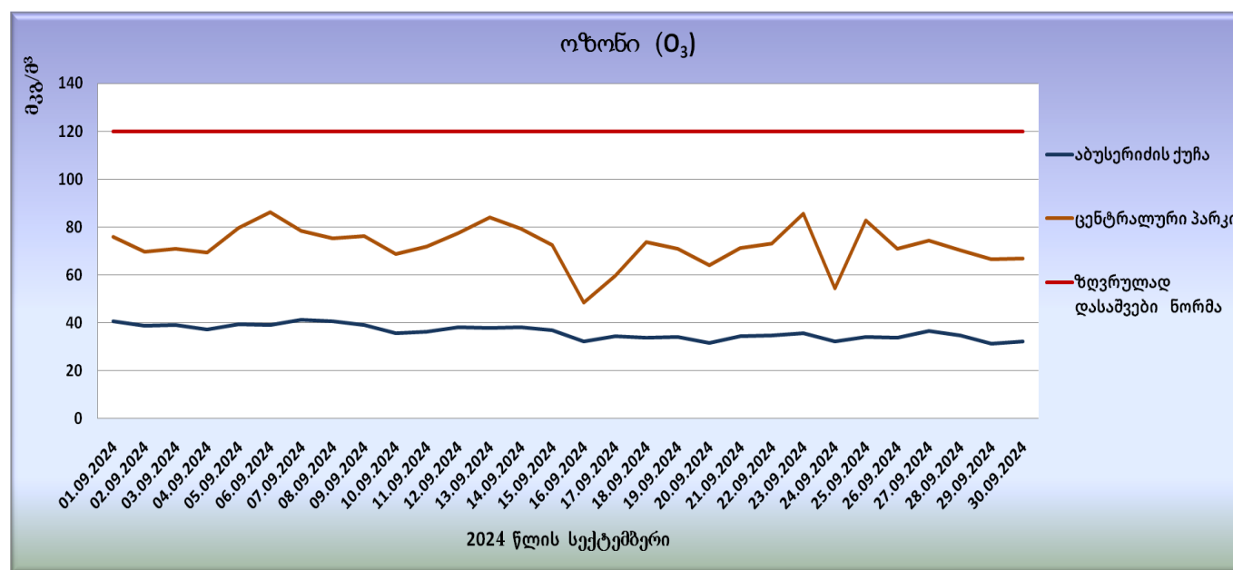
გრაფიკი N9. ოზონის (O 3 ) მაქსიმალური ყოველდღიური რეგისტრირებული საშუალო კონცენტრაციები
