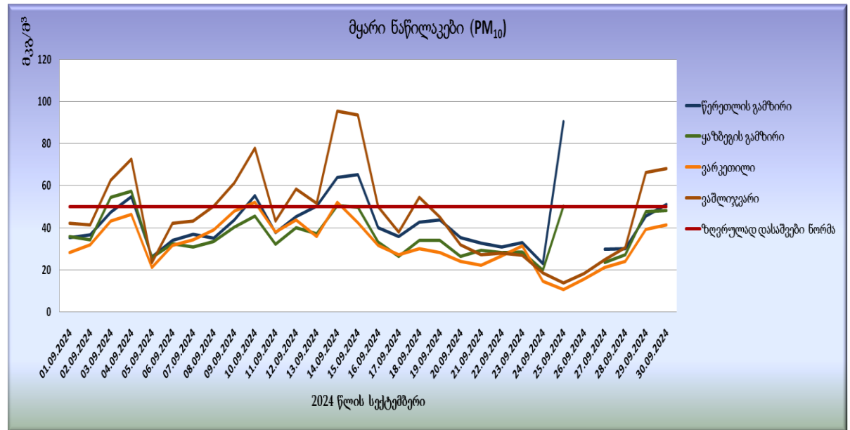
გრაფიკი N2. მყარი ნაწილაკების (PM 10 ) საშუალო საღებრამისო კონცენტრაციები
