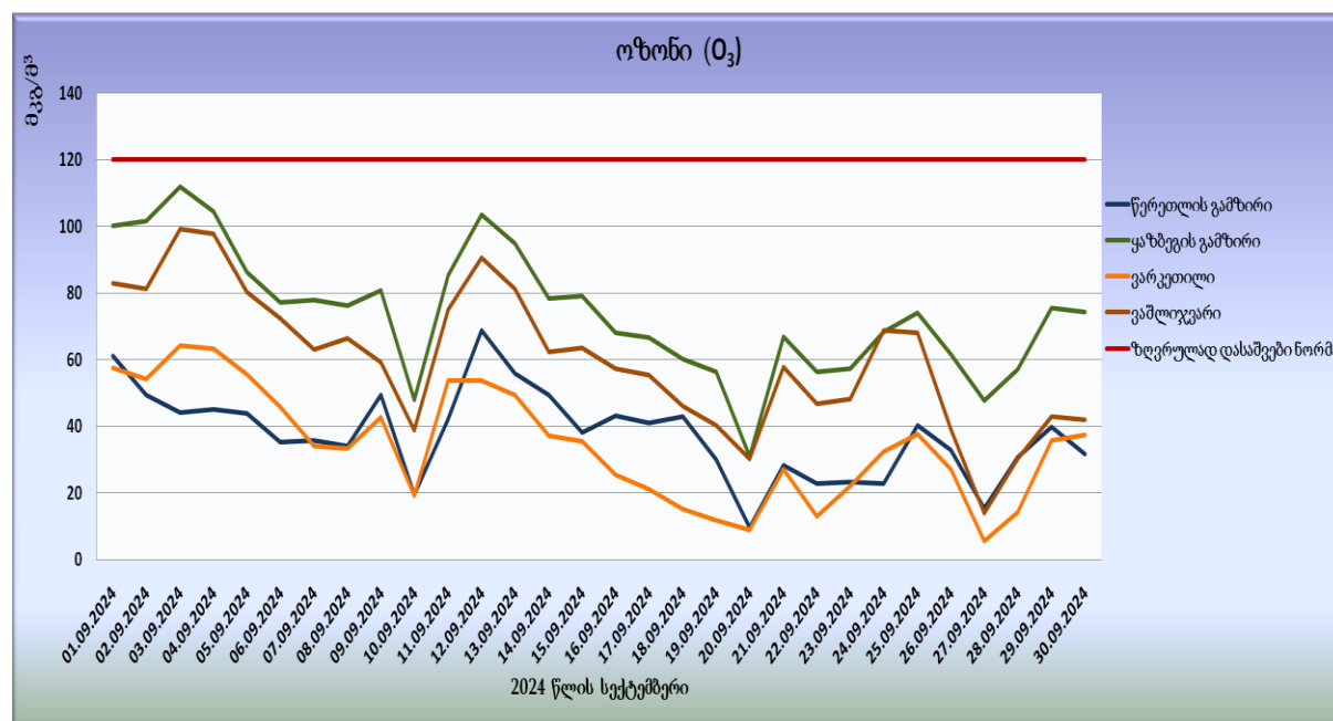
გრაფიკი N4. ოზონის (O 3 ) მაქსიმალური ყოველდღიური რეკორდები საშუალო კონცენტრაციები
