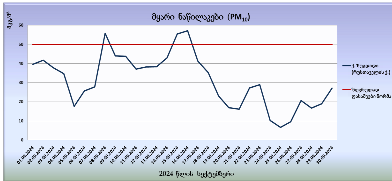
გრაფიკი N26. მყარი ნაწილაკების (PM 10 ) საშუალო სადღეღამისო კონცენტრაციები
