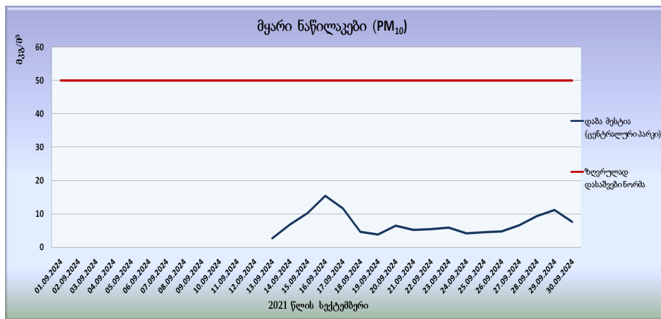
გრაფიკი N32. მყარი ნაწილაკების (PM 10 ) საშუალო სადღეღამისო კონცენტრაციები
