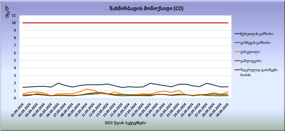
გრაფიკი N5. ნახშირბადის მონოქსიდის (CO) მაქსიმალური ყოველდღიური რეკორდები საშუალო კონცენტრაციები
