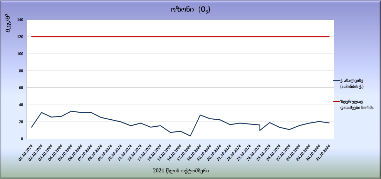
გრაფიკი N22. ოზონის (O 3 ) რეკორდები საშუალო კონცენტრაციები
