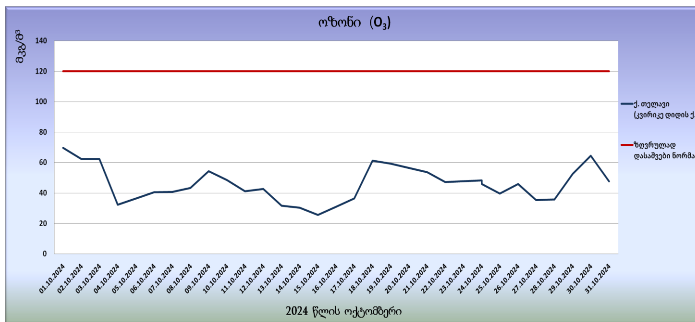
გრაფიკი N31. ოზონის ( O_3 ) მაქსიმალური ყოველდღიური რეკორდული საშუალო კონცენტრაციები
