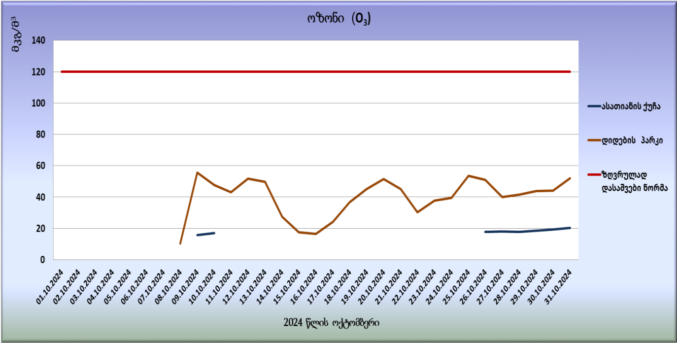
გრაფიკი N17. ოზონის (O 3 ) რეკორდული საშუალო კონცენტრაციები
