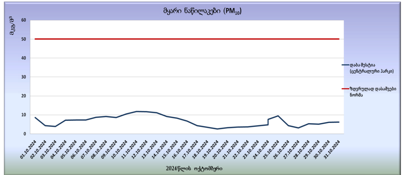
გრაფიკი N32. მყარი ნაწილაკების (PM 10 ) საშუალო სადღეღამისო კონცენტრაციები
