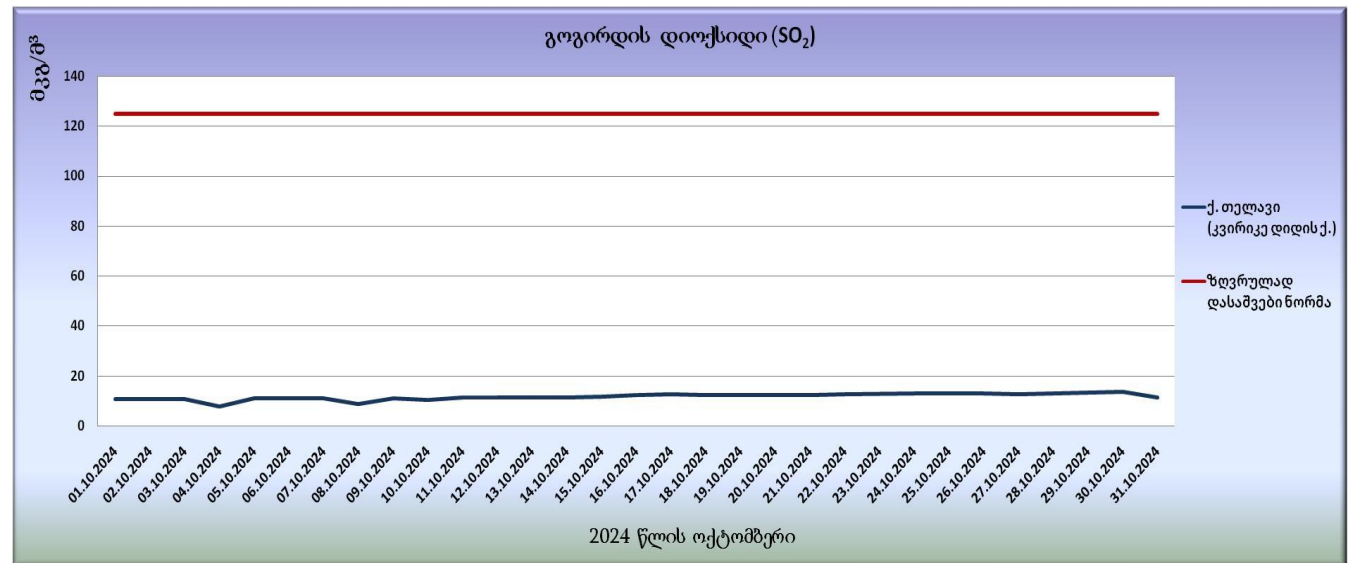
გრაფიკი N28. გოგირდის დიოქსიდის (SO 2 ) საშუალო სადღეღამისო კონცენტრაციები
