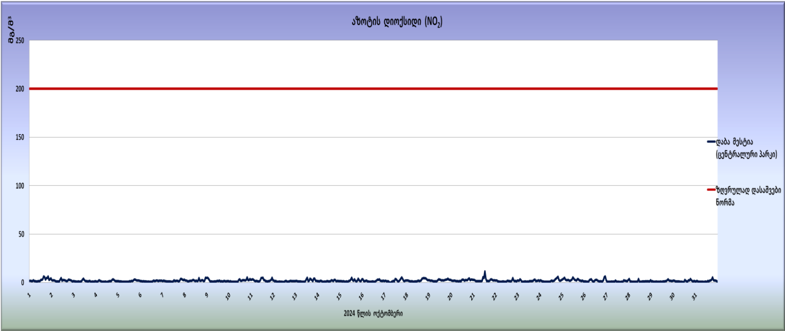
გრაფიკი N33. აზოტის დიოქსიდის (NO 2 ) 1 სთ-იანი გასაშუალოებით მიღებული კონცენტრაციები
