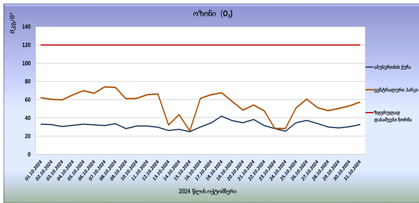
გრაფიკი N9. ოზონის (O 3 ) მაქსიმალური ყოველდღიური რეკორდები საშუალო კონცენტრაციები
