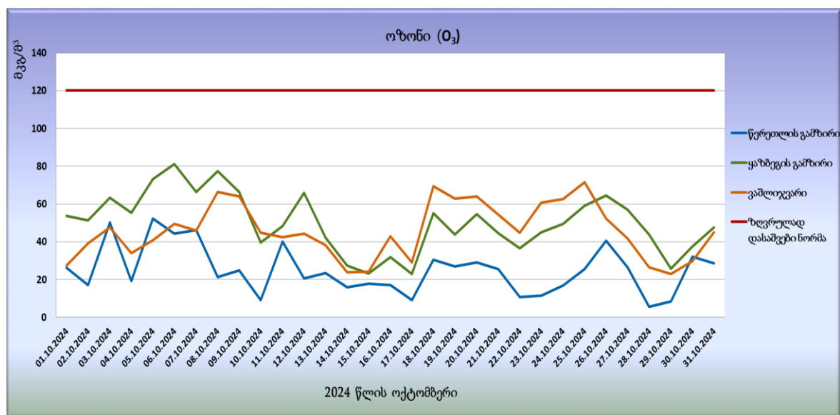
გრაფიკი N4. ოზონის (O 3 ) მაქსიმალური ყოველდღიური რეკორდები
