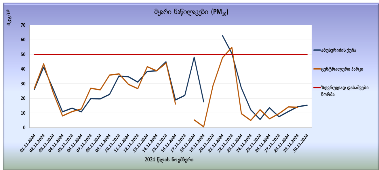
გრაფიკი N7. მყარი ნაწილაკების (PM 10 ) საშუალო საღებუდამისო კონცენტრაციები
