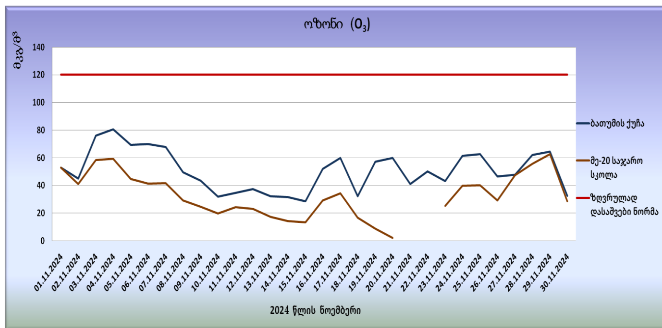
გრაფიკი N14. ოზონის (O 3 ) მაქსიმალური ყოველდღიური რეკონსტრუირებული კონცენტრაციები
