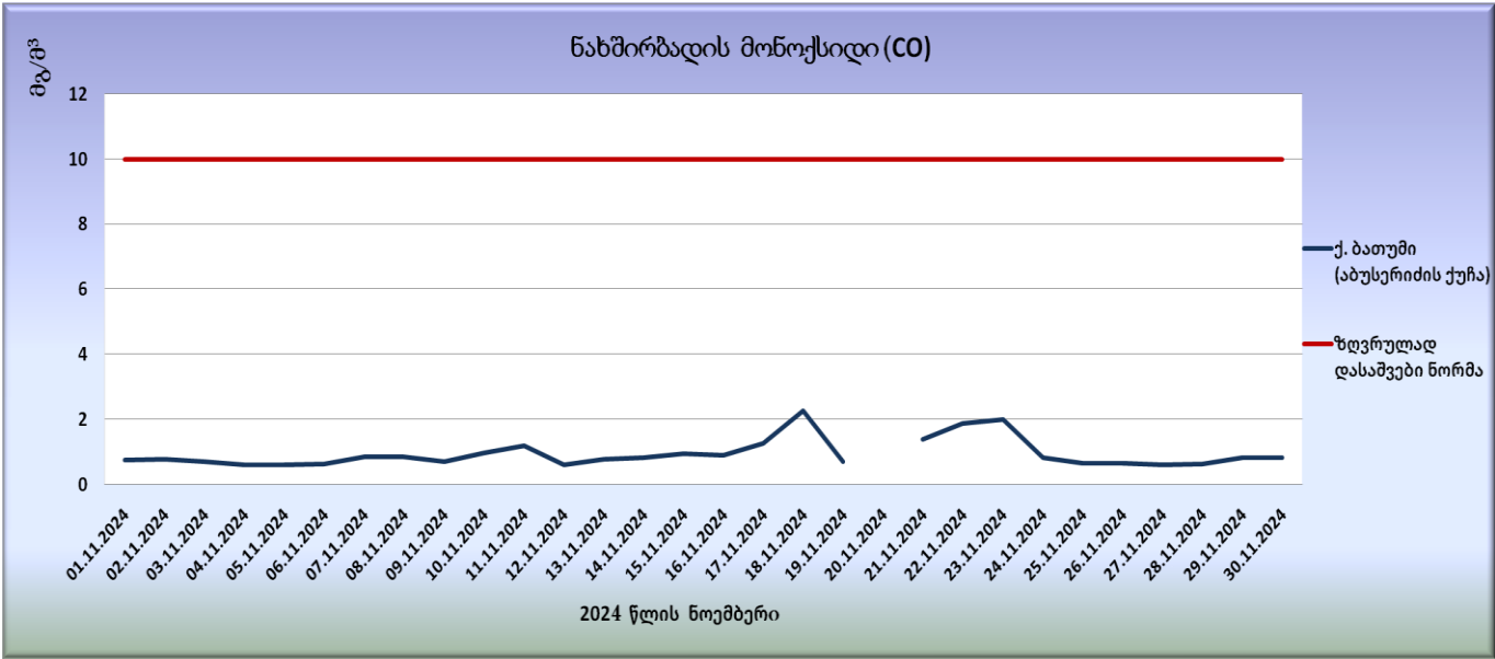
გრაფიკი N10. ნახშირბადის მონოქსიდის (CO) მაქსიმალური ყოველდღიური რვასაათიანი საშუალო კონცენტრაციები
