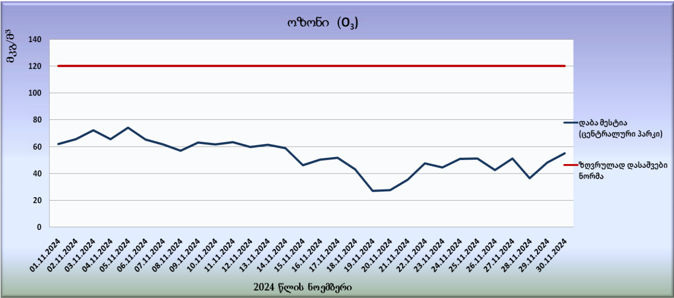
გრაფიკი N34. ოზონის ( O_3 ) მაქსიმალური ყოველდღიური რეკორდები რეკორდები კონცენტრაციები
