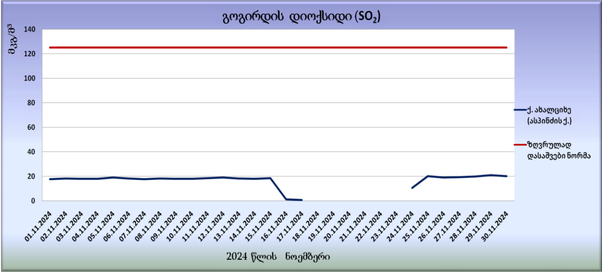
გრაფიკი N20. გოგირდის დიოქსიდის (SO 2 ) საშუალო სადღეღამისო კონცენტრაციები
