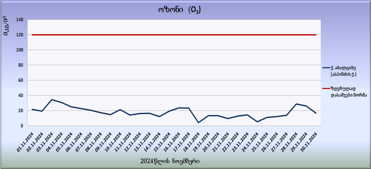
გრაფიკი N22. ოზონის (O 3 ) რეკორდული საშუალო კონცენტრაციები
