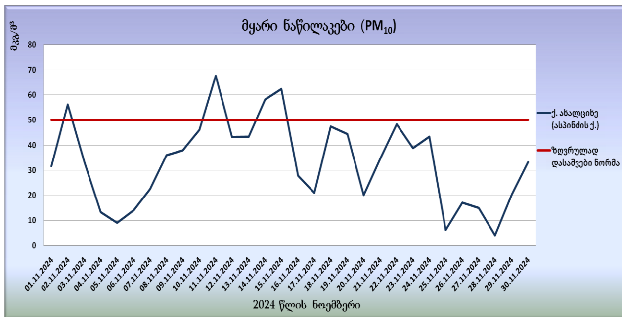
გრაფიკი N21. მყარი ნაწილაკების (PM 10 ) საშუალო სადღეღამისო კონცენტრაციები
