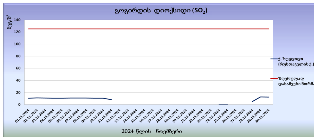
გრაფიკი N25. გოგირდის დიოქსიდის (SO 2 ) საშუალო სადღეღამისო კონცენტრაციები
