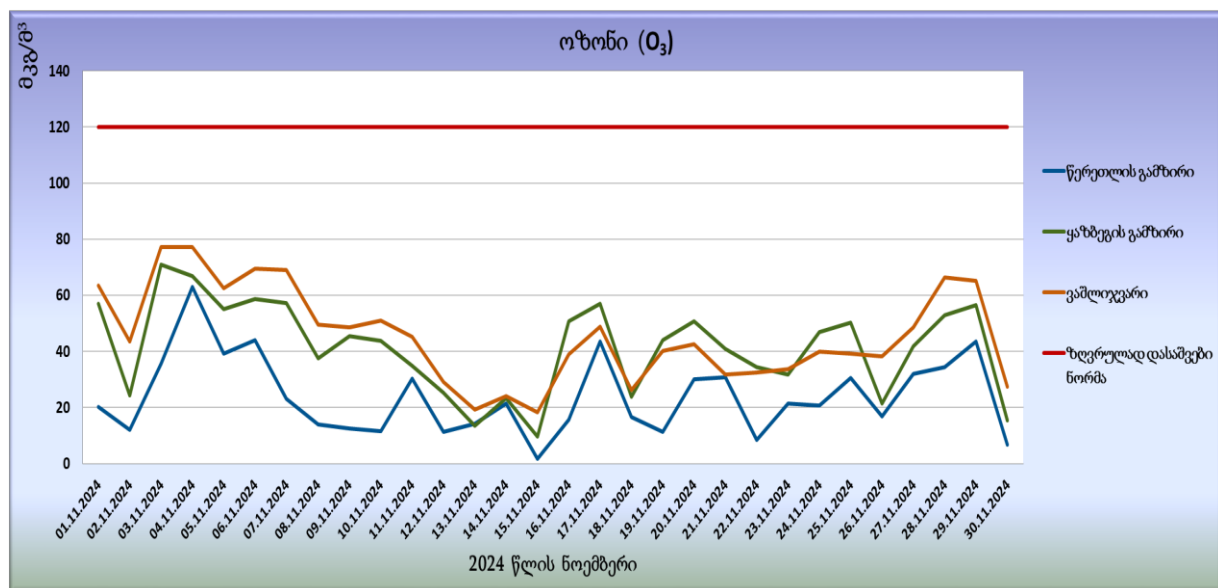
გრაფიკი N4. ოზონის (O 3 ) მაქსიმალური ყოველდღიური რეკორდები
