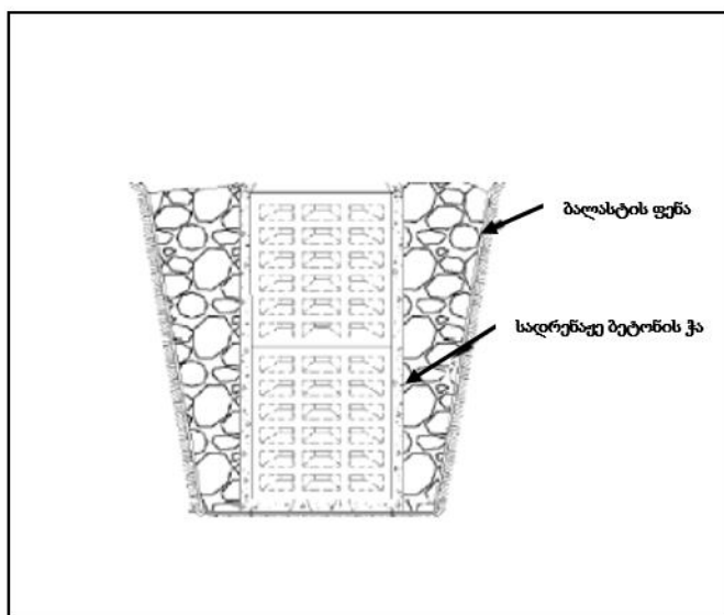
სურათი 6. სადრენაჟე ჭის მოწყობის პრინციპული სქემა
