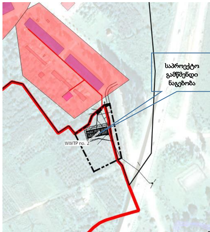
ნახაზი 4.2.5.1 საპროექტო საკანალიზაციო ქსელის არეალი (მონიშნულია ვარდისფრად)
