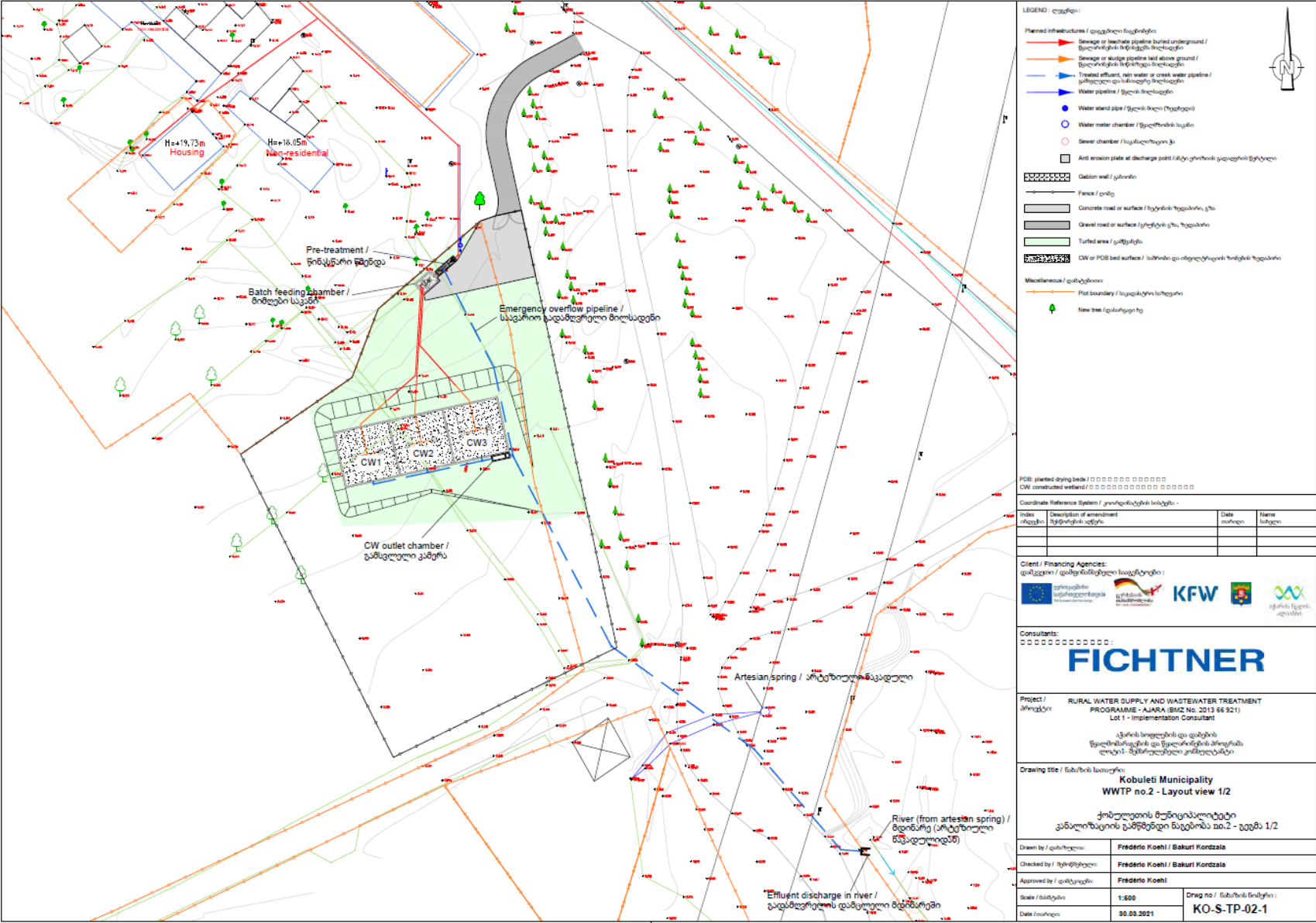
ნახაზი 4.2.4.1 გამწმენდი ნაგებობის გენ-გეგმა
