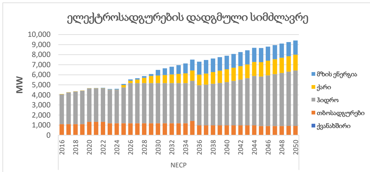
ნახ.3 ელექტროენერჯის გენერაციის სადგურების სიმძლავრის ცვლილება დაგეგმვის პერიოდის განმავლობაში
