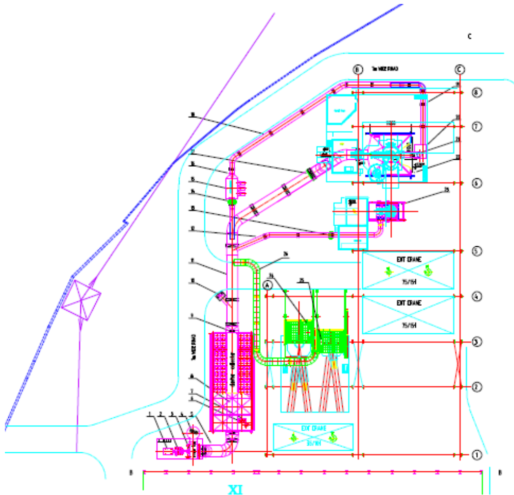
საწარმოს მტვერდამჭერი სისტემის სქემა
