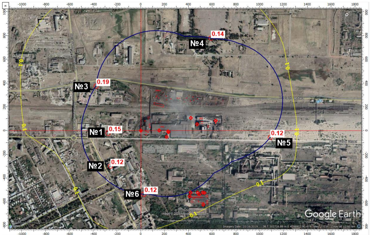
ნივთიერება: 0123 რკინის ტროქსიდი (რკინის ოქსიდი) (რკინაზე გადაანგარიშებით). მაქსიმალური კონცენტრაციები უახლოეს საცხოვრებელ სახლთან (წერტ. N1,2) და ნორმირებულ 500 მ. ზონის საზღვართან (წერტ.3,4,5,6).
