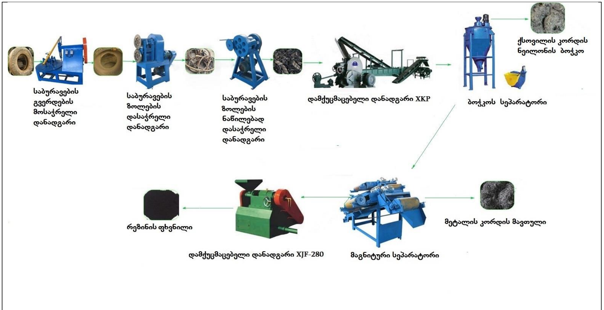
სურათი 4.5.2.7.3. საბურავების გადამუშავების ტექნოლოგიურ პროცესებში გამოყენებული დანადგარების ტიპური ხედი და გადამუშავების პროცესის სქემა
