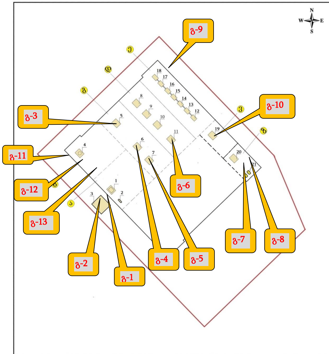
ნახაზი 4.4.1. შ.პ.ს. „რევიკლინგი“-ს საწარმოს გენგეგმა
