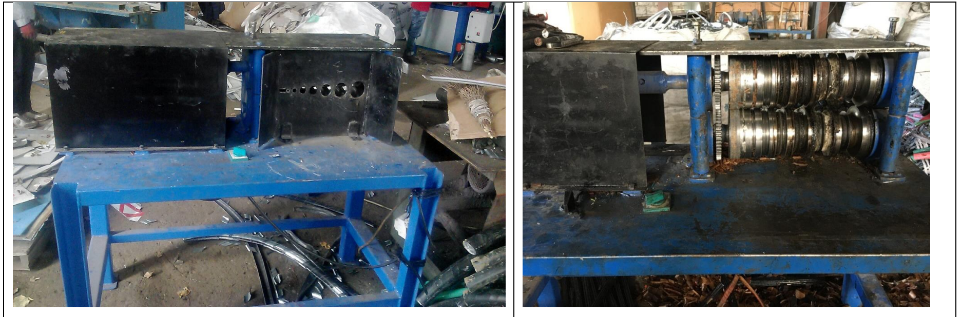
სურათი 4.5.2.8.4. ტექნოლოგიურ პროცესებში გამოყენებული ელექტროკაბელის გასაფცქვნიელი დანადგარი (თვითნაკეთი)
