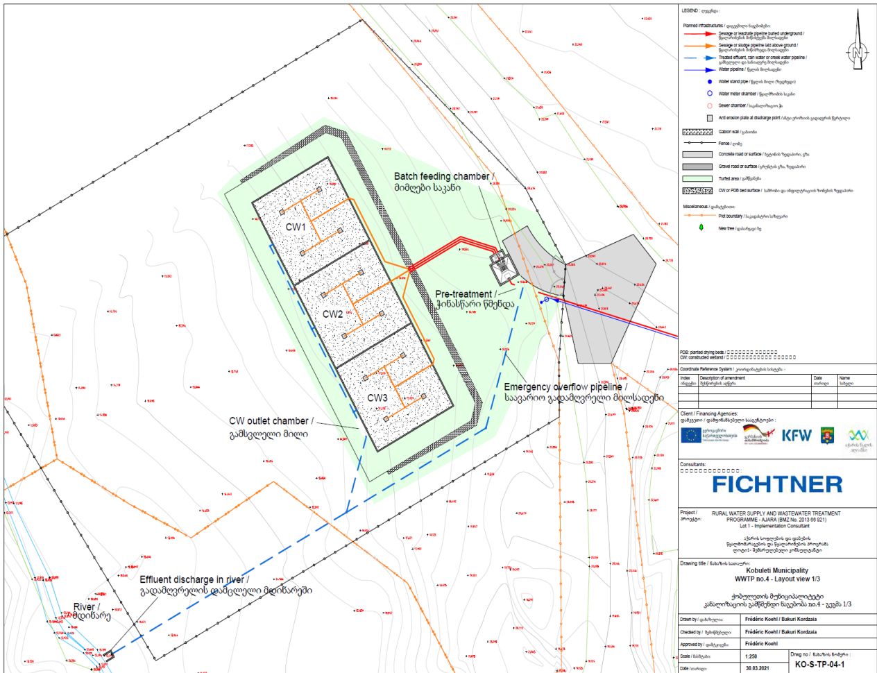
ნახაზი 3.2.4.1. გამწმენდი ნაგებობის გენ-გეგმა
