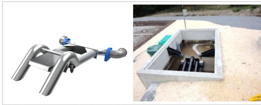
სურათი 3.2.5.1. ავტომატური რეგულირების სიფონი
