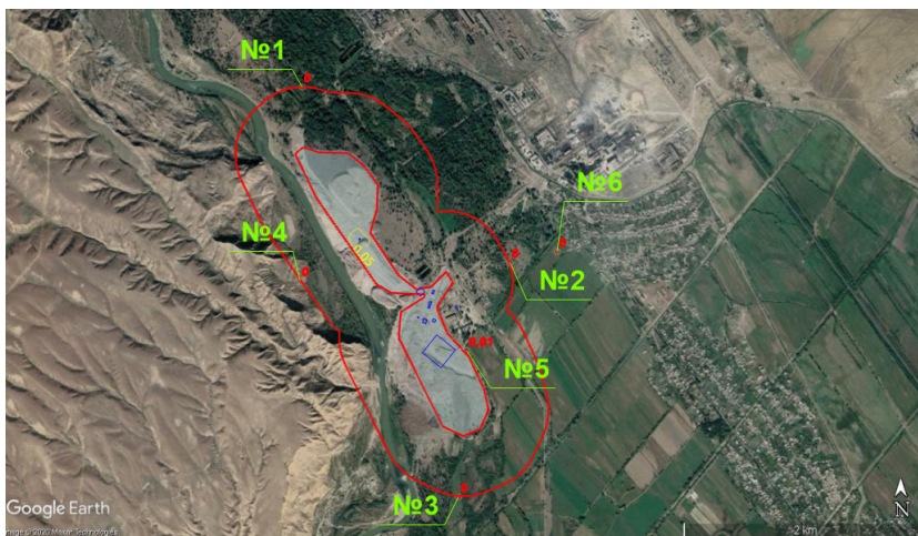
ნახშირბადის ოქსიდის (კოდი 337) მაქსიმალური კონცენტრაციები 500 მ-იანი ზონის საზღვარზე (წერტილები № 1,2,3,4), სასოფლო სამეურნეო სავარგულის საზღვარზე (წერტილი № 5) და უახლოესი დასახლებული ზონის საზღვარზე (წერტილი № 6)
