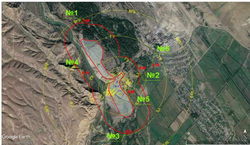
შეწონილი ნაწილაკების (კოდი 2902) მაქსიმალური კონცენტრაციები 500 მ-იანი ზონის საზღვარზე (წერტილები № 1,2,3,4), სასოფლო სამეურნეო სავარგულის საზღვარზე (წერტილი № 5) და უახლოესი დასახლებული ზონის საზღვარზე (წერტილი № 6)
