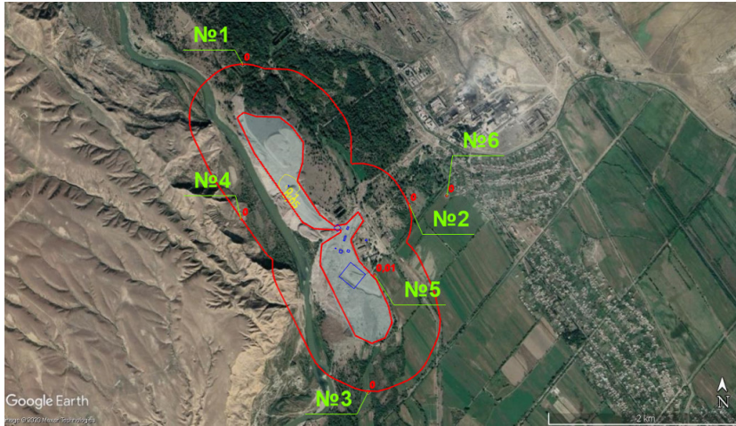
გოგირდის დიოქსიდის (კოდი 330) მაქსიმალური კონცენტრაციები 500 მ-იანი ზონის საზღვარზე (წერტილები № 1,2,3,4), სასოფლო სამეურნეო სავარგულის საზღვარზე (წერტილი № 5) და უახლოესი დასახლებული ზონის საზღვარზე (წერტილი № 6)
