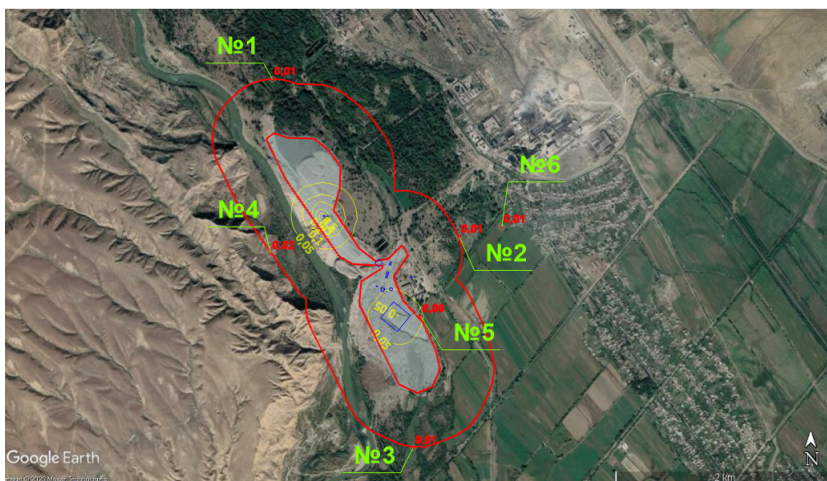
ჭვარტლის (კოდი 328) მაქსიმალური კონცენტრაციები 500 მ-იანი ზონის საზღვარზე (წერტილები № 1,2,3,4), სასოფლო სამეურნეო სავარგულის საზღვარზე (წერტილი № 5) და უახლოესი დასახლებული ზონის საზღვარზე (წერტილი № 6)
