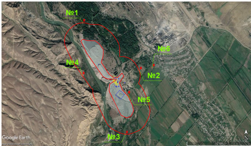
გოგირდწყალბადის (კოდი 333) მაქსიმალური კონცენტრაციები 500 მ-იანი ზონის საზღვარზე (წერტილები № 1,2,3,4), სასოფლო სამეურნეო სავარგულის საზღვარზე (წერტილი № 5) და უახლოესი დასახლებული ზონის საზღვარზე (წერტილი № 6)
