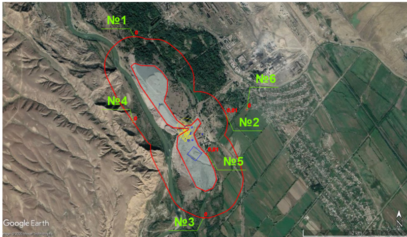
ნაჯერი ნახშირწყალბადების (კოდი 2754) მაქსიმალური კონცენტრაციები 500 მ-იანი ზონის საზღვარზე (წერტილები № 1,2,3,4), სასოფლო სამეურნეო სავარგულის საზღვარზე (წერტილი № 5) და უახლოესი დასახლებული ზონის საზღვარზე (წერტილი № 6)
