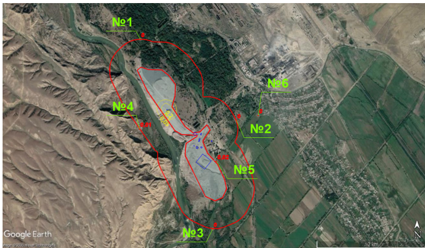
აზოტის ოქსიდის (კოდი 304) მაქსიმალური კონცენტრაციები 500 მ-იანი ზონის საზღვარზე (წერტილები № 1,2,3,4), სასოფლო სამეურნეო სავარგულის საზღვარზე (წერტილი № 5) და უახლოესი დასახლებული ზონის საზღვარზე (წერტილი № 6)
