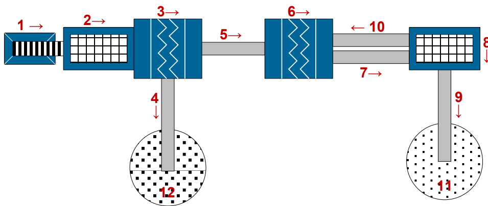
ნახაზი 3.1. სამსხვრევის ტექნოლოგიური სქემა
