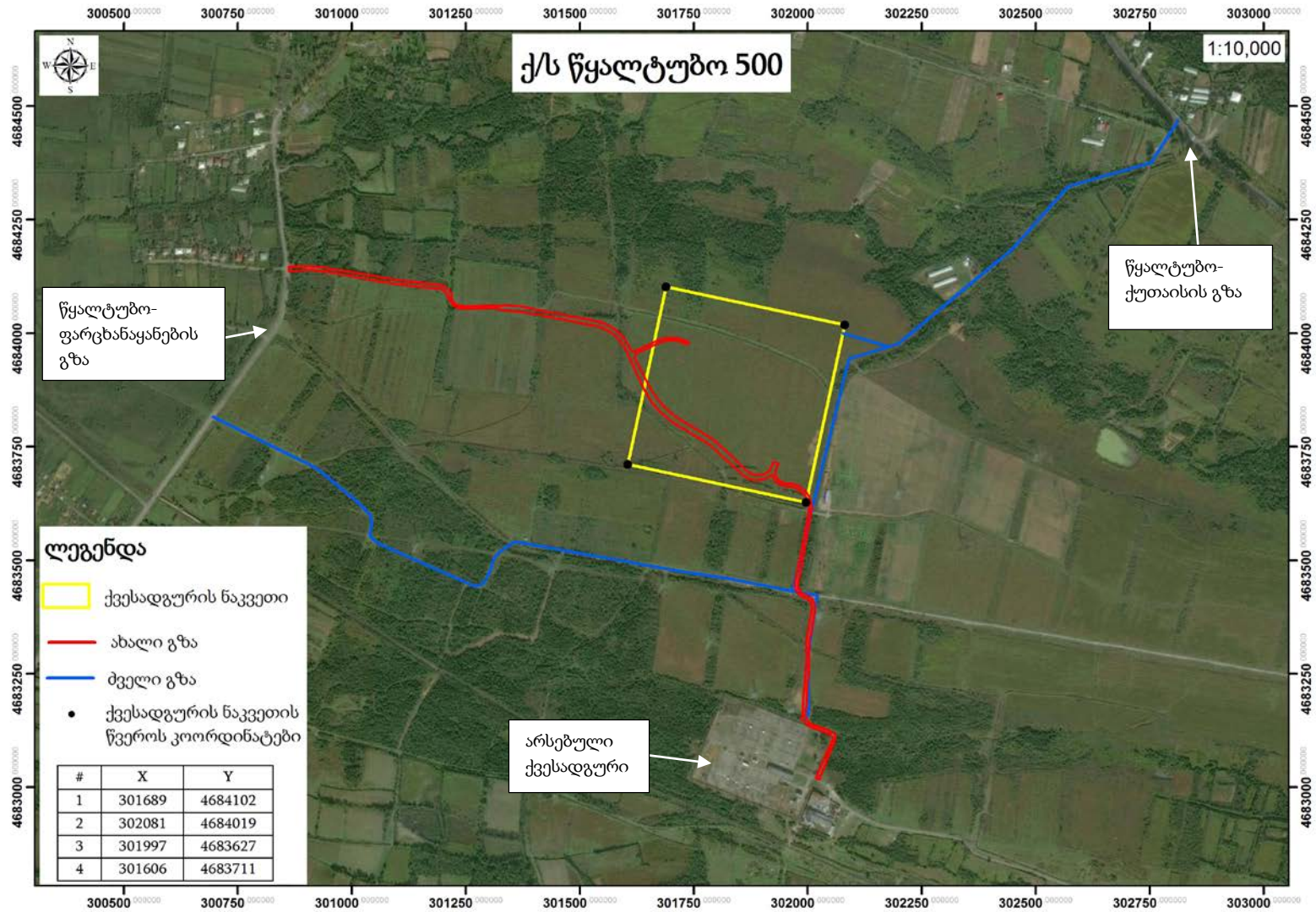
სურათი 2.1. წყალტუბოს 500 კვ ქვესადგურის ტერიტორია მასთან მისასვლელი გზების დატანით
