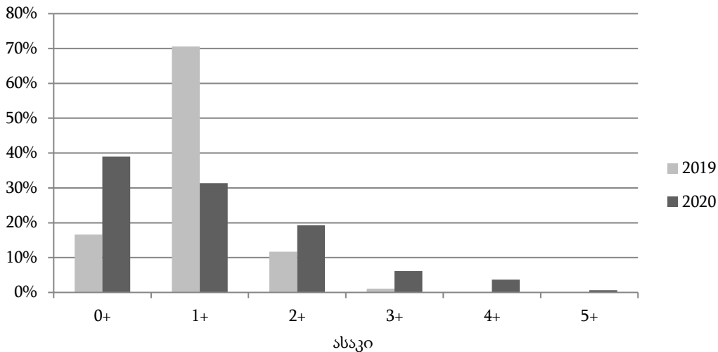
სურ. 21. სტატისტიკა ასაკობრივი სიხშირის გავრცელება, 2019-2020 წწ
