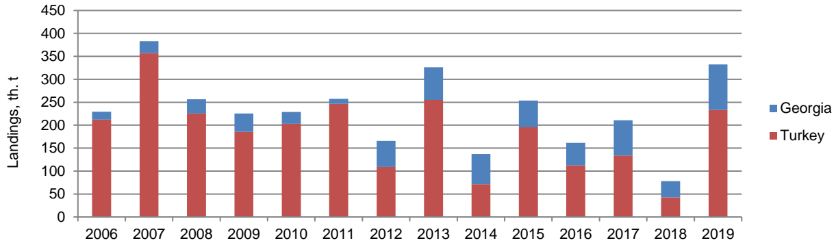
სურ.1 შავი ზღვის ქაფშიას ჭერილი სარეწაო სეზონების მიხედვით.
