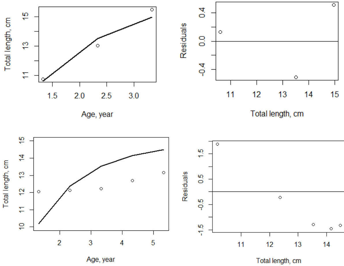
სურ. 25. სტავრიდას ზრდის მრუდი. 2019 წელი (ზედა სქემა), 2020 წელი (ქვედა სქემა).
