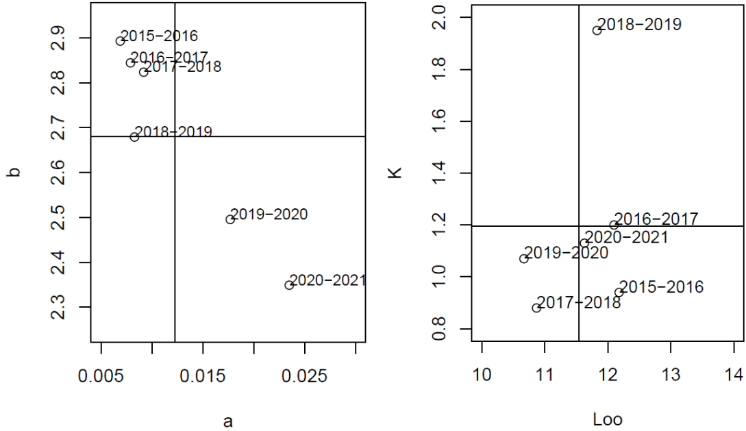
სურ. 7. ქაფშიას ზრდის პარამეტრების საშუალო მნიშვნელობები, 2015-2021.
