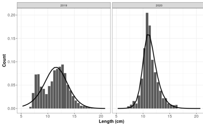
სურ. 38. ხონთქარას სიგრძითი გავრცელება.
