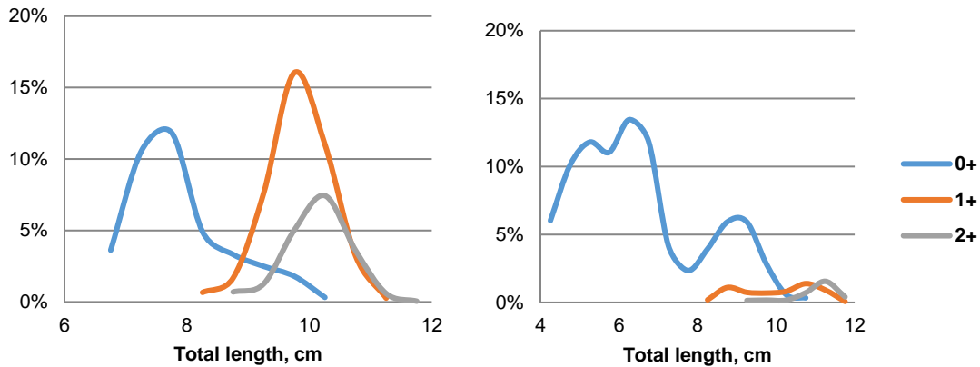
სურ. 19. სიგრძის სიხშირის განაწილება ასაკობრივი ჯგუფების მიხედვით, 2019-2020 (მარცხნივ) და 2020-2021 (მარჯვნივ).
