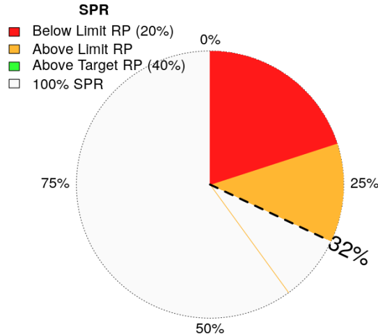
სურ.16. 2018-2019წწ 2019-2020წწ და 2020-2021წწ სეზონების შეფასებული SPR-ის მნიშვნელობა საქართველოს წყლებში.
