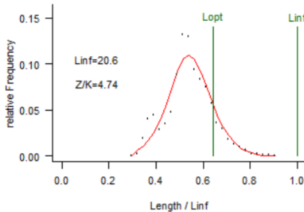
სურ. 35. ხონთქარას სიგრძითი გავრცელება დროის მონაკვეთში .
