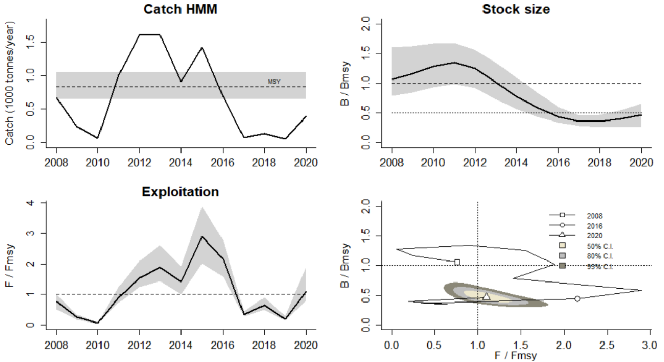
სურ.28. სტავრიდას CMSY ანალიზის შედეგები საქართველოს წყლებში
