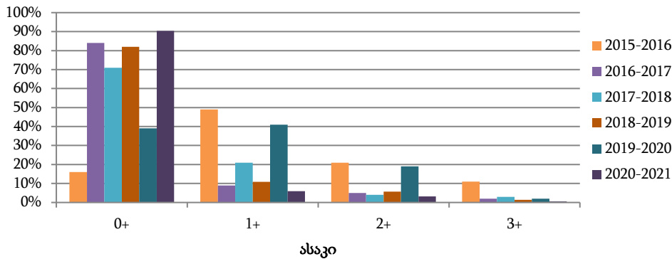
სურ. 3. საქართველოს წყლებში ქაფშიას ასაკობრივი სიხშირის განაწილება.
