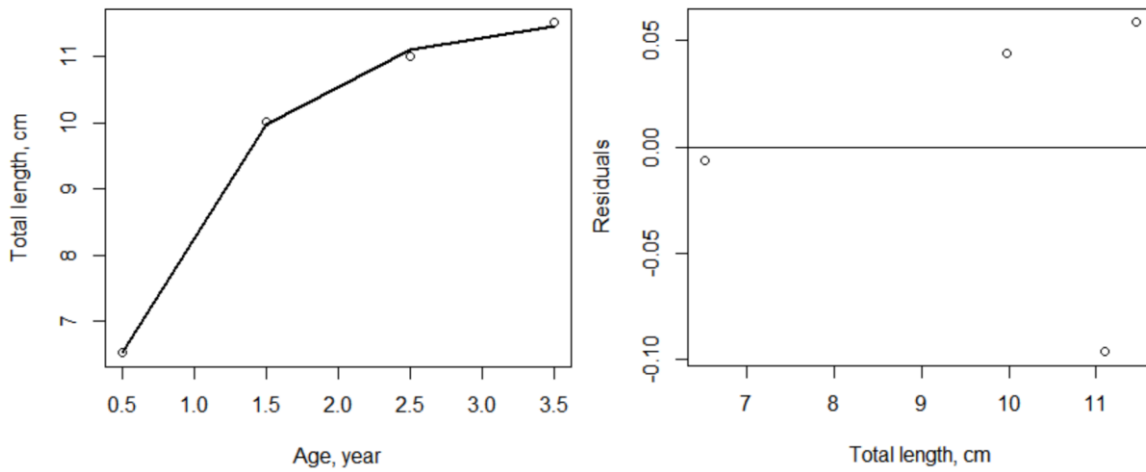
სურ.13. ქაფშიას ზრდის მრუდი, 2020-2021.
