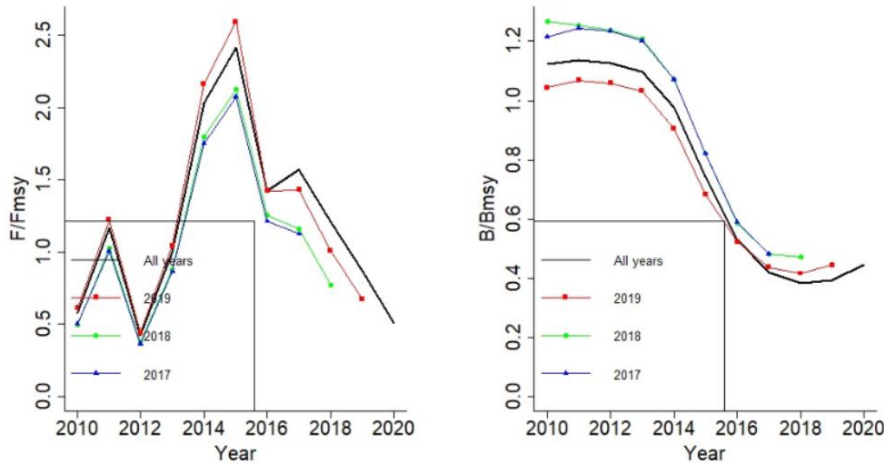
სურ.39. ხონთქარას რეტროსპექტული ანალიზი CMSY მოდელის შესაბამისად.
