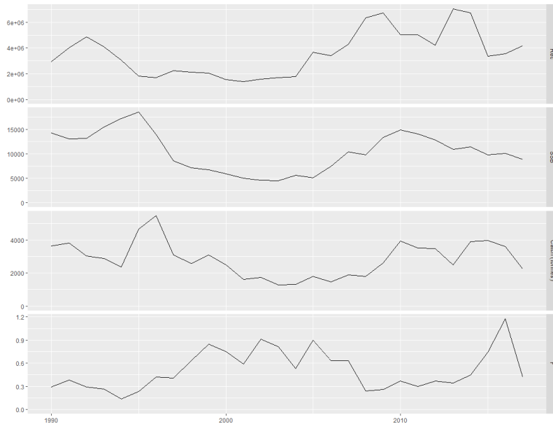
სურ.33. ხონტქარას ჭერილები, სატოფო მარაგის ბიომასა, სარეწაო სიკვდილიანობის მაჩვენებელი და ახალმოზარდების ს რაოდენობა მთელ შავ ზღვაში, 1989-2017
