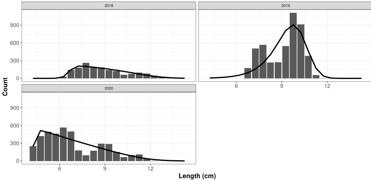
სურათი 18. . ქაფშიის სიგრძითი გავრცელების შესაბამისობა.
