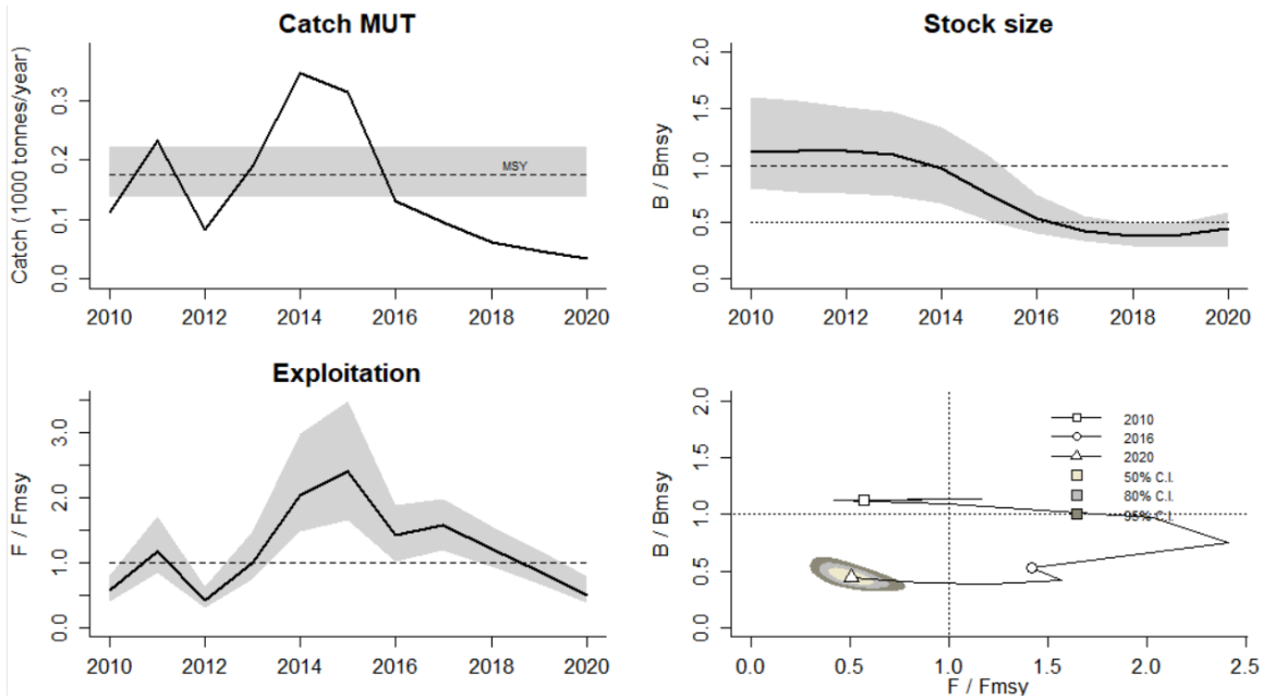
სურ. 37. ხონთქარას CMSY ანალიზის შედეგები საქართველოს წყლებში
