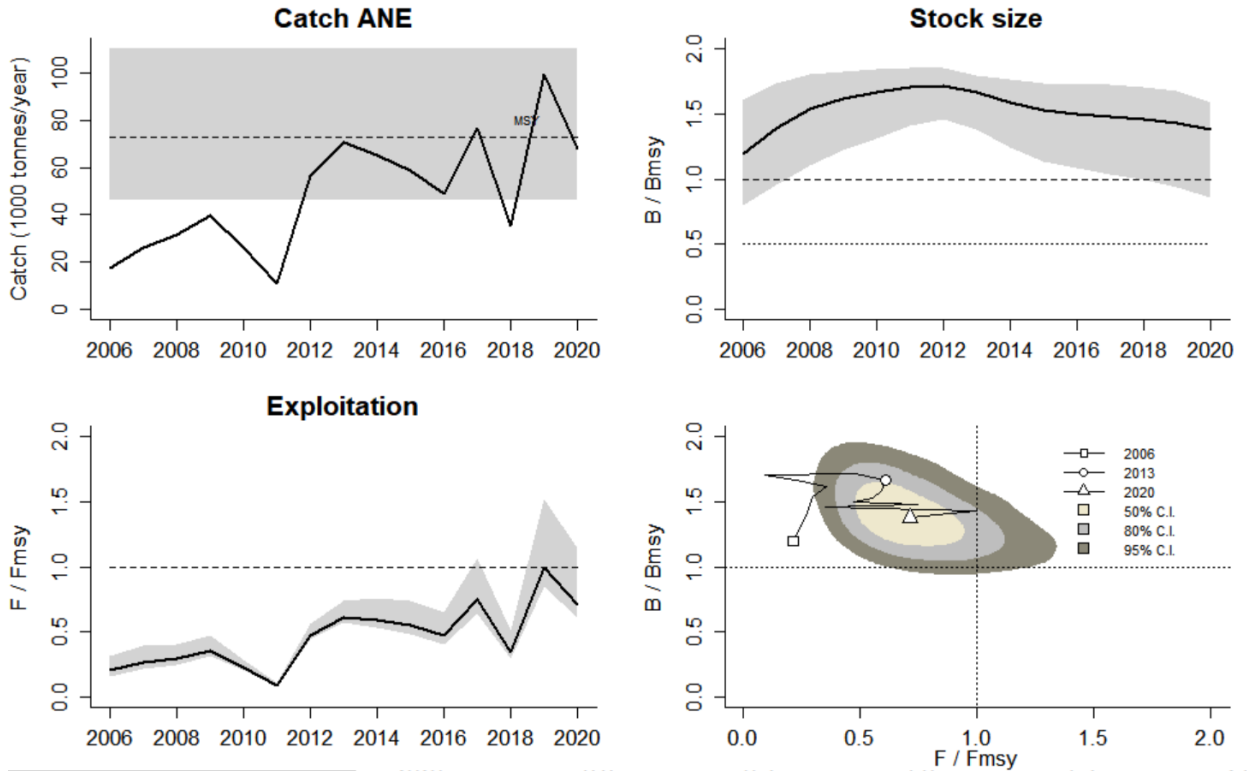
სურ. 17. CMSY ანალიზის შედეგები შავი ზღვის ქაფშიაზე საქართველოს წყლებში.
