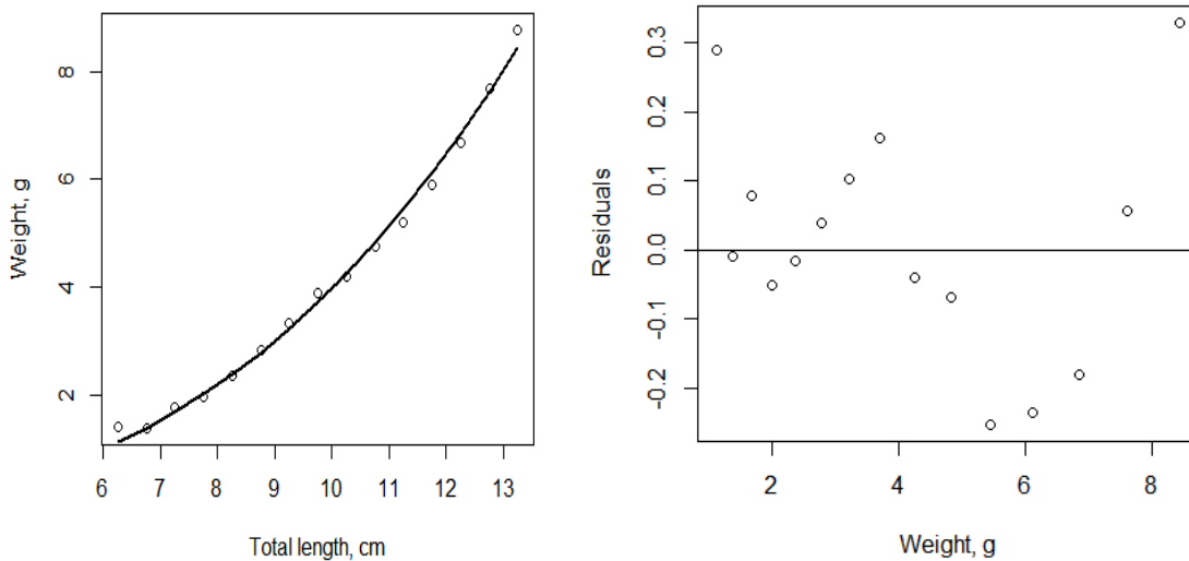
სურ. 8. ქაფშიას სიგრძისა და წონის ურთიერთდამოკიდებულება, 2018-2019.
