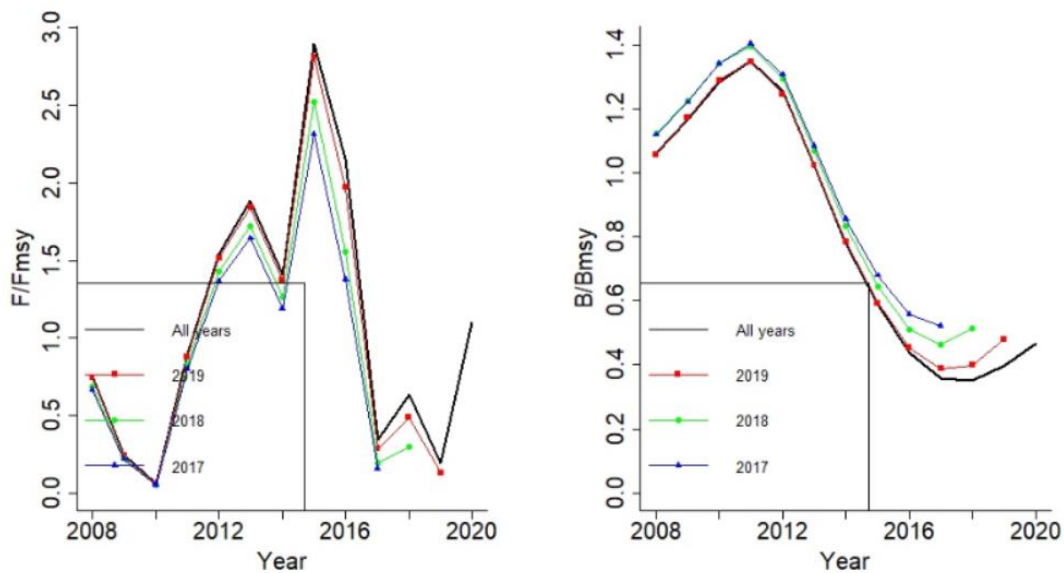
სურ. 30. სტავრიდას რეტროსპექტული ანალიზი CMSY მოდელის შესაბამისად
