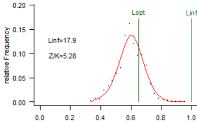
სურ 26. სტავრიდას სიგრძითი გავრცელება დროის მონაკვეთში, დეკემბერი 2019-2020
