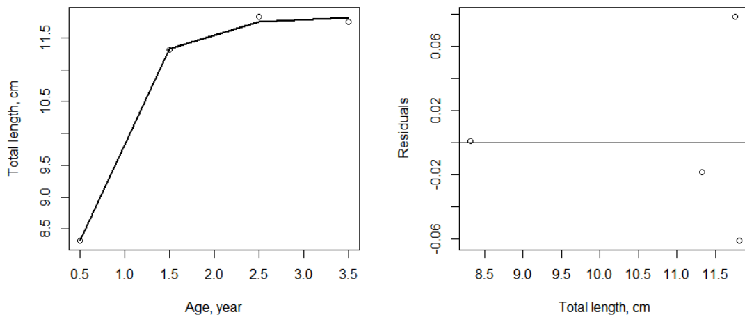
სურ.11. ქავშიას ზრდის მრუდი, 2018-2019.
