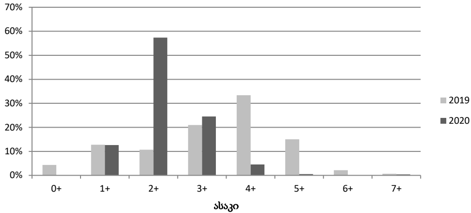
სურ. 31. ხონთქარას ასაკობრივი-სიხშირის გავრცელება
