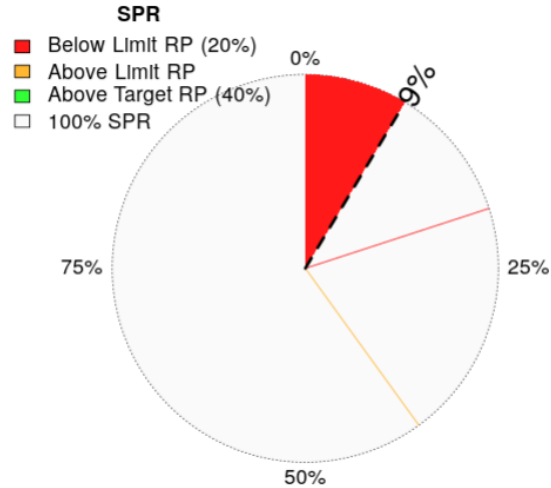
სურ. 27. საქართველოს წყლებში სტავრიდას SPR შეფასება, 2020წ.
