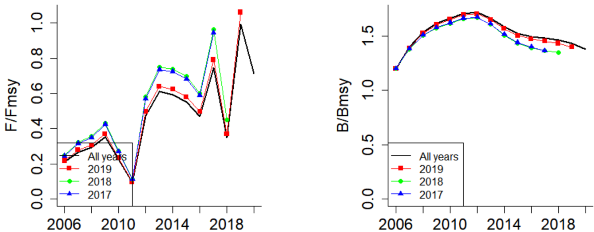
სურ.20. CMSY მოდელის რეტროსპექტული ანალიზი შავი ზღვის ქაფშიასთვის.
