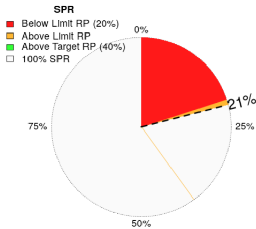
სურ. 36. საქართველოს წყლებში ხონთქარას SPR შეფასება.
