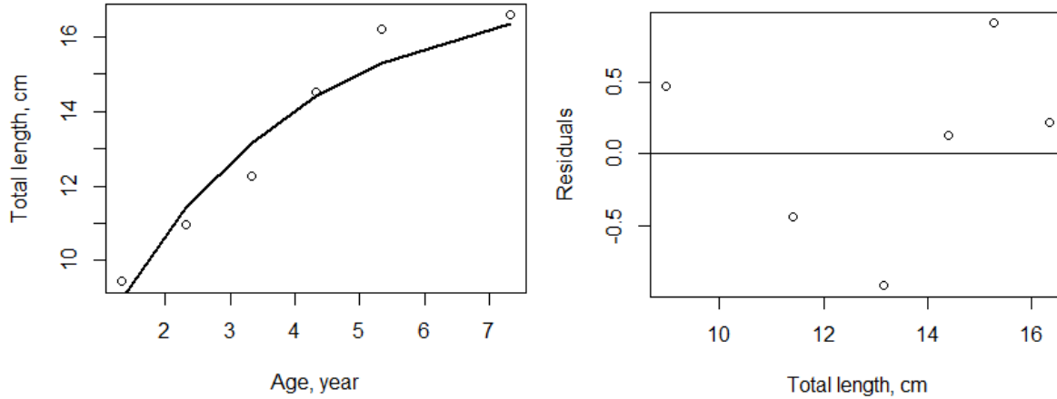
სურ. 35. ხონთქარას ზრდის მრუდი. ზედა სქემა 2019 წლის მონაცემით. ქვედა სქემა 2020 წლის მონაცემით
