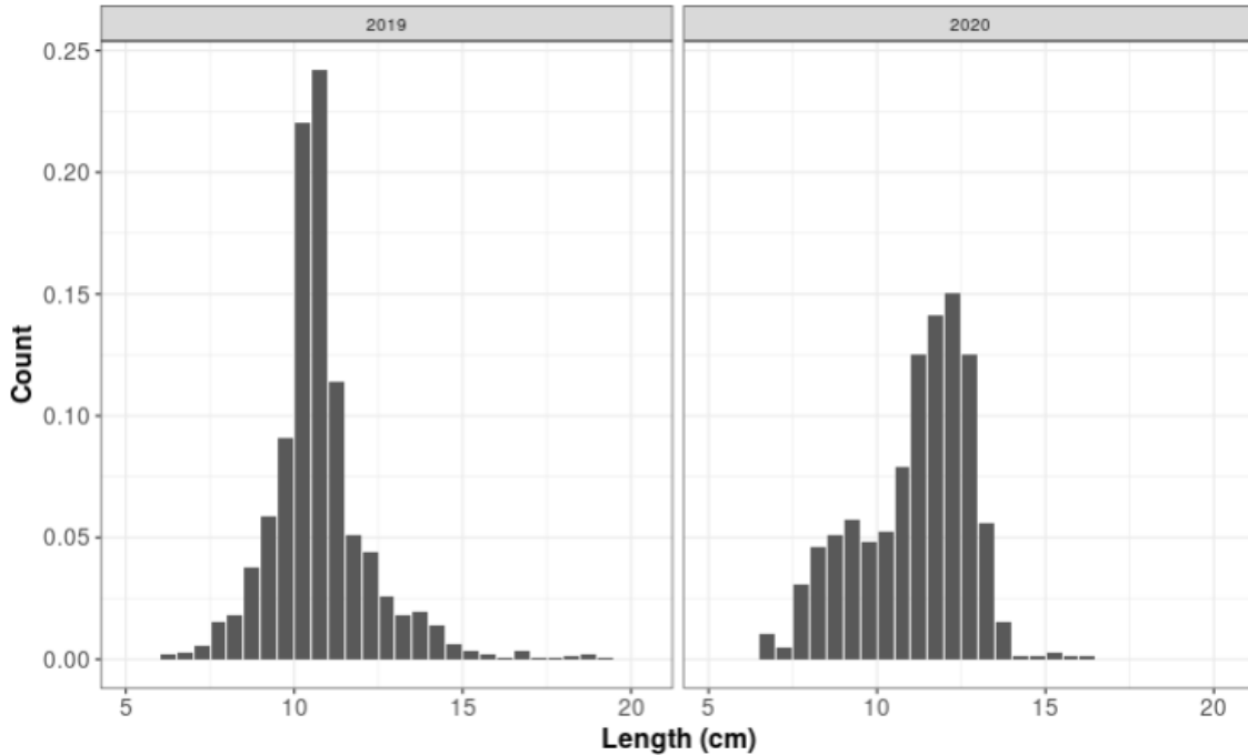
სურ.22 სტავრიდას სიგრძითი გავრცელება საქართველოს წყლებში, 2019-2020 წწ
