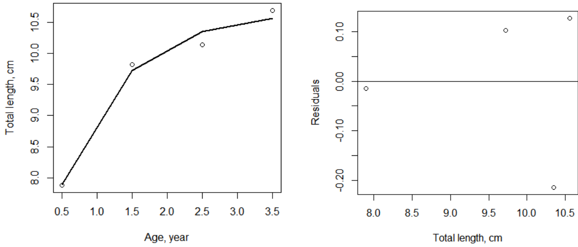
სურ.12. ქაფშიას ზრდის მრუდი, 2019-2020
