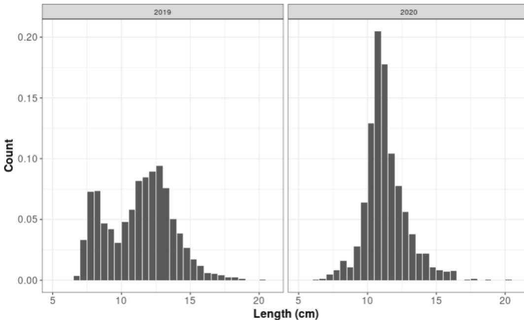
სურ. 32. ხონთქარას სიგრძითი გავრცელება.
