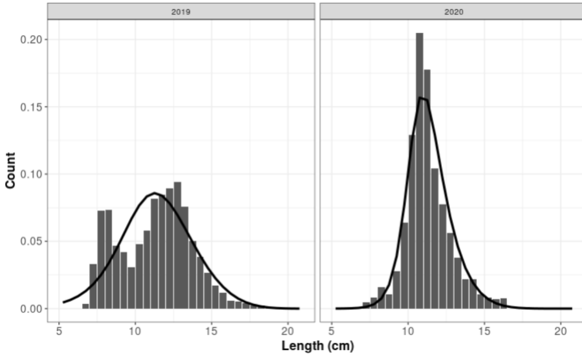
სურ.29. სტავრიდას სიგრძითი გავრცელება, დეკემბერი 2019-2020
