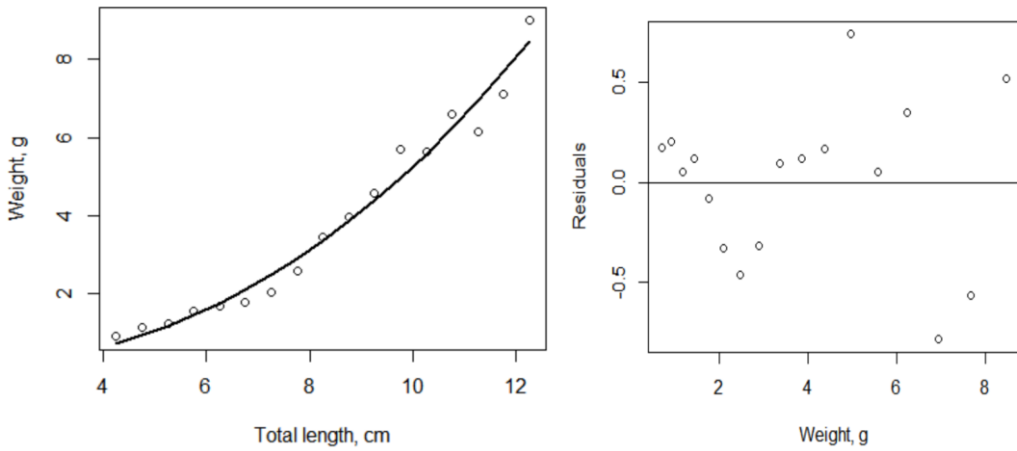
სურ.10. ქავშიას ზომა-წონითი ურთიერთდამოკიდებულება 2020-2021.
