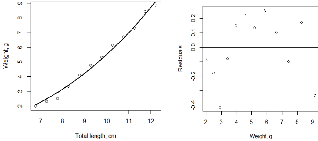
სურ.9. ქავშიას ზომა-წონითი ურთიერთდამოკიდებულება, 2019-2020.
