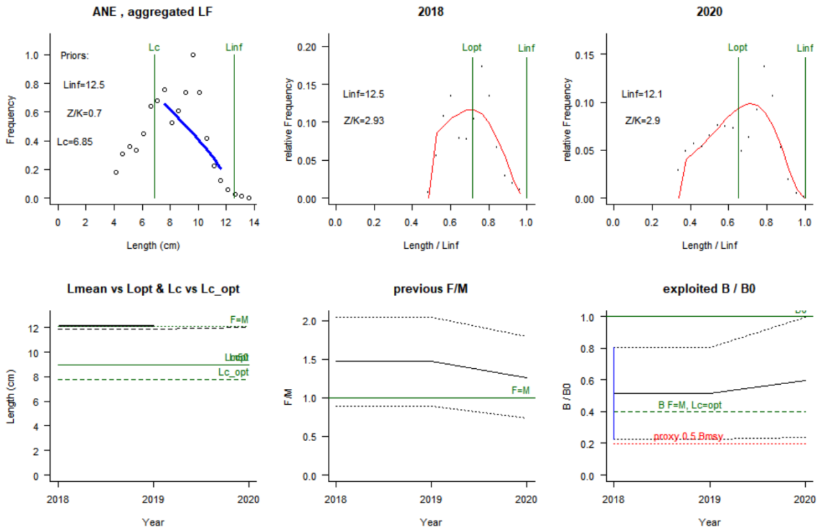
სურ. 15. შავი ზღვის ქაფშიას LBB ანალიზის შედეგები საქართველოს წყლებში.
