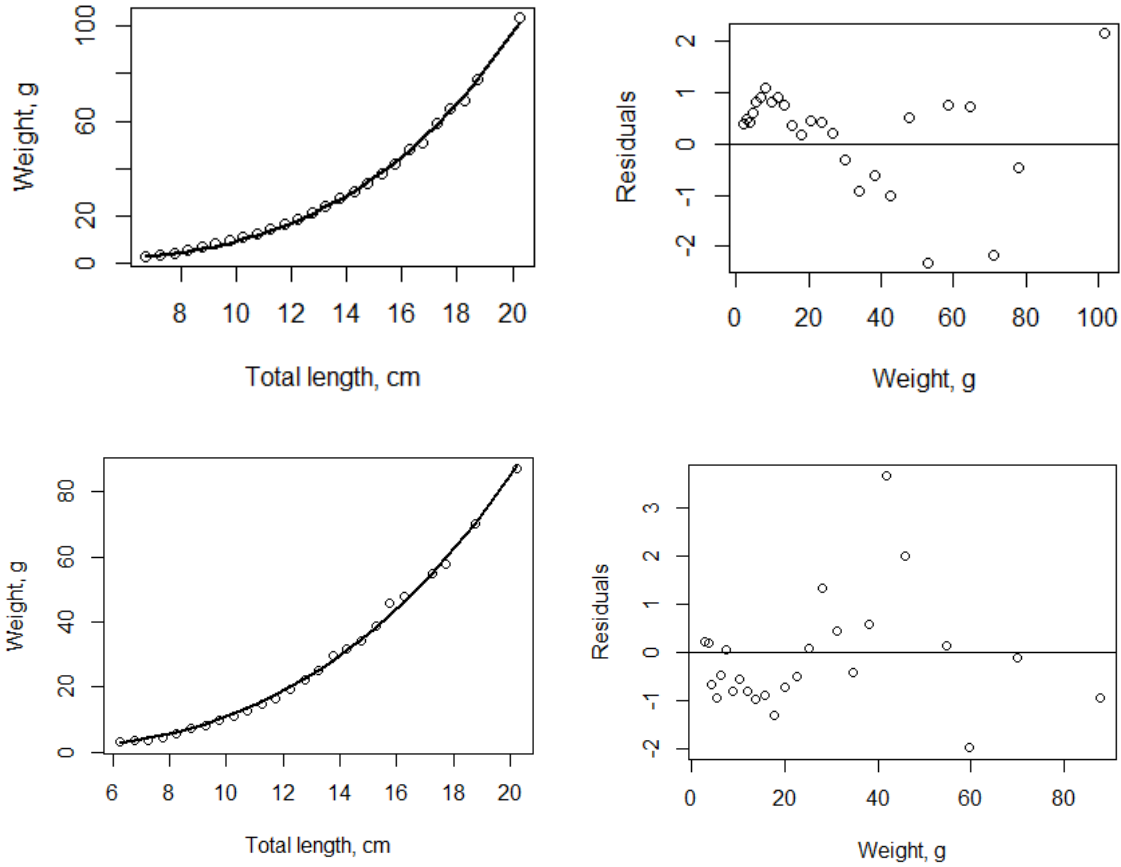
სურ. 34. ხონთქარას სიგრძისა და წონის თანაფარდობა. ზედა სქემა 2019 წლის მონაცემით. ქვედა სქემა 2020 წლის მონაცემით
