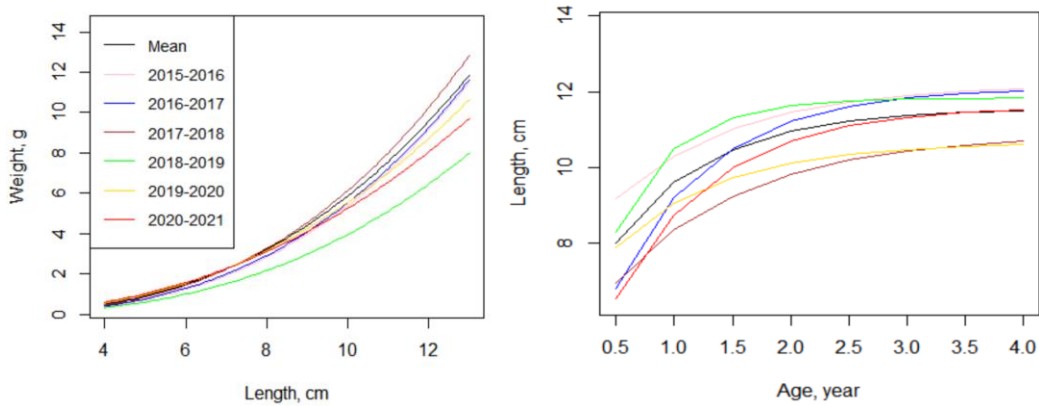
სურ.14 ქაფშიას სიგრძე-წონითი ურთიერთდამოკიდებულება და ზრდის მრუდი.
