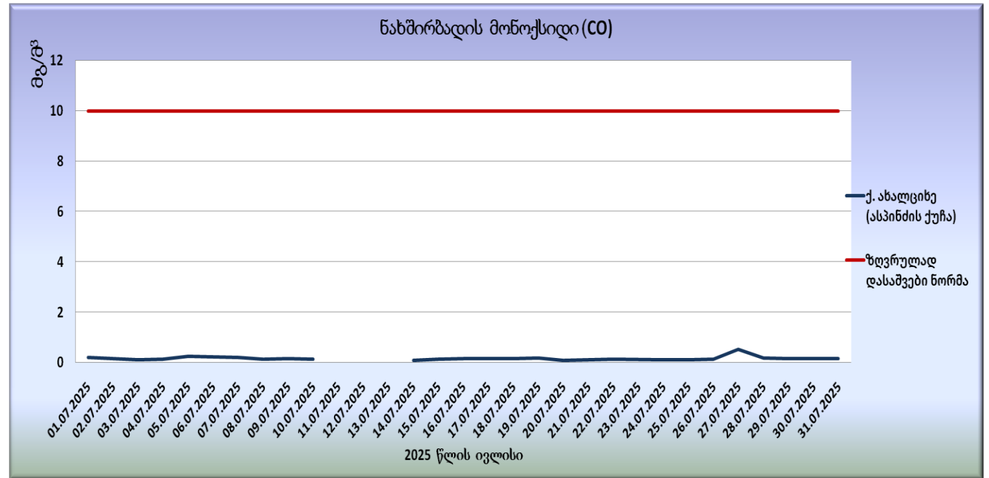
გრფუკი N23. ნახშირბადის მონოქსიდის (CO) ყოველდღიური რეგისტრაციის მაქსიმალური საშუალო კონცენტრაციები
