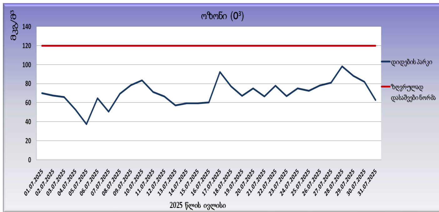
გრაფიკი N17. ოზონის ( O_3 ) ყოველდღიური რეასაათანი მაქსიმალური საშუალო კონცენტრაციები
