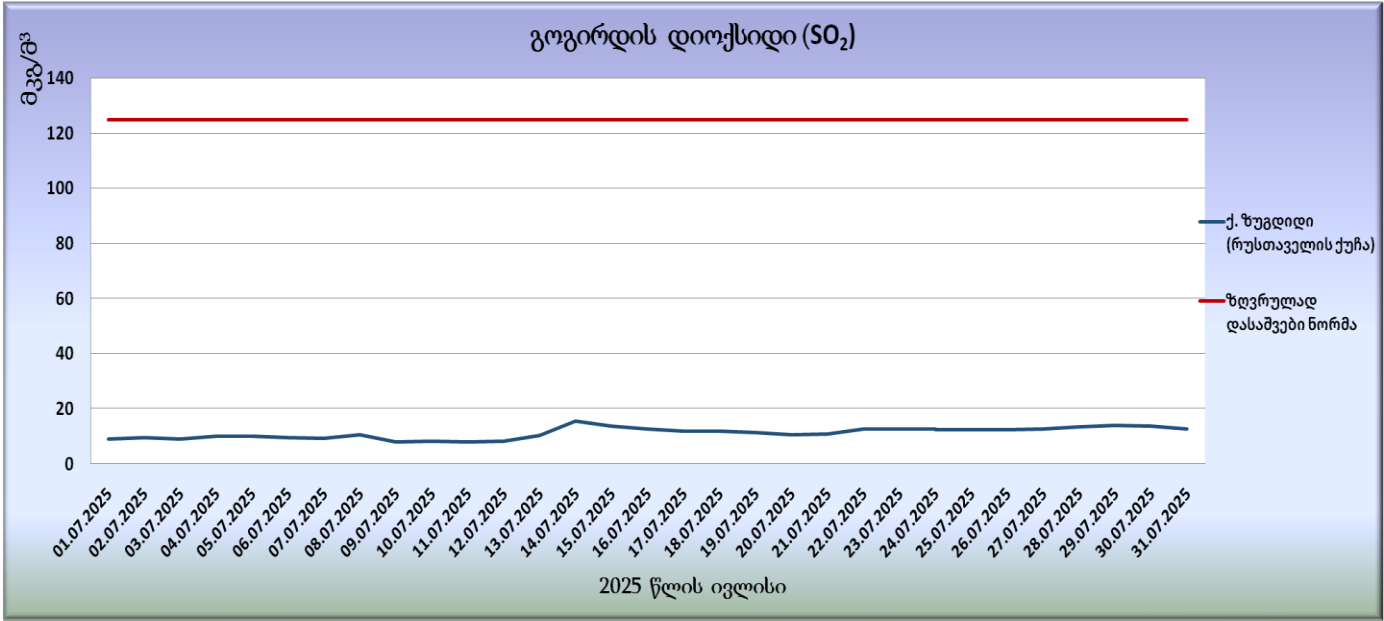
გრაფიკი N24. გოგირდის დიოქსიდის (SO 2 ) საშუალო დღეისო კონცენტრაციები
