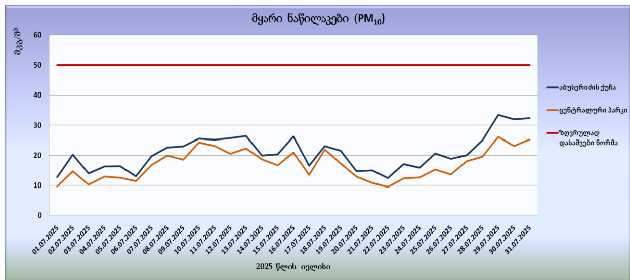
გრაფიკი N7. მყარი ნაწილაკების (PM 10 ) საშუალო დღედი მონიტორინგის ცენტრები
