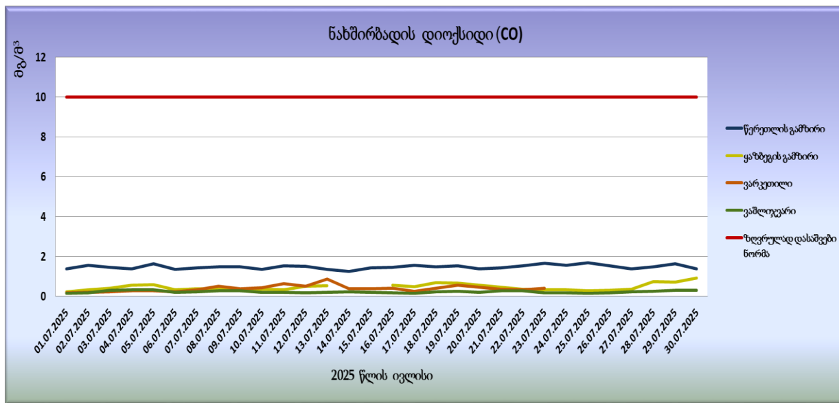
გრაფიკი N5. ნახშირბადის მონოქსიდის (CO) ყოველდღიური რეგსაათიანი მაქსიმალური საშუალო კონცენტრაციები
