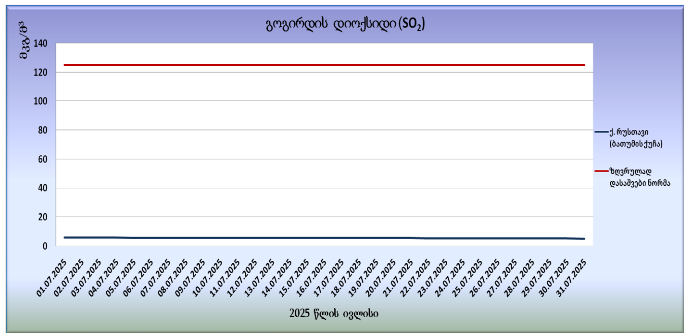
გრფიკი N11. გოგირდის დიოქსიდის (SO 2 ) საშუალო დღეობის კონცენტრაციები
