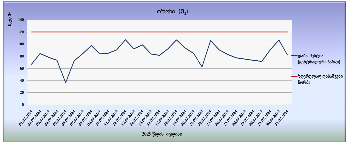
გრფიკი N34. ოზონის (O 3 ) ყოველდღიური რეგისტრირებული მაქსიმალური საშუალო კონცენტრაციები
