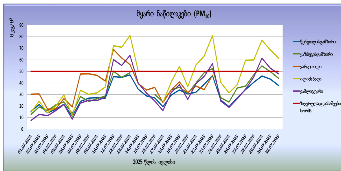
გრფუკი N2. მყარი ნაწილაკების (PM 10 ) საშუალო საღებულისოკონცენტრაციები
