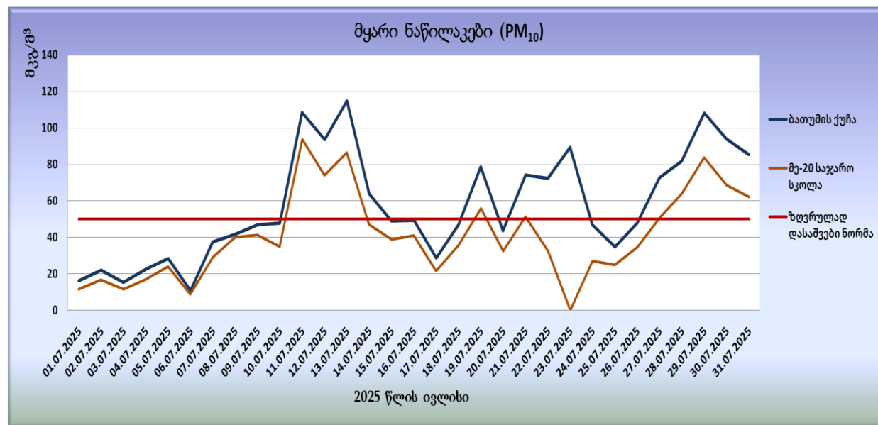
გრაფიკი N12. მყარი ნაწილაკების ( PM_{10} ) საშუალო დღე-ღამის საშუალო კონცენტრაციები
