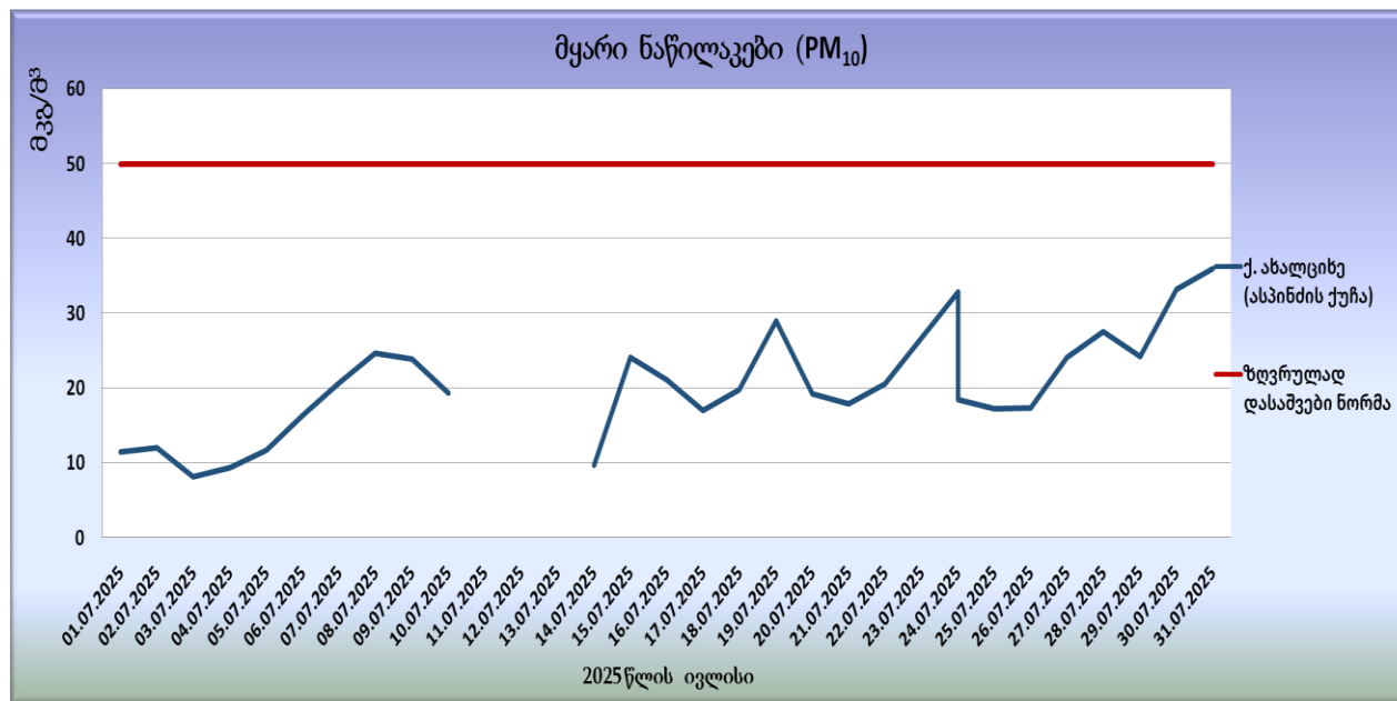
გრაფიკი N20. მყარი ნაწილაკების (PM 10 ) საშუალო დღეისო კონცენტრაციები
