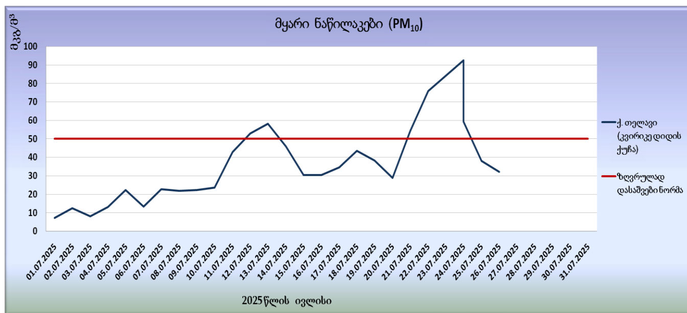
გრფიკი N29. მყარი ნაწილაკების (PM 10 ) საშუალოდღეობის კონცენტრაციები
