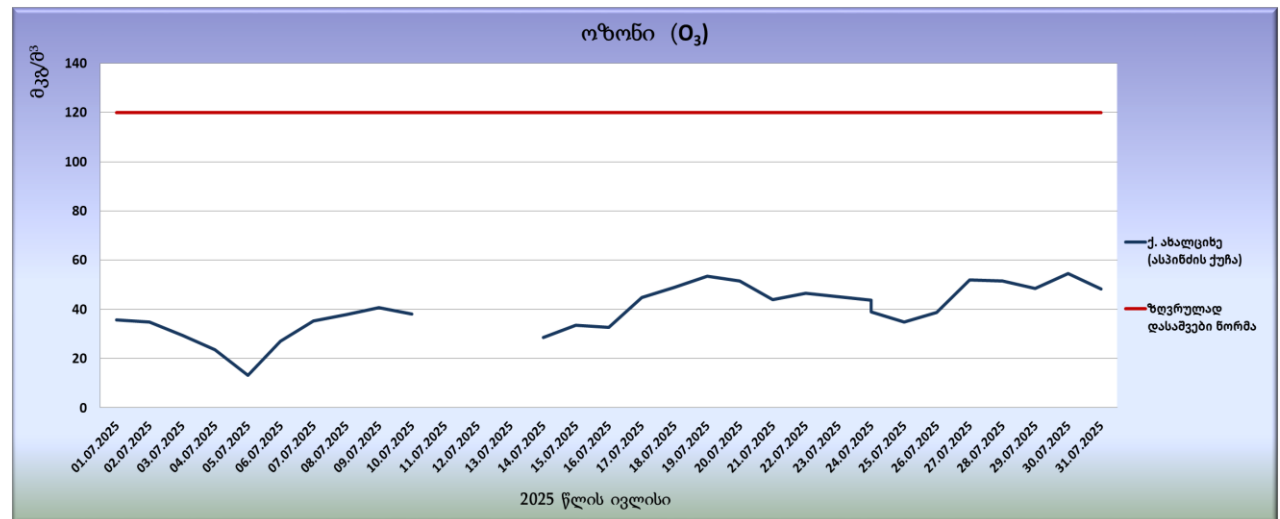
გრაფიკი N21. ოზონის ( O_3 ) ყოველდღიური რეგისტრირებული მაქსიმალური საშუალო კონცენტრაციები
