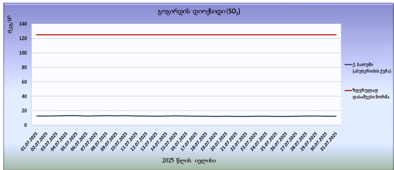
გრფიკი N6. გოგირდის დიოქსიდის ( \text{SO}_2 ) საშუალო დღეობის კონცენტრაციები
