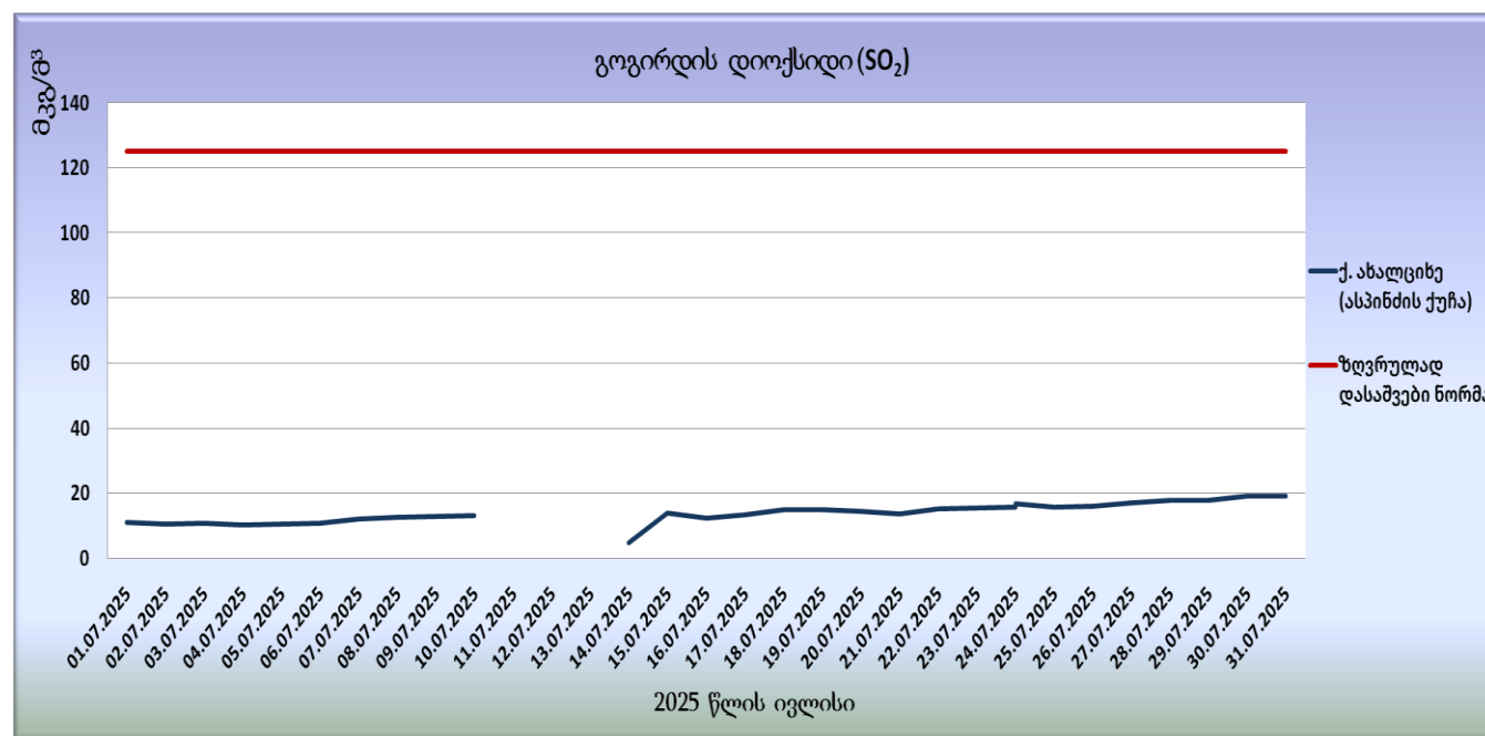
გრფუკი N19. გოგირდის დიოქსიდის (SO 2 ) საშუალო დღეობრივი კონცენტრაციები
