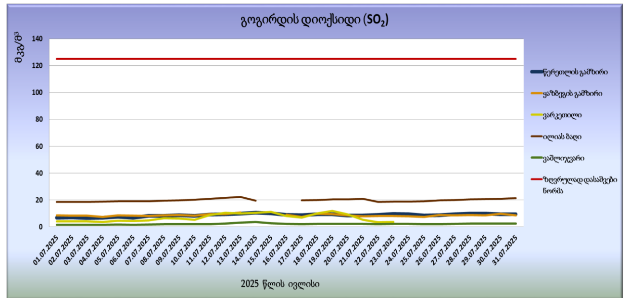
გრფიკი N1. გოგირდის დიოქსიდის (SO 2 ) საშუალო სადღლამისოკონცენტრაციები
