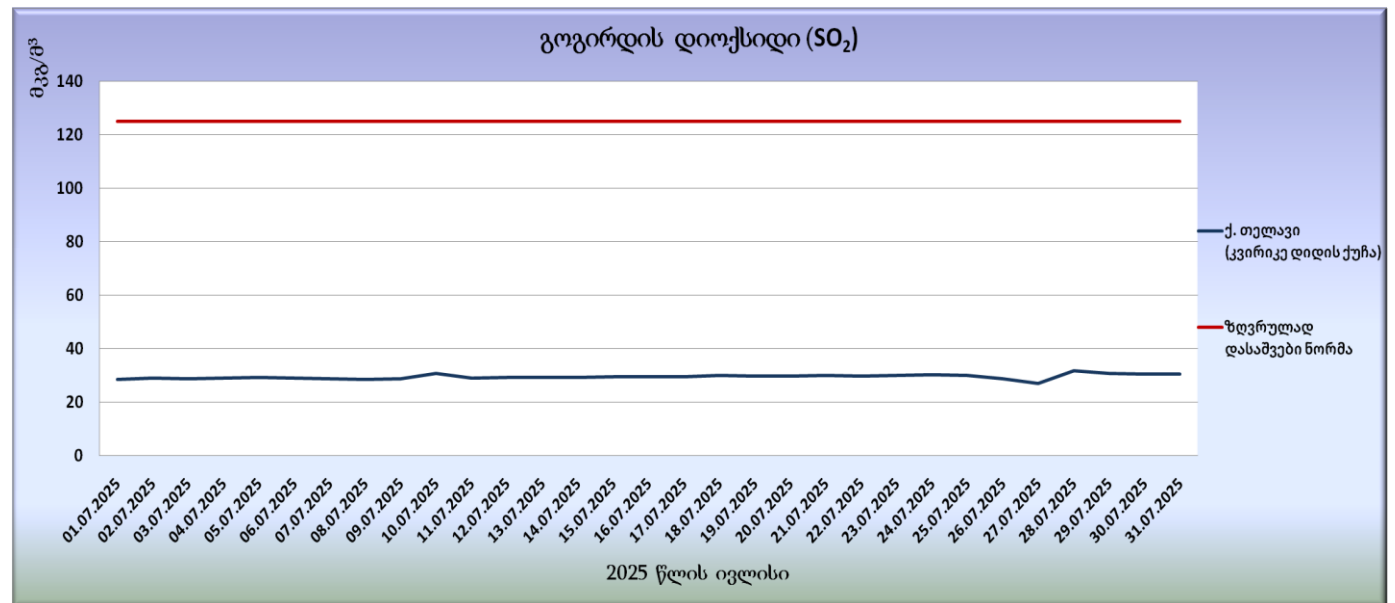
გრფიკი N28. გოგირდის დიოქსიდის (SO 2 ) საშუალო დღეობის კონცენტრაციები
