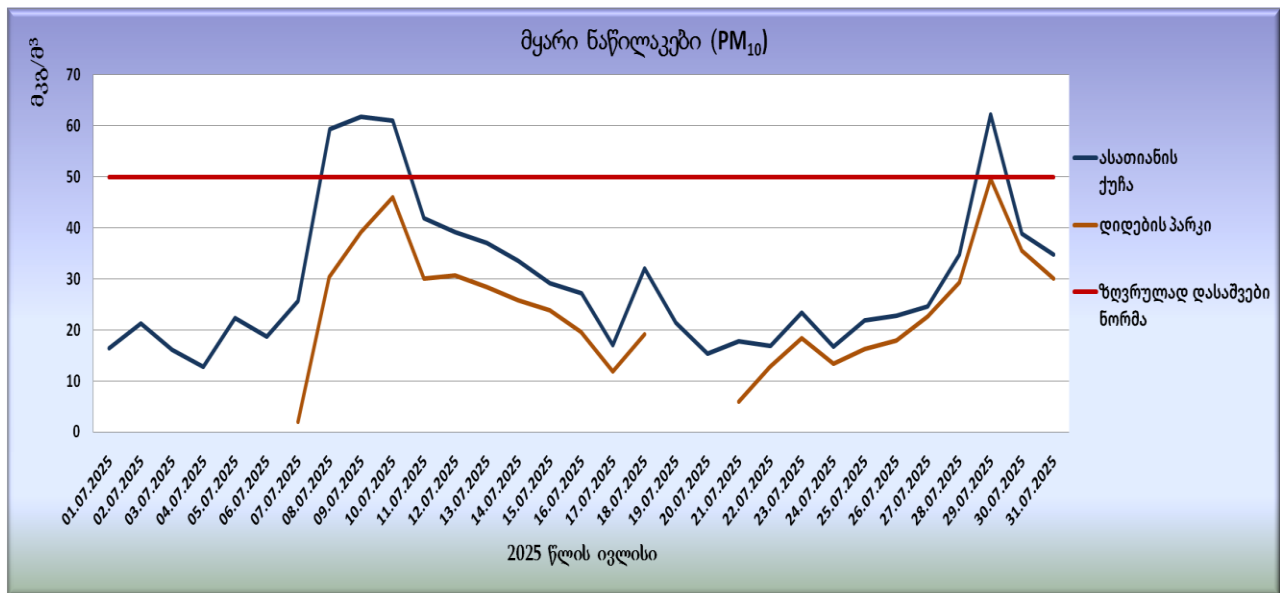
გრაფიკი N16. მყარი ნაწილაკების (PM 10 ) საშუალო სადღღმისოკონცენტრაციები
