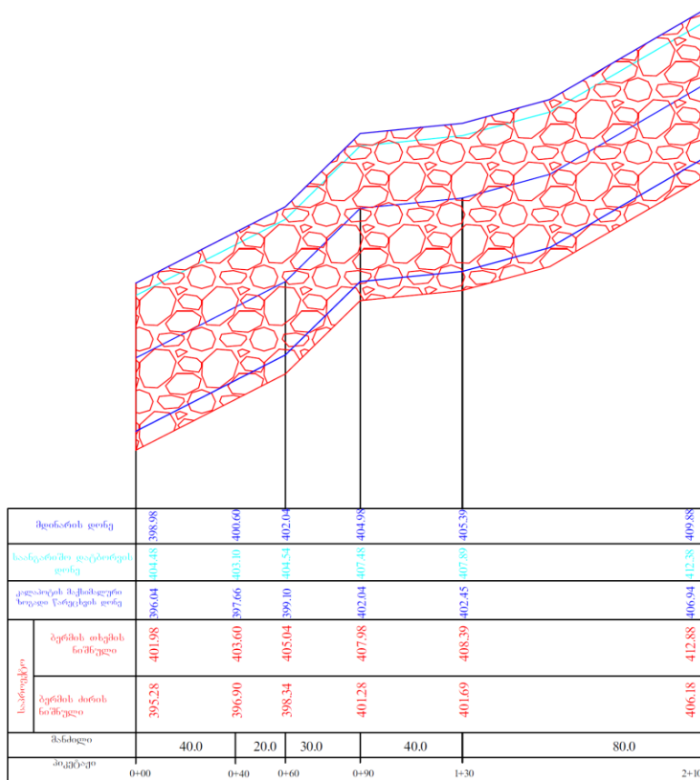
ნახაზი 4 ნაპირსამაგრი კედლის და სანაყროს ჭრილი
