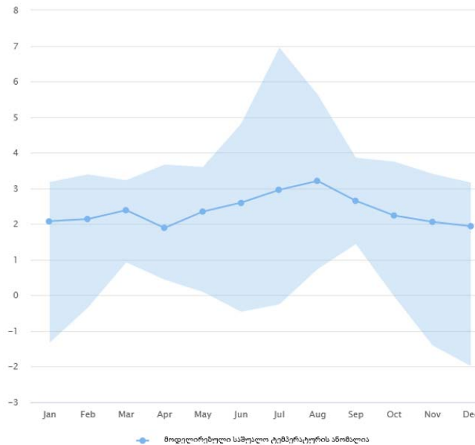
ნახაზი 10 - ტემპერატურის ცვლილების პროგნოზი 2040-2059 წლებისთვის RCP 8.5-ის პირობებში - გურიის რეგიონი
