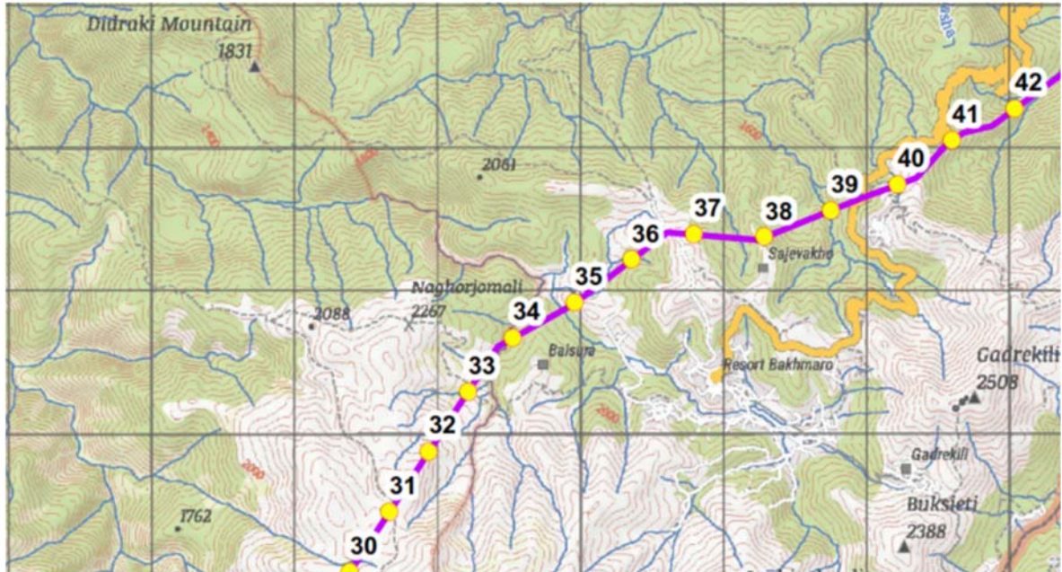
ნახაზი 7 - ოზურგეთი - ზოტი 110 კვ ხაზის მარშრუტი ბახმაროს მახლობლად
