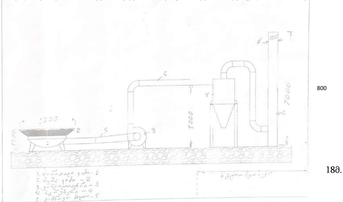
ნახაზზე 3.1.1. აგლომერაციის პროცესის ტექნოლოგიური სქემა
