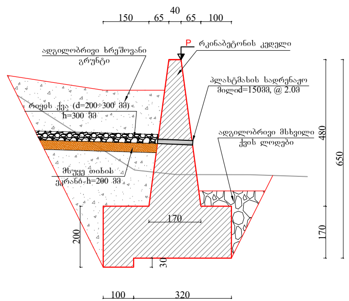
განვიკვეთი მ. 1:50
