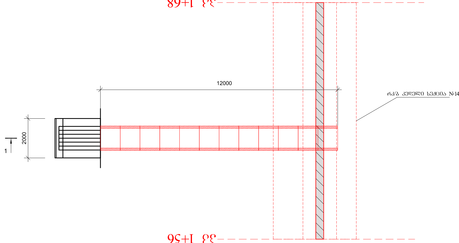
გეგმა მ 1:100
