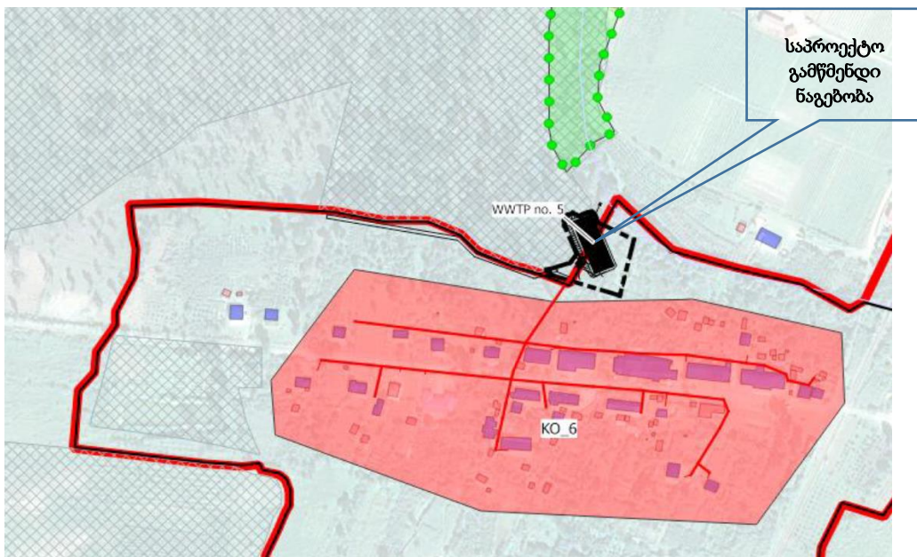
ნახაზი 4.2.5.1 საპროექტო საკანალიზაციო ქსელის არეალი (მონიშნულია ვარდისფრად)
