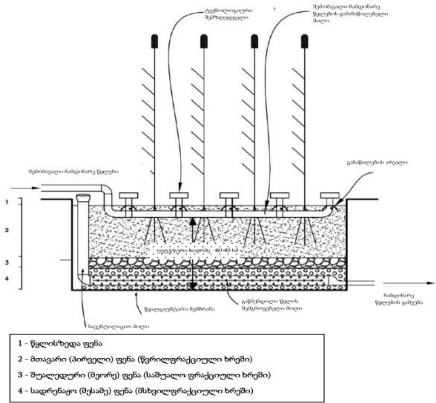
სურათი 4.2.2.1. ვერტიკალურ ნაკადიანი ჰიდრობოტანიკური მოედნის - . ე.წ. „აშენებული ჭაობების“ ტიპური სქემა
