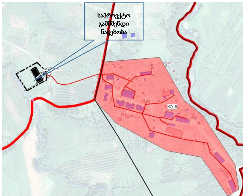
ნახაზი 4.2.5.1 საპროექტო საკანალიზაციო ქსელის არეალი (მონიშნულია ვარდისფრად)
